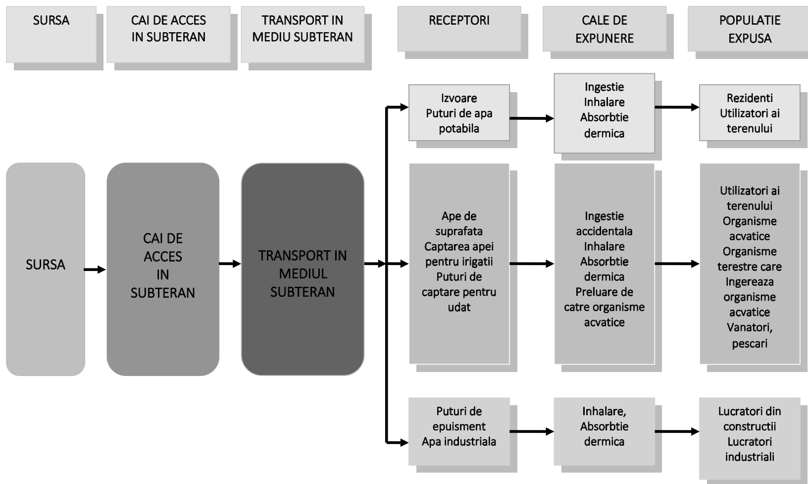
Figura 2 Diagrama cale-receptor
