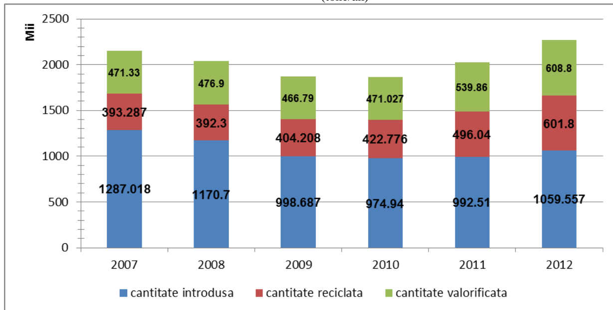
Graficul nr. IV.7.1.3.2.7. Cantități de ambalaje introduse pe piață la nivel național, deșeuri de ambalaje reciclate/valorificate (tone/an)
