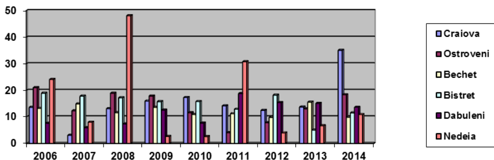
Graficul nr. IV.9.1.3.3. Evoluția multianuală a Cs-137 din probele de sol din zona de influență a CNE Kozlodui
