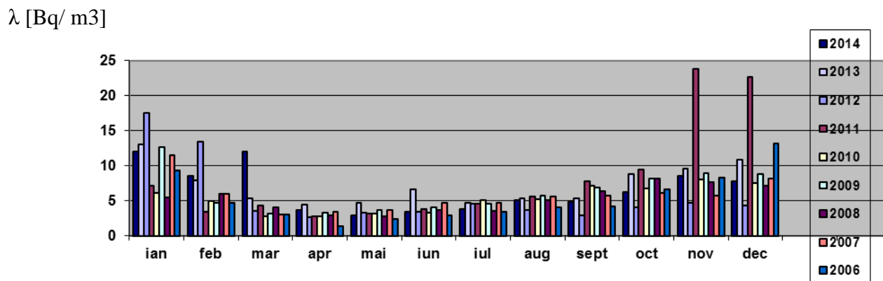
Graficul nr. IV.9.1.1.8. Evoluția multianuală și sezonieră a radioactivității descendenților radonului, între orele 9-14 în locația Bechet
