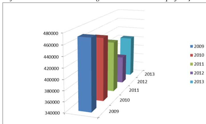
Graficul nr. IV.10.1.2.3. - Energia termica distribuită pe județul Dolj
