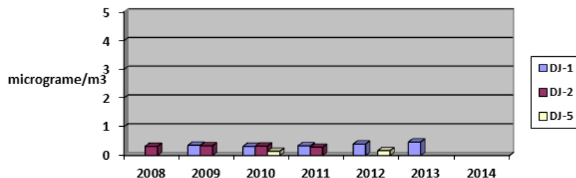
Graficul nr. IV.1.1.1.2.5. CO- Evoluția mediilor anuale în stațiile de monitorizare
