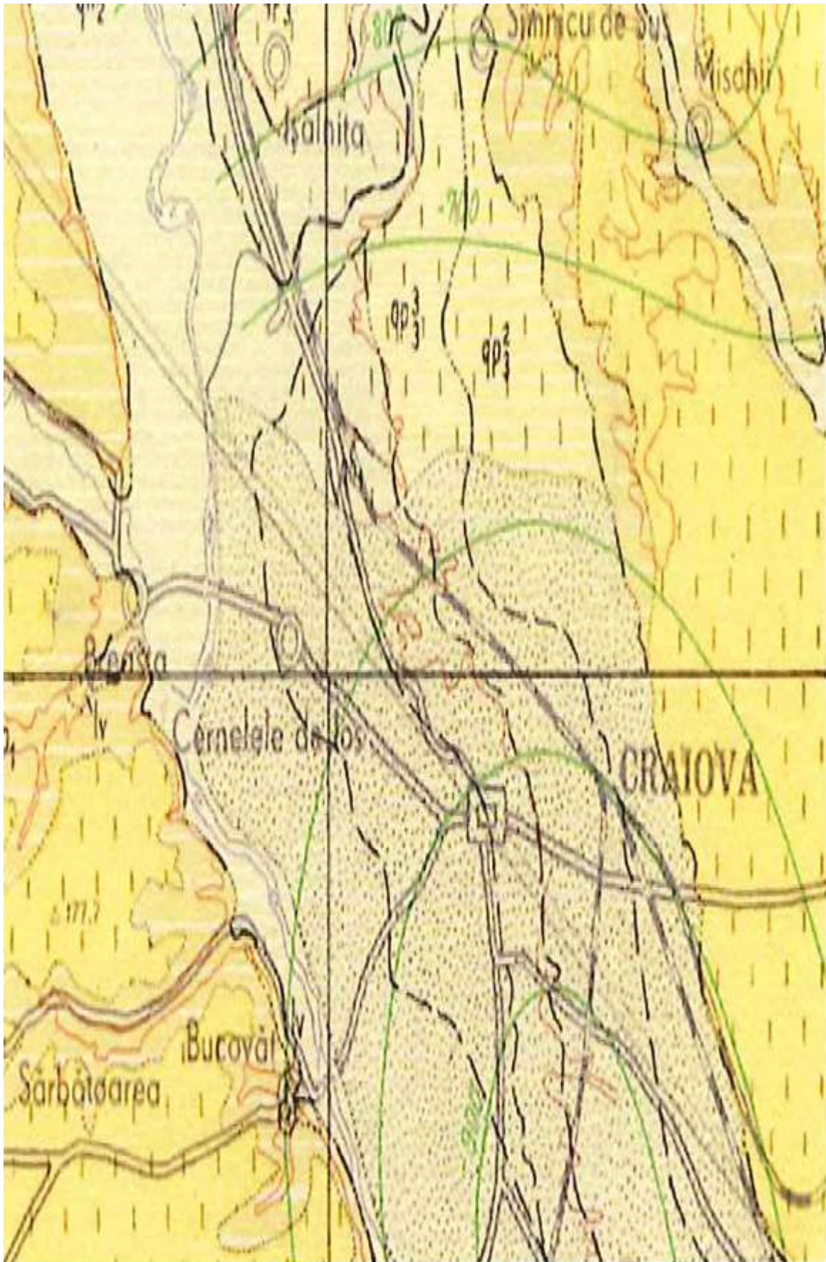
Harta geologică qp 2 3 - pietrișuri și nisipuri- Pleistocen superior
