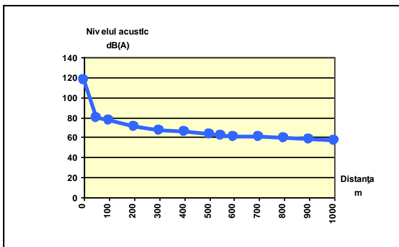
Fig. nr. 6. Variația teoretică a intensității zgomotului produs de utilajele balastierii în funcție de distanță
