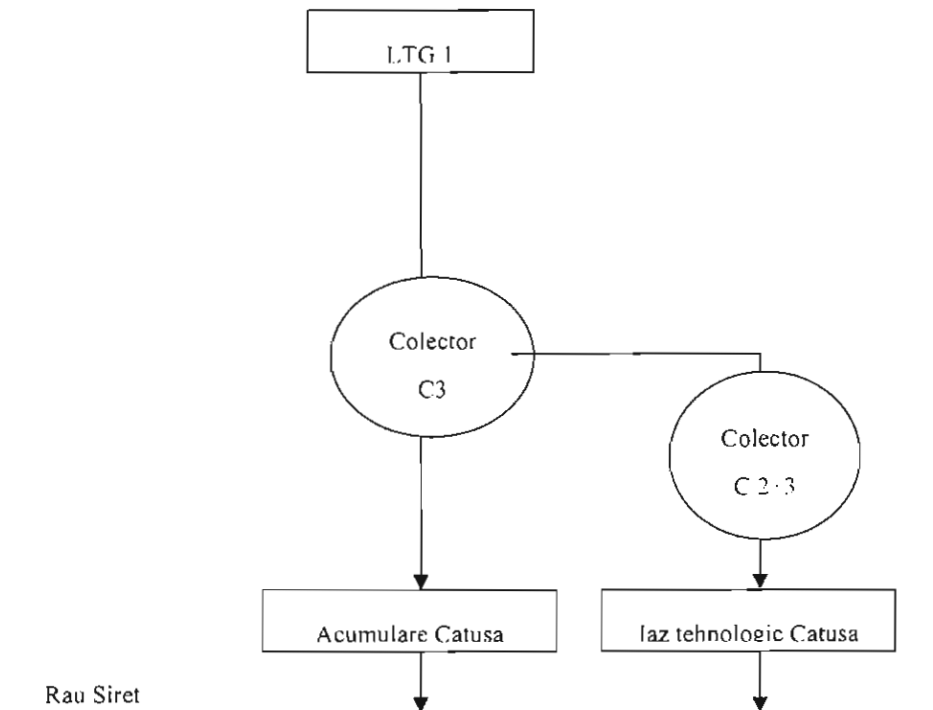
Schema de funcționare a colectoarelor de la LTG 1
