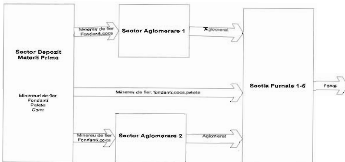
Diagrama proceselor tehnologice desfășurate pe amplasament
