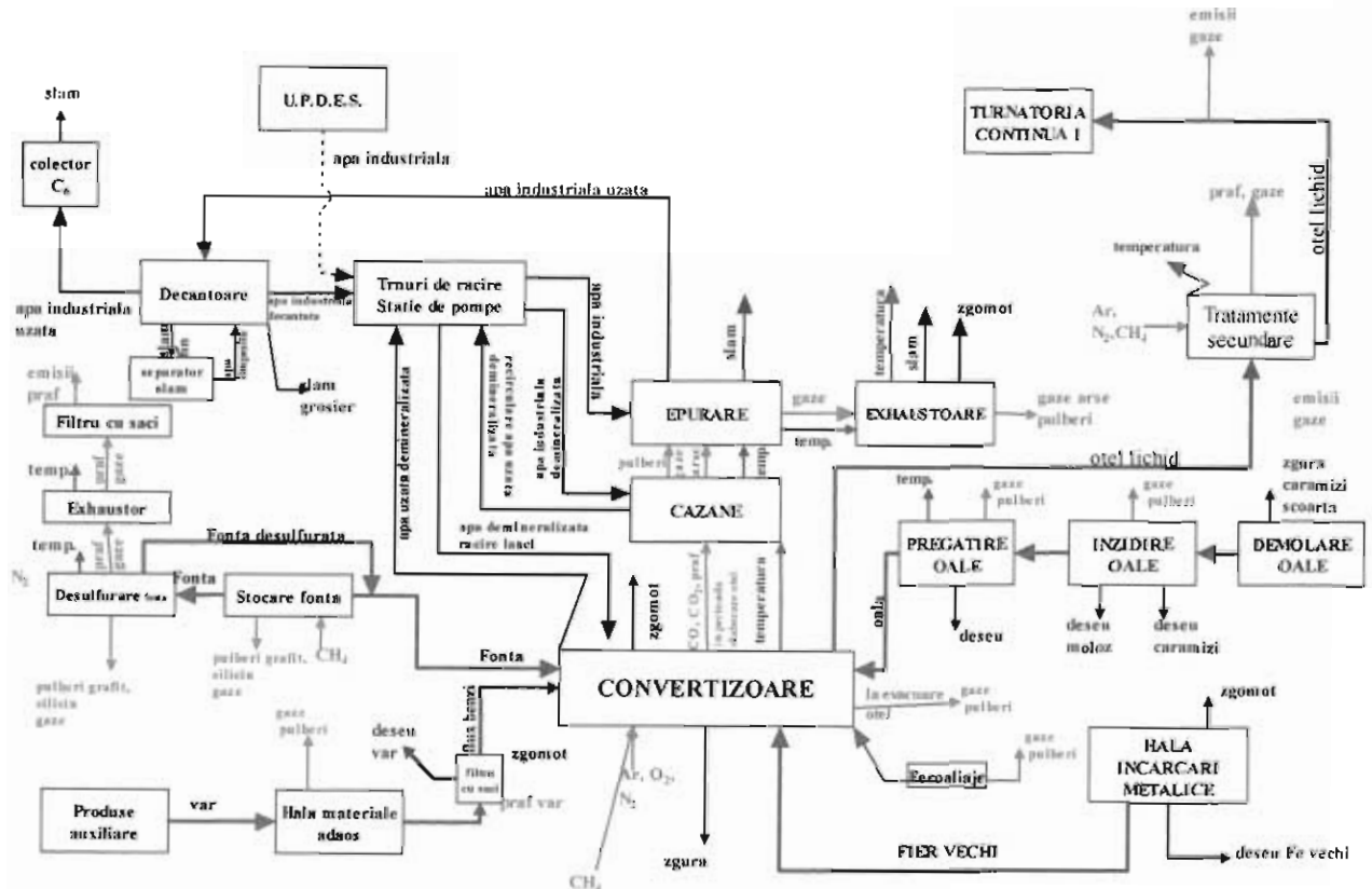
Diagrama proceselor tehnologice desfășurate pe amplasamentul Oțelăriei LD1
