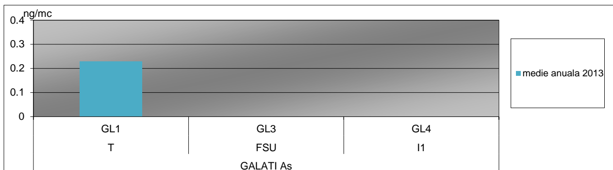
Fig. I.1.1.2.7. Evoluția arsenului, în perioada 2011 – 2016, \mu\text{g}/\text{mc}
