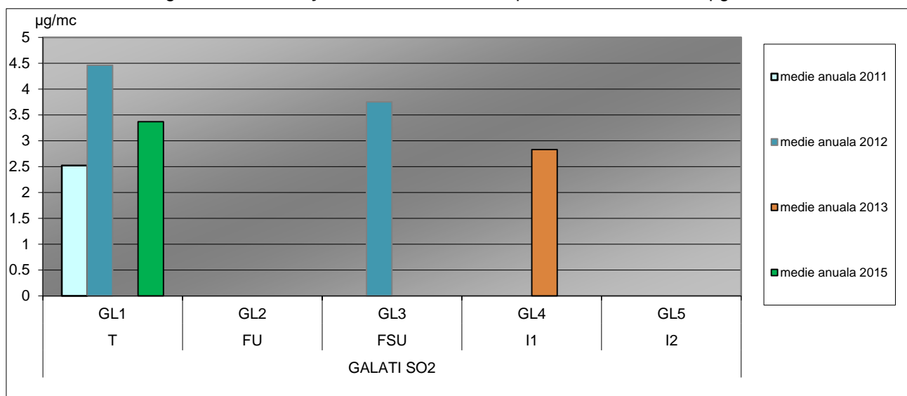
Fig. I.1.1.2.2. Evoluția dioxidului de sulf în perioada 2011 – 2016, \mu\text{g}/\text{m}^3
