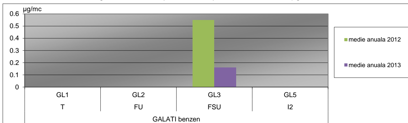
Fig. I.1.1.2.9. Evoluția benzen în perioada 2011 - 2016, \mu\text{g}/\text{mc}
