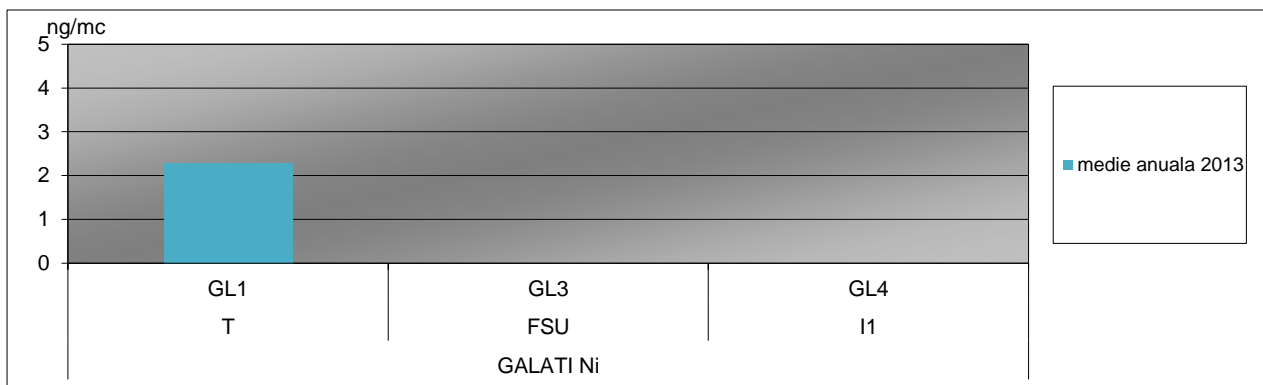
Fig. I.1.1.2.6. Evoluția nichel, în perioada 2011 – 2016, \mu\text{g}/\text{mc}
