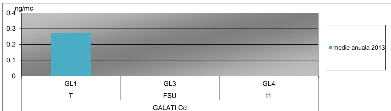
Fig. I.1.1.2.5. Evoluția cadmiului, în perioada 2011 – 2016, \mu\text{g}/\text{mc}
