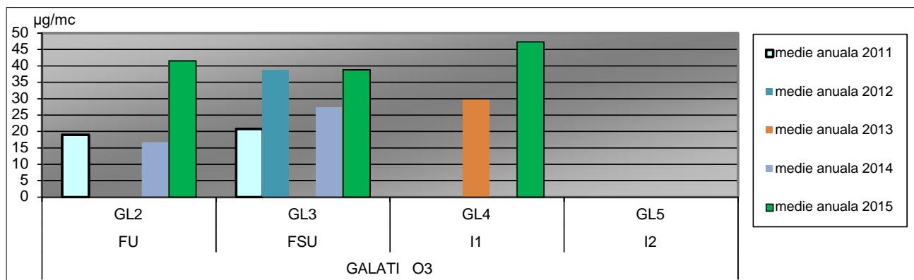
Fig. I.1.1.2.10. Evoluția ozonului în perioada 2011 - 2016, \mu\text{g}/\text{mc}
