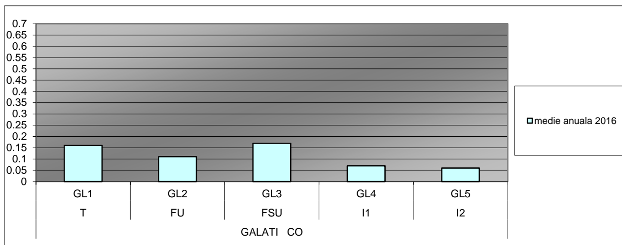
Fig. I.1.1.1.5. Concentrații medii anuale ale monoxidului de carbon în anul 2016, mg/mc
