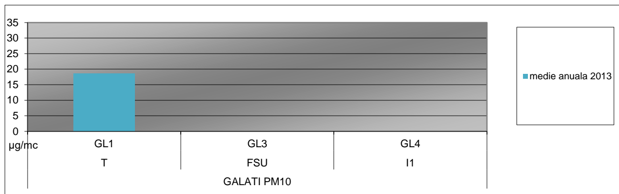
Fig. I.1.1.2.3. Evoluția pulberilor în suspensie, fracțiunea PM10 gravimetric în perioada 2011 – 2016 ( \mu\text{g}/\text{mc} )
