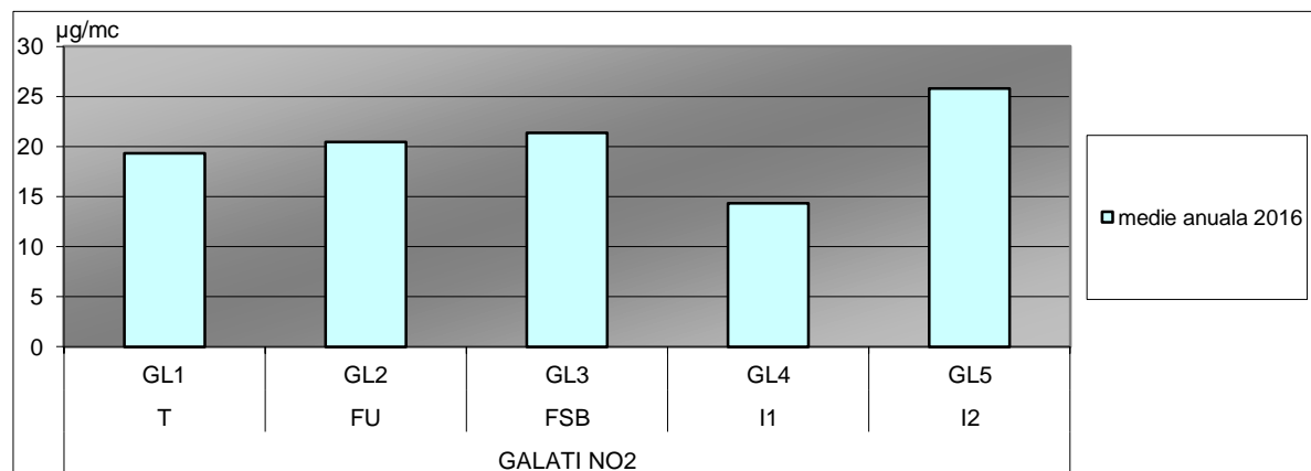
Fig. I.1.1.1.1. Concentrații medii anuale ale dioxidului de azot în anul 2016
