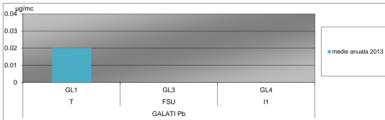
Fig. I.1.1.2.4. Evoluția plumbului, în perioada 2011 – 2016, \mu\text{g}/\text{mc}
