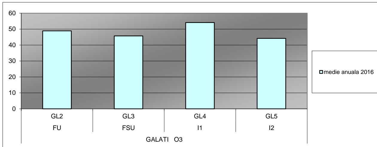
Fig. I.1.1.1.7. Concentrații medii anuale de O 3 în anul 2016, µg/mc
