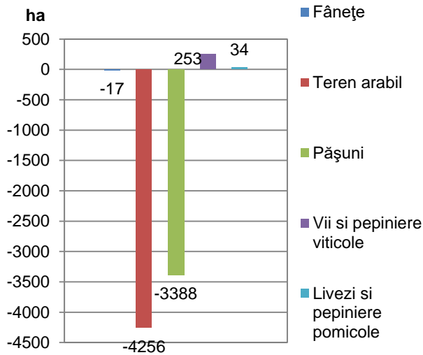
Fig. IV.1.2.1. Schimbări în acoperirea/utilizarea terenurilor, în perioada 2010-2016 (ha)
