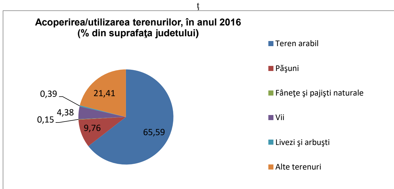
Figura IV.1.1.1. - Acoperirea/utilizarea terenurilor, în anul 2016 (% din suprafața totală a județului Galați)
