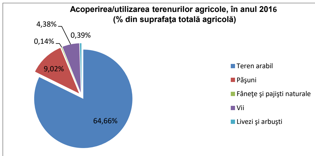
Figura IV.1.1.2. - Acoperirea/utilizarea terenurilor agricole, în anul 2016 (% din suprafața totală agricolă)
