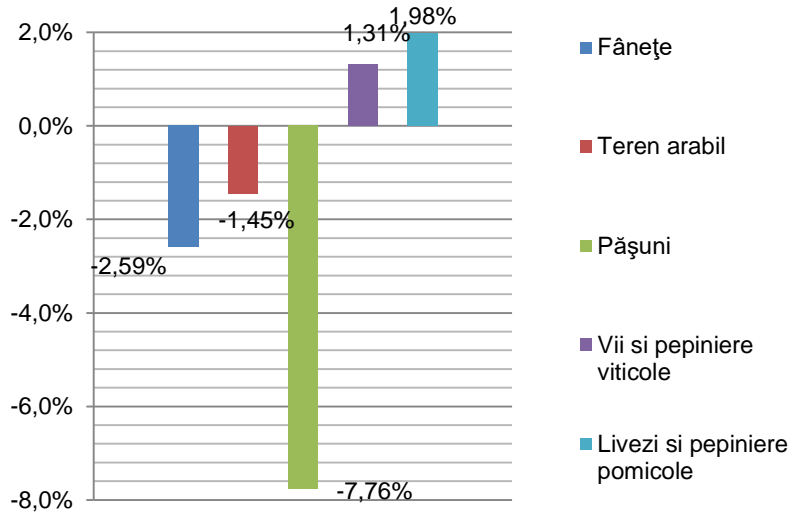
Fig. IV.1.2.2. Schimbări în acoperirea/utilizarea terenurilor, în perioada 2010-2016 (% din anul 2010)
