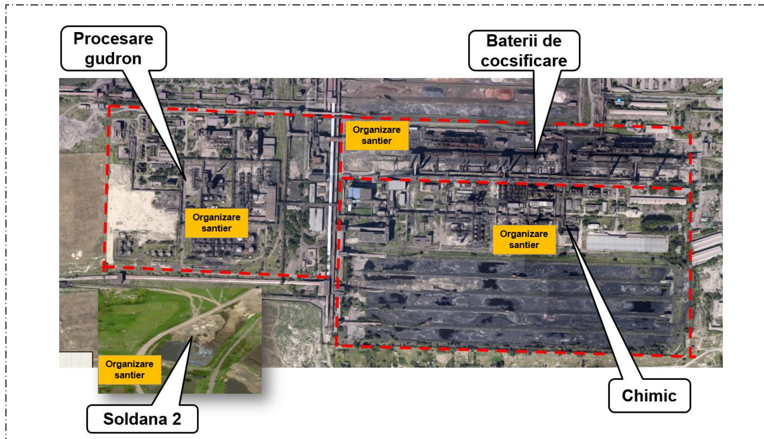
Plan organizării de șantier
