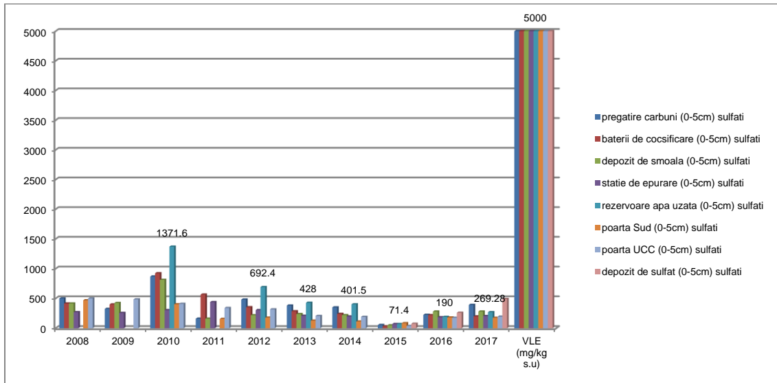
Valorile concentrației ionului Sulfați în orizonturile de sol cuprinse între 0 ÷ 5 cm, în perioada 2008 ÷ 2017
