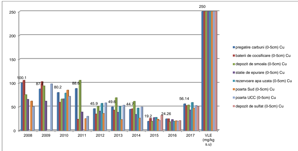
Valorile concentrației Cupru în orizonturile de sol cuprinse între 0 ÷ 5 cm, în perioada 2008 ÷ 2017
