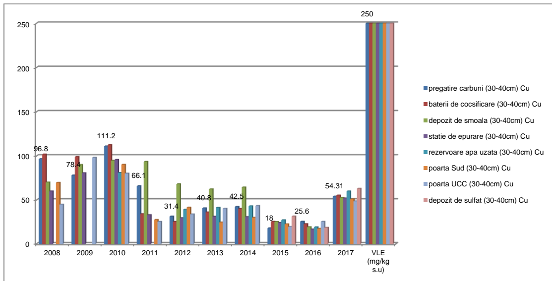
Valorile concentrației Cupru în orizonturile de sol cuprinse între 30 ÷ 40 cm, în perioada 2008 ÷ 2017 Analizând valorile obținute și comparând cu valorile de referință pentru urme de elemente
