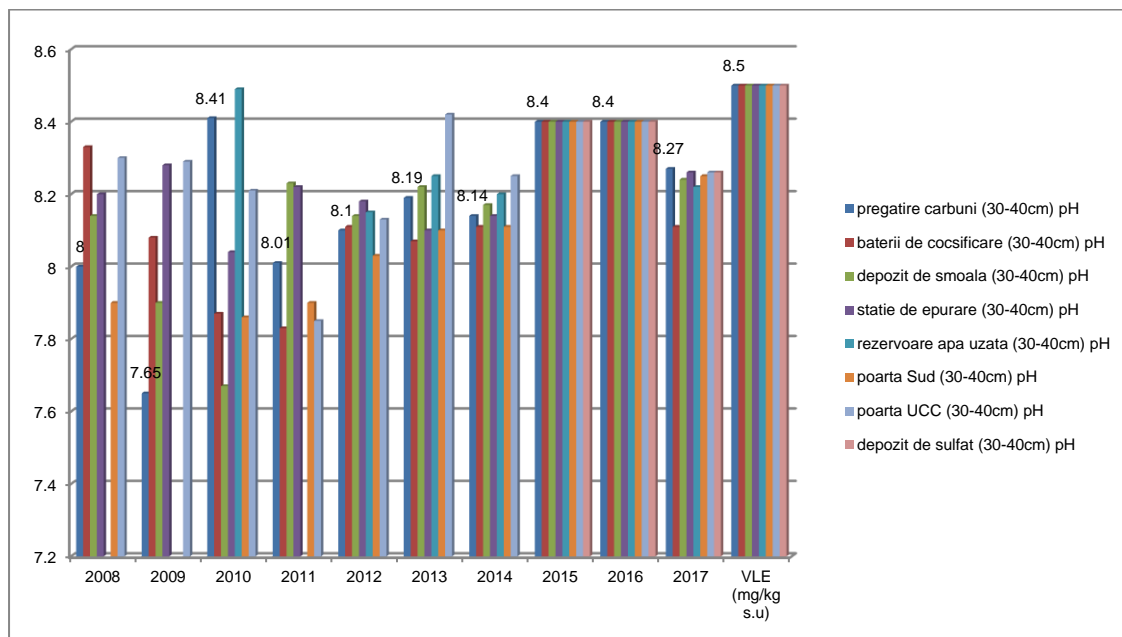
Variația pH-ului în zona UCC1, în orizonturile de sol cuprinse între 30 ÷ 40 cm, în perioada 2008 ÷ 2017
