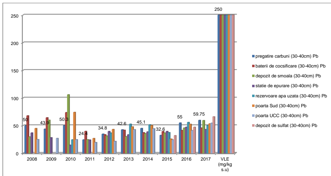
Valorile concentrației Plumb în orizonturile de sol cuprinse între 30 ÷ 40 cm, în perioada 2008 ÷ 2017
