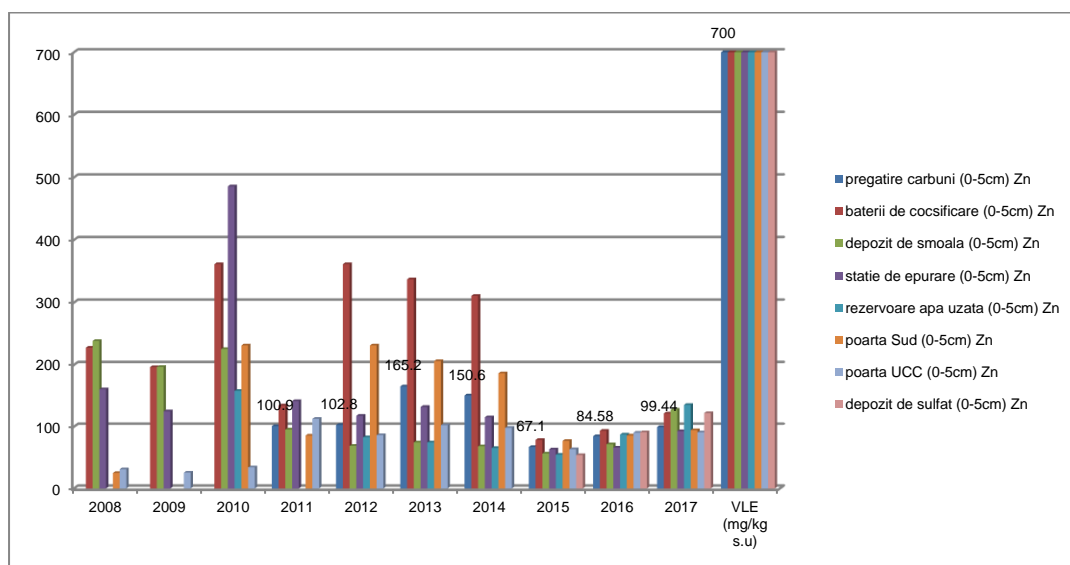
Valorile concentrației Zinc în orizonturile de sol cuprinse între 0 ÷ 5 cm, în perioada 2008 ÷ 2017 Analizând valorile obținute și comparând cu valorile de referință pentru urme de elemente
