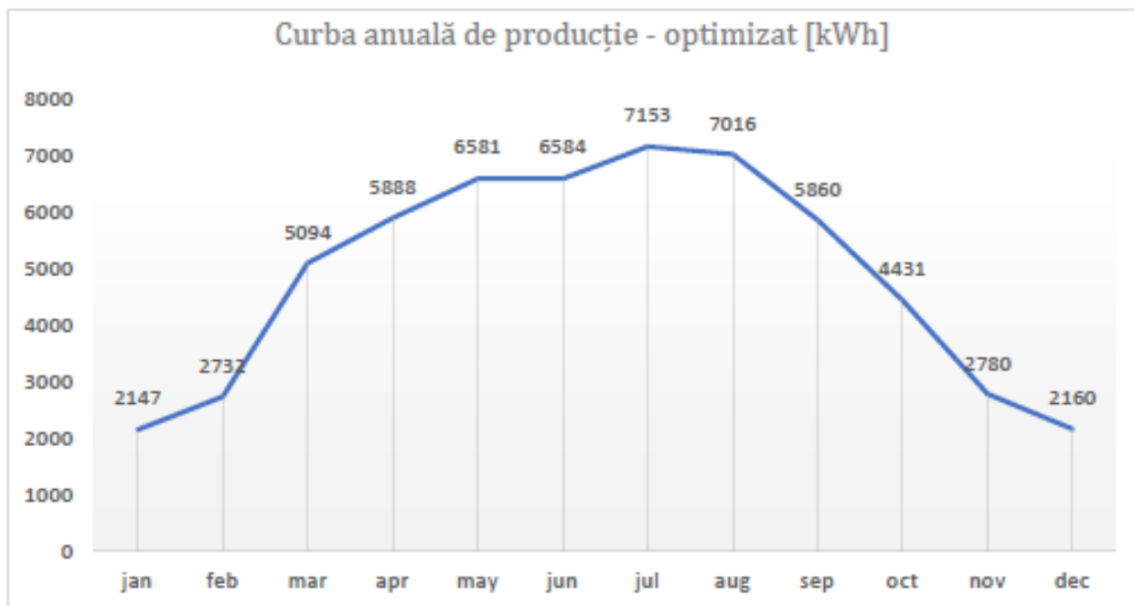
Figura 11 Curba anuală de producție – optimizat
