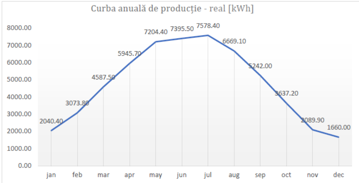
Figura 12 Curba anuală de producție - real
