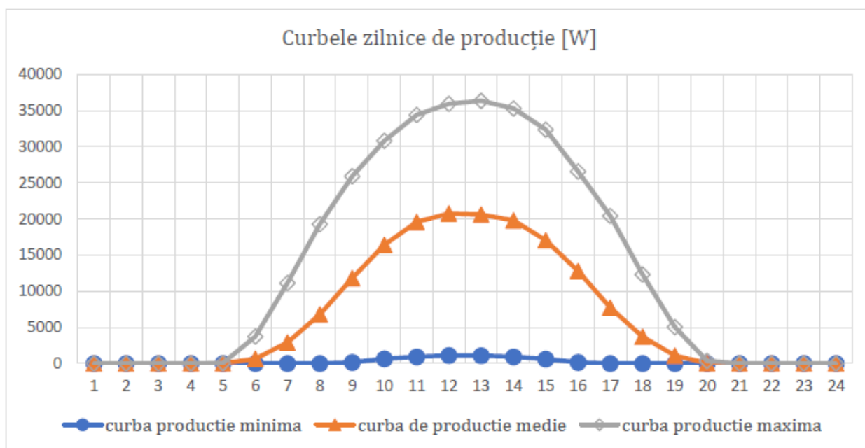
Figura 9 Curbele zilnice de producție
