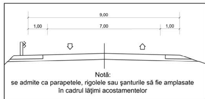
DRUM VICINAL CU 2 BENZI DE CIRCULAȚIE (M. Of. nr. 138 bis/6.IV.1998)
