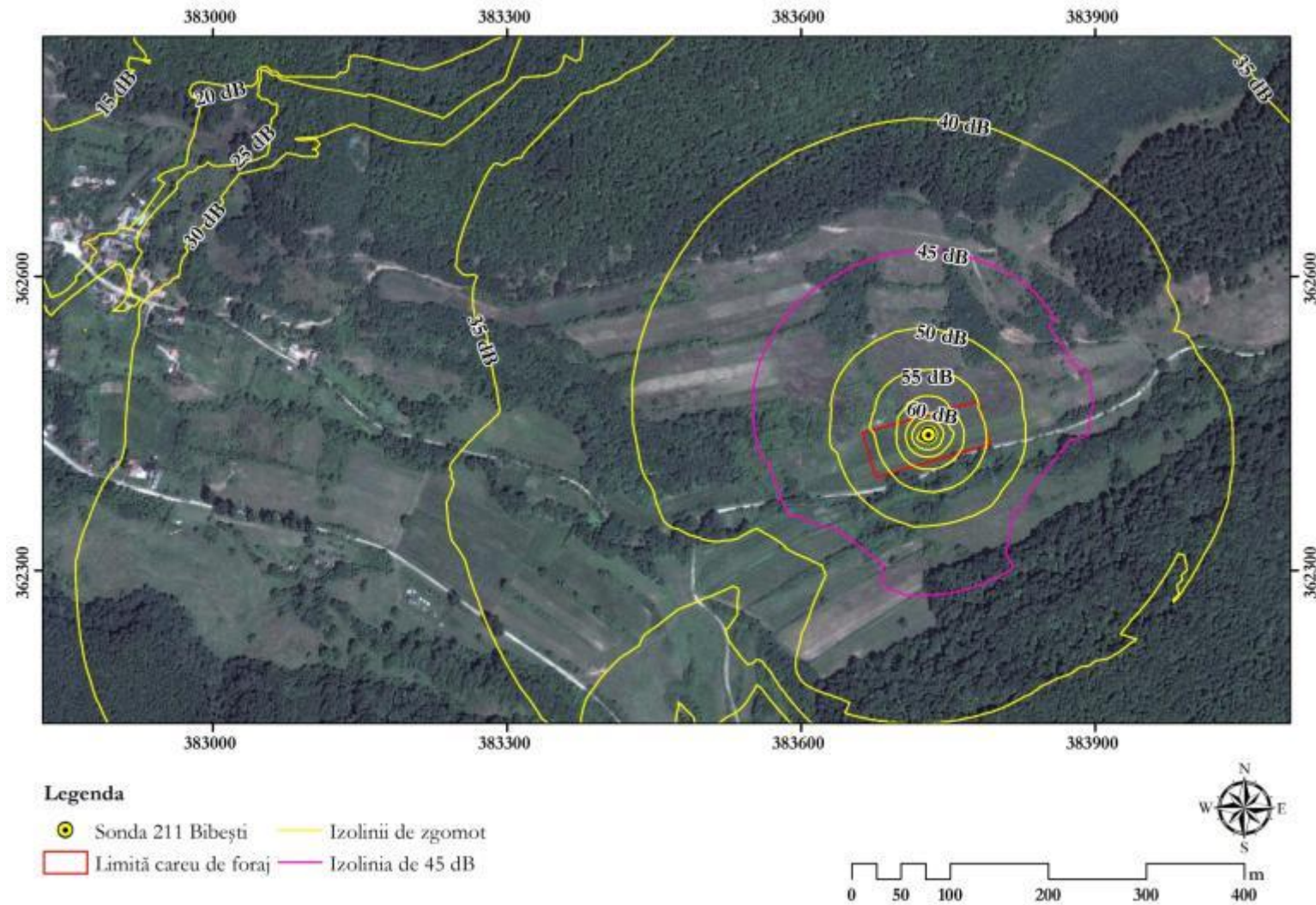
Figura nr. 1-8 Reprezentarea grafică a rezultatelor modelării surselor de zgomot în faza de execuție a proiectului
