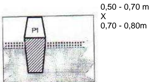
Fig. 3. Model de borna inscriptiata pentru materializarea in teren a profilelor etalon pentru masuratori topo ante si post executie
