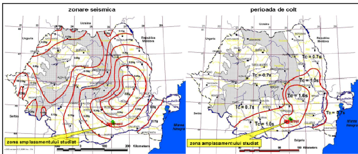
Fig. 17. Harta seismică
