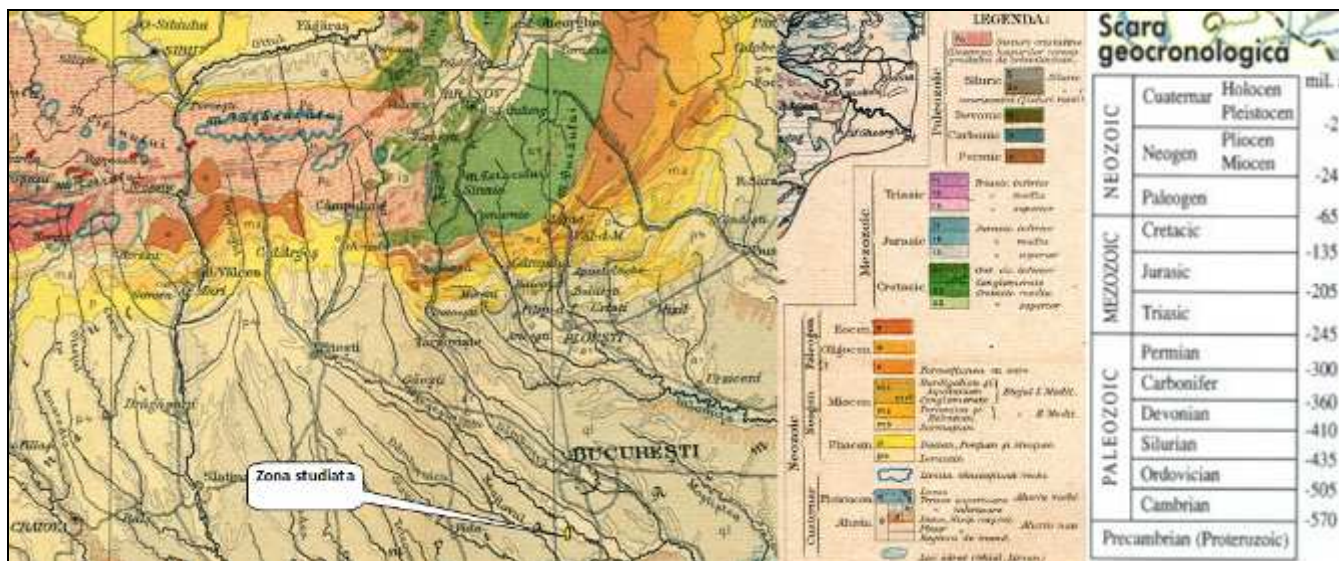
Fig. 16. Harta geologie
