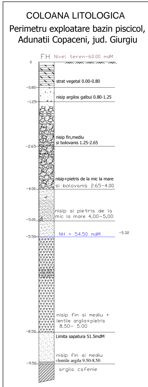
Fig. 7. Coloana litologica
