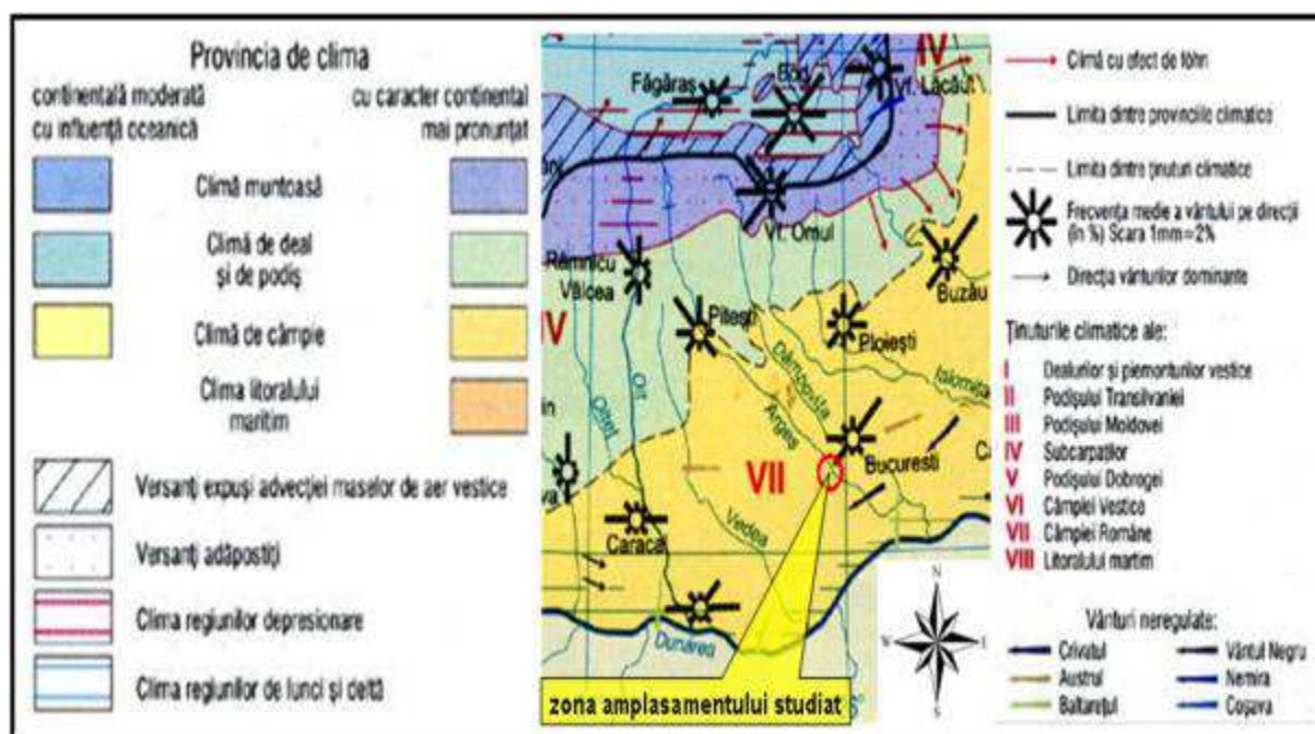
Fig. 11. Harta clima
