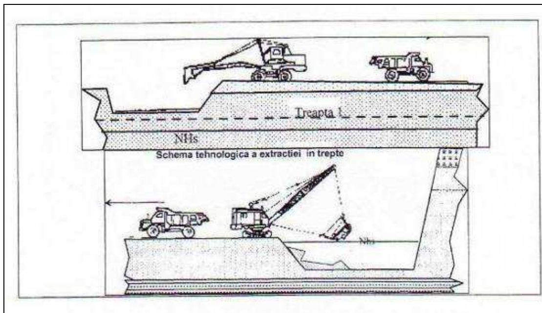
Fig 4. Schema tehnologica a extractiei in trepte
