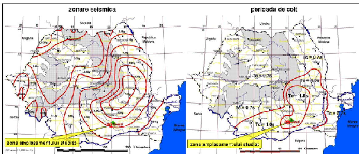
Fig. 17. Harta seismica
