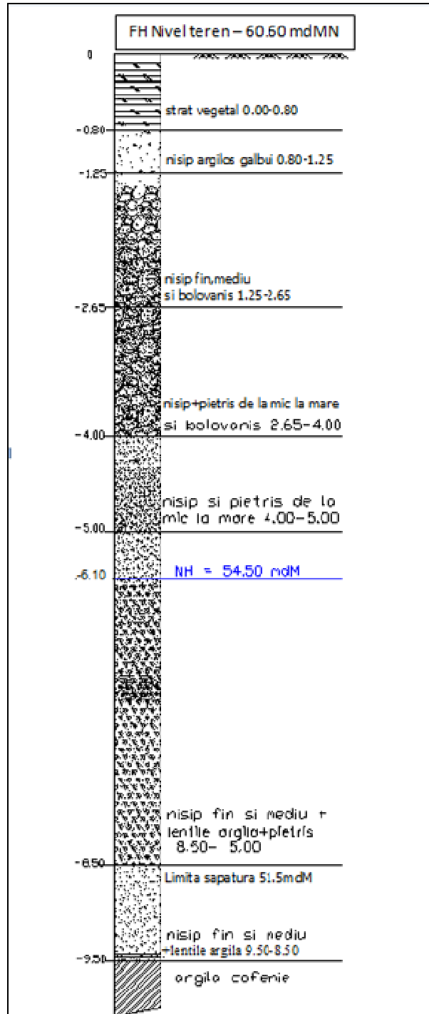
Fig. 7. Coloana litologica
