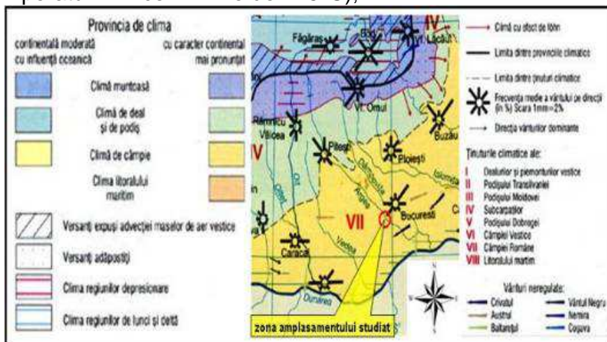
Fig. 11. Harta clima
