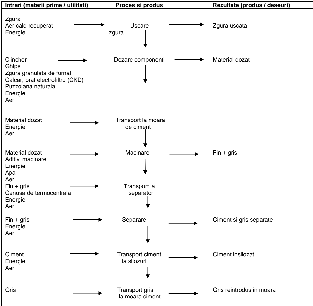
Diagrama de proces tehnologic pentru producerea cimentului
