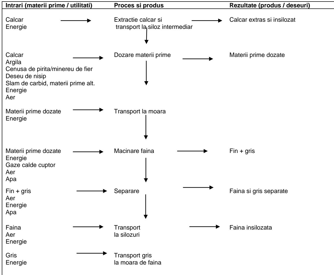
Diagrama de proces tehnologic pentru producerea fainii
