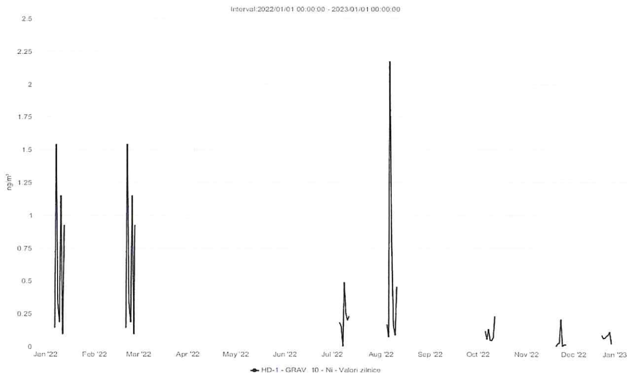
Figura nr. 2.4.3. Evoluția valorilor zilnice de Ni (ng/mc) din PM 10 gravimetric, pe parcursul a 8 săptămâni distribuite uniform pe toată durata anului 2022, la stația automată de monitorizare HD-1 din județul Hunedoara
