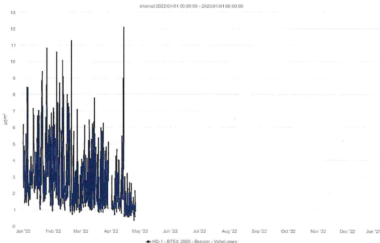
Figura nr. 2.6.1. Evoluția valorilor de benzen ( \mu\text{g}/\text{mc} ) în anul 2022 la stația automată de monitorizare HD-1, Deva, str. Carpați
