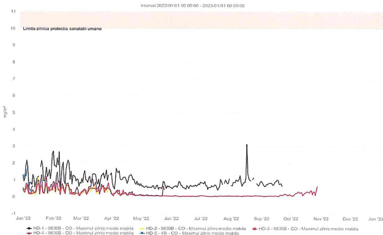
Figura nr. 2.5.1. Evoluția valorilor maxime zilnice a mediilor pe 8h de CO (mg/mc) în anul 2022 la stațiile automate de monitorizare din județul Hunedoara
