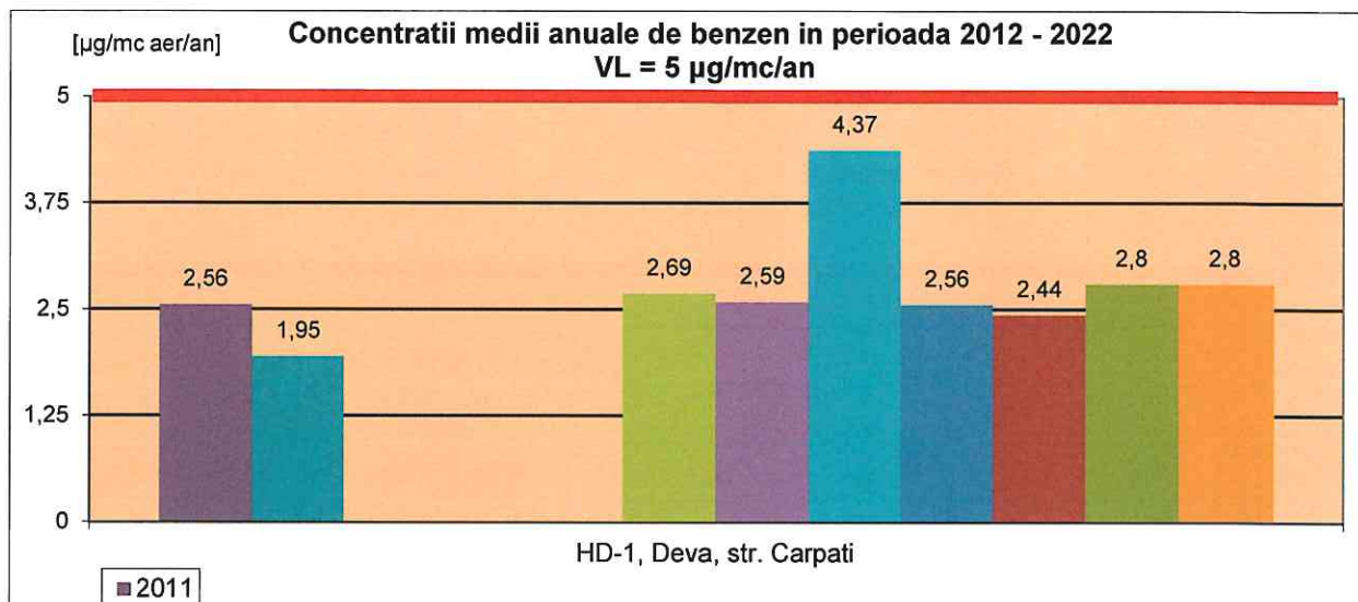
Figura nr. 2.8.6. Evoluția concentrațiilor medii anuale a benzenului, obținută prin rețeaua automată de monitorizare a calității aerului din județul Hunedoara în perioada 2012 – 2022
