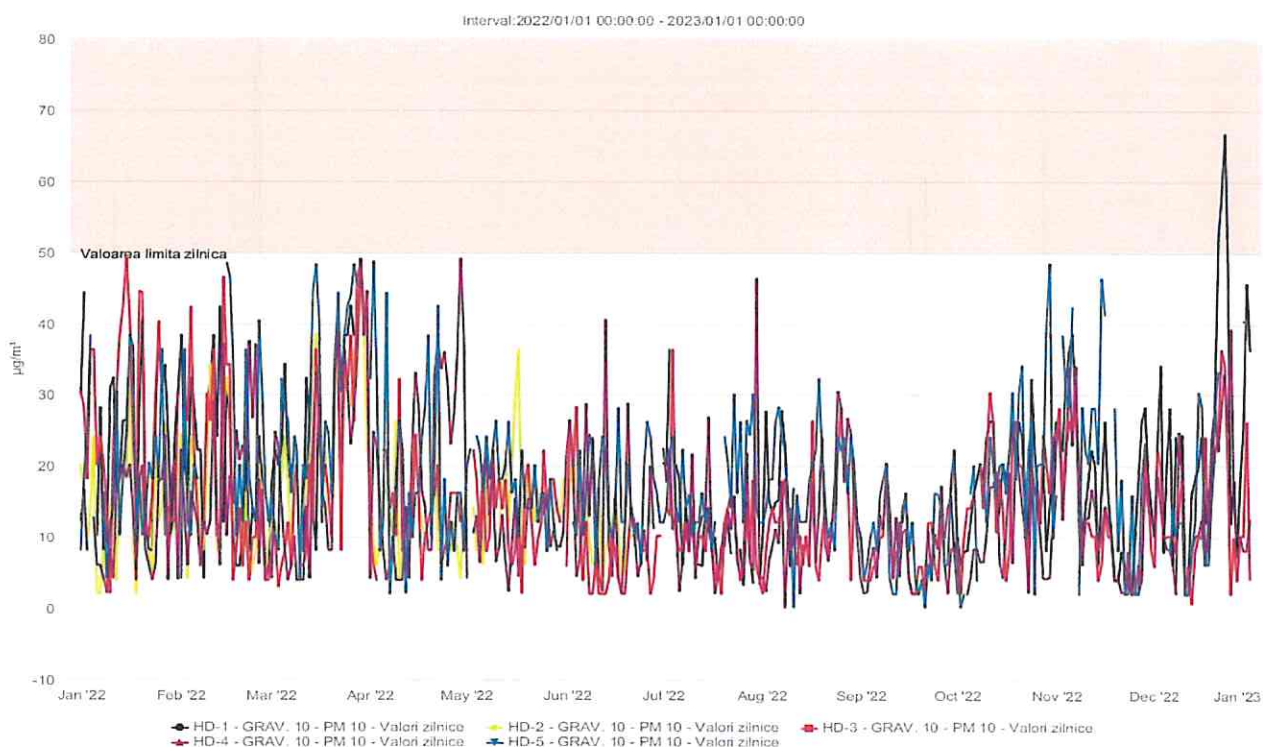
Figura nr. 2.3.2. Evoluția zilnică a valorilor de PM_{10} ( \mu\text{g}/\text{mc} ) determinat gravimetric în anul 2022 la stațiile automate de monitorizare din județul Hunedoara
