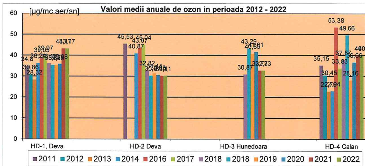
Figura nr. 2.8.7. Evoluția valorilor medii anuale ale ozonului, obținute prin rețeaua automată de monitorizare a calității aerului din județul Hunedoara în perioada 2012 – 2022
