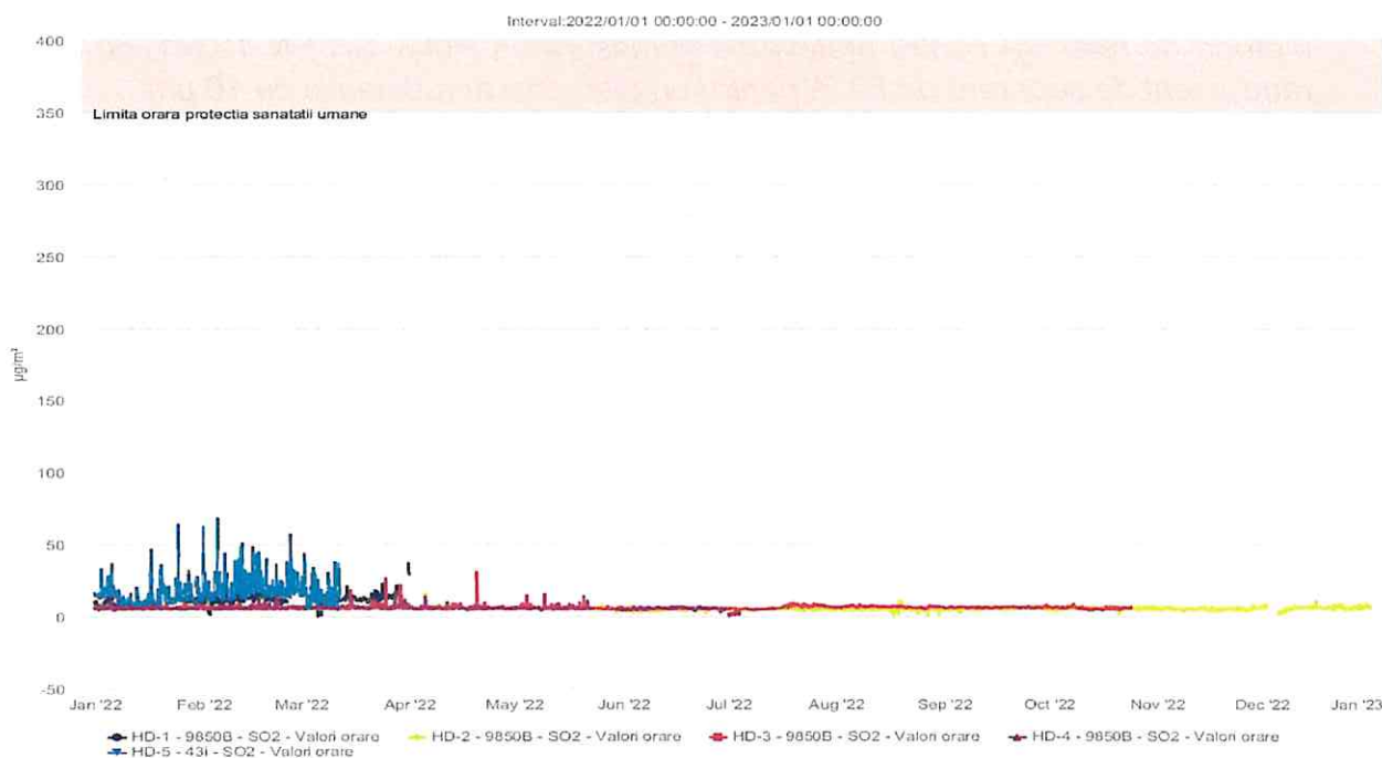
Figura nr. 2.2. 1. Evoluția valorilor orare de \text{SO}_2 ( \mu\text{g}/\text{mc} ) în anul 2022, la stațiile automate de monitorizare din județul Hunedoara
