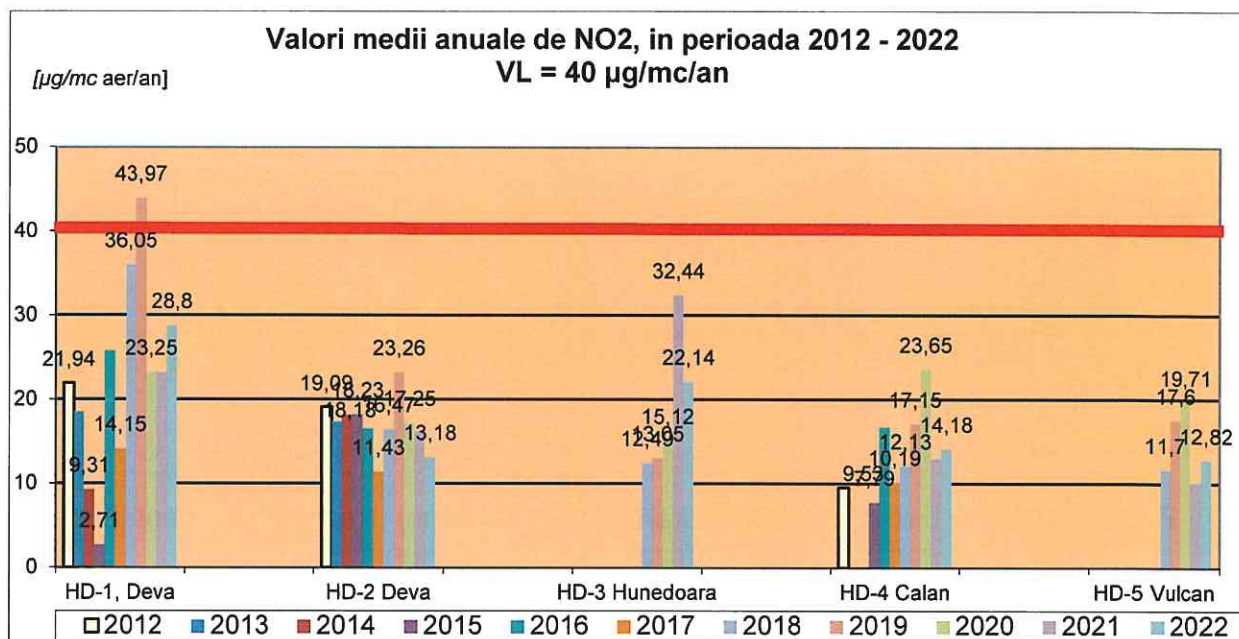
Figura nr. 2.8.1. Evoluția valorilor medii anuale de dioxid de azot obținute prin rețeaua automată de monitorizare a calității aerului din județul Hunedoara, în perioada 2012 – 2022
