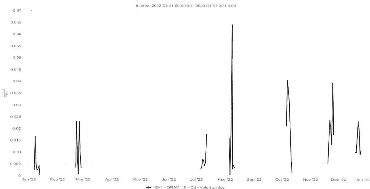
Figura nr. 2.4.2. Evoluția valorilor zilnice de Cd (ng/mc) din PM 10 gravimetric, pe parcursul a 8 săptămâni distribuite uniform pe toată durata anului 2022, la stația automată de monitorizare HD-1 din județul Hunedoara
