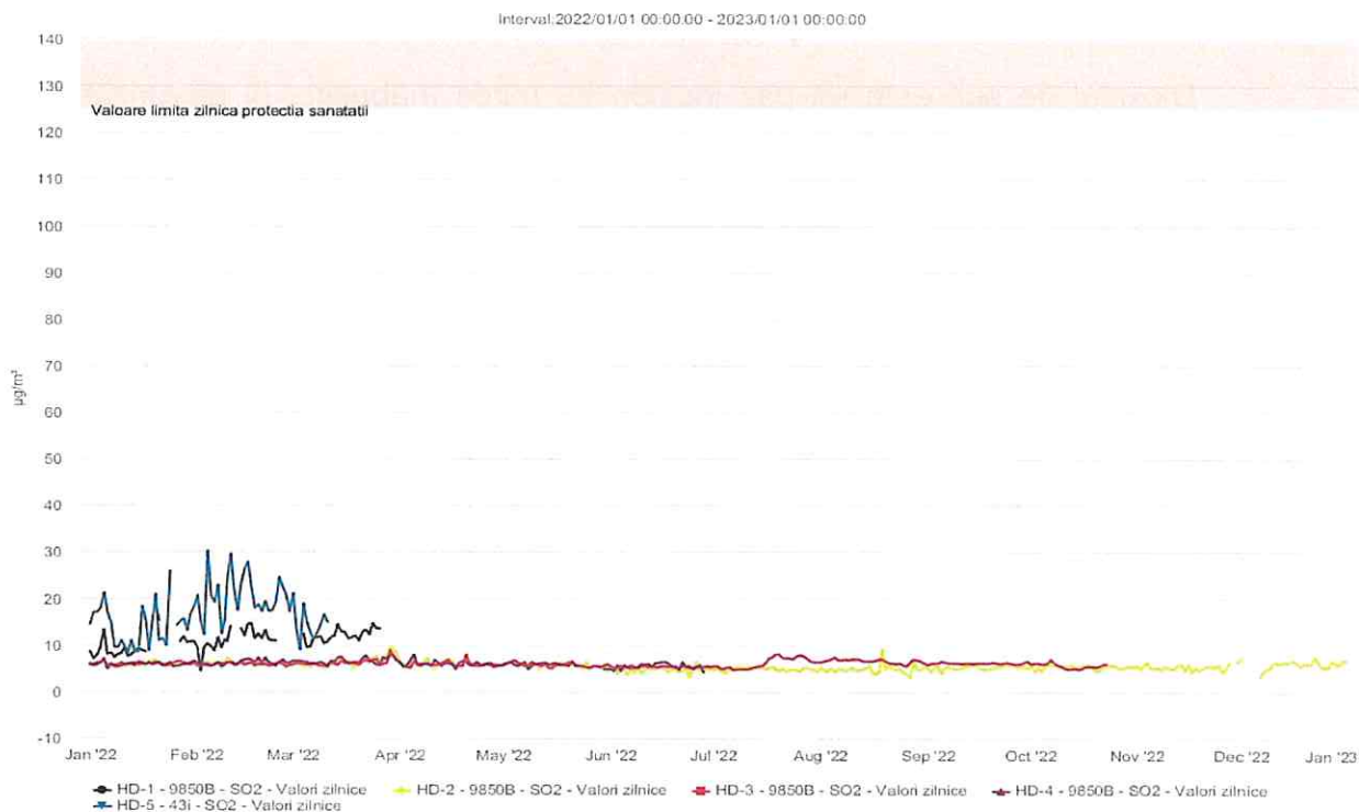
Figura nr. 2.2.2. Evoluția valorilor zilnice de SO 2 (µg/mc) în anul 2022 la stațiile automate de monitorizare din județul Hunedoara
