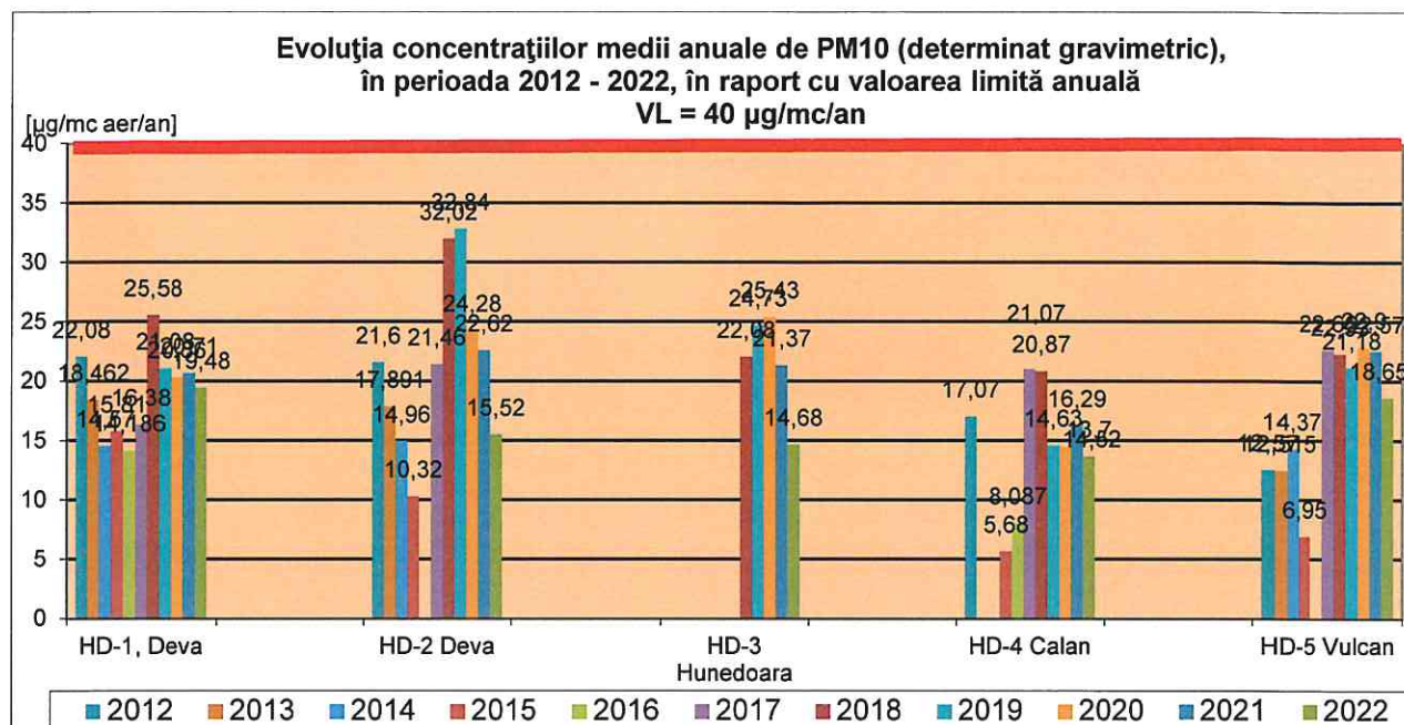
Figura nr. 2.8.3. Evoluția valorilor medii anuale ale PM 10 determinate gravimetric, obținute prin rețeaua automată de monitorizare a calității aerului din județul Hunedoara, în perioada 2012 – 2022
