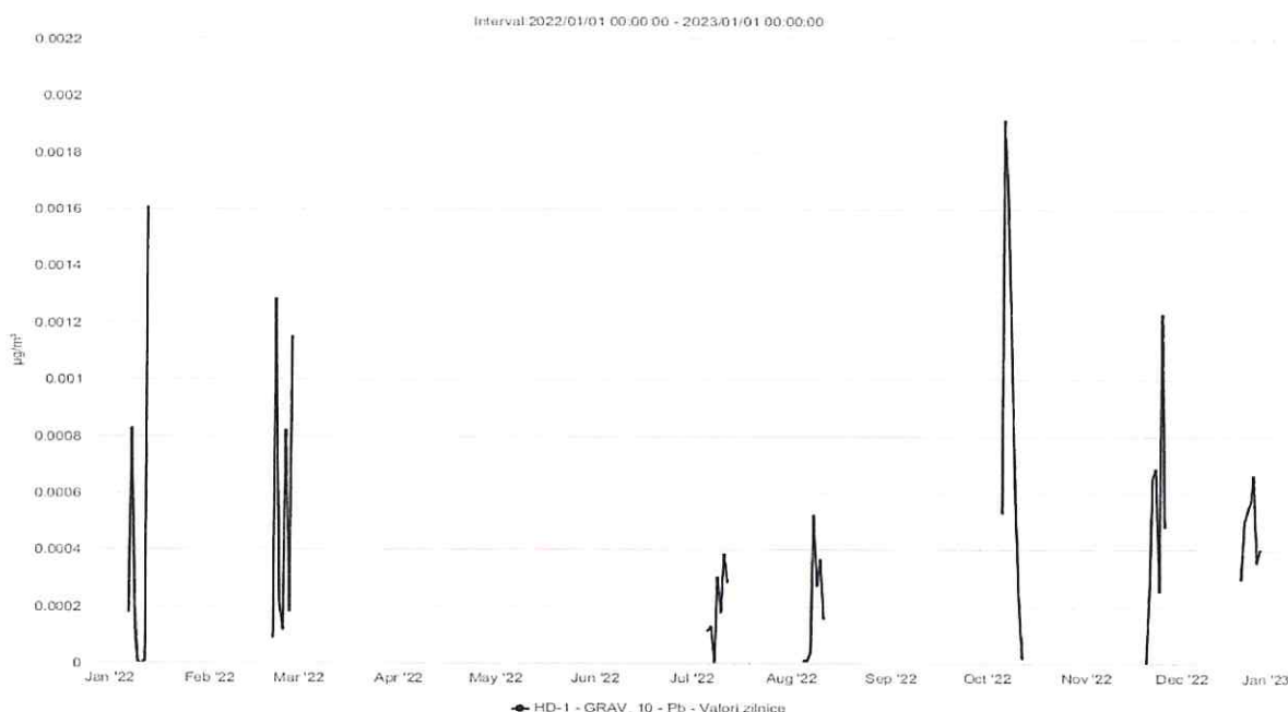
Figura nr. 2.4.1. Evoluția valorilor zilnice de Pb (μg/mc) din PM 10 gravimetric, pe parcursul a 8 săptămâni distribuite uniform pe toată durata anului 2022, la stația automată de monitorizare HD-1 din județul Hunedoara
