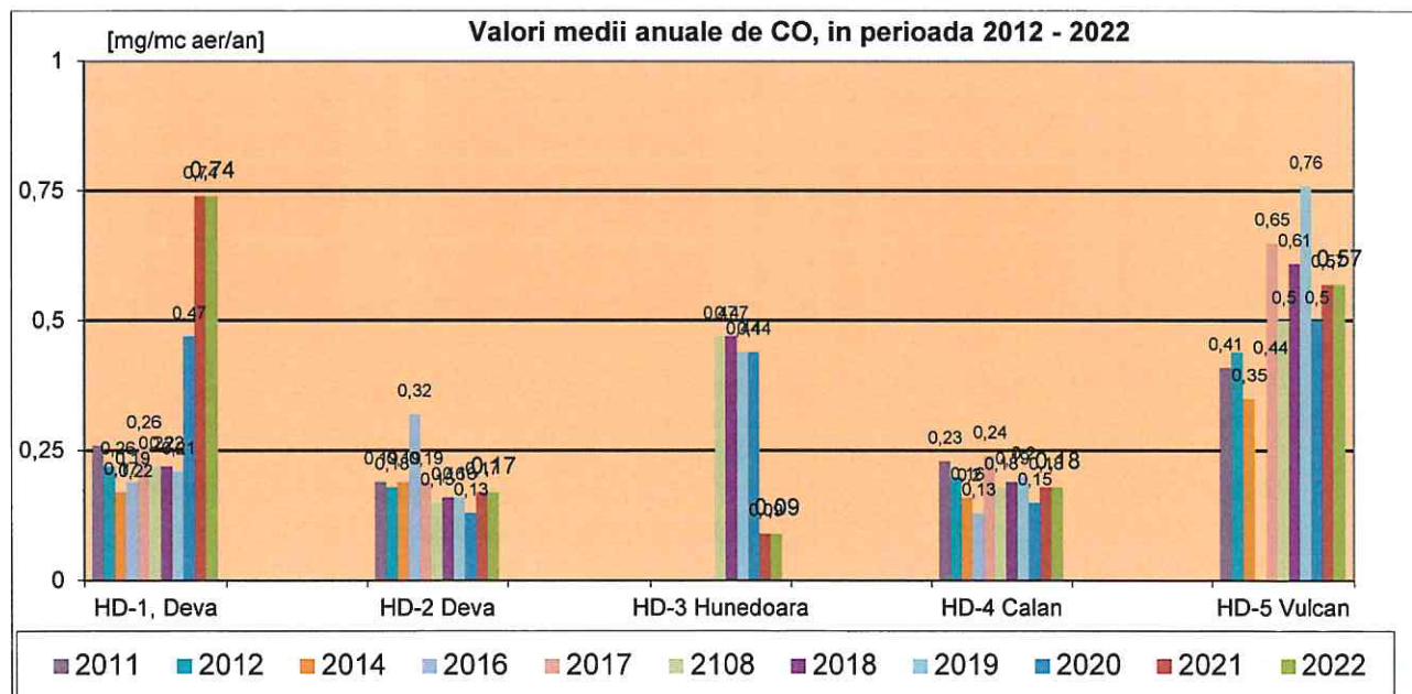
Figura nr. 2.8.5. Evoluția valorilor medii anuale de monoxid de carbon obținute prin rețeaua automată de monitorizare a calității aerului din județul Hunedoara, în perioada 2012 – 2022
