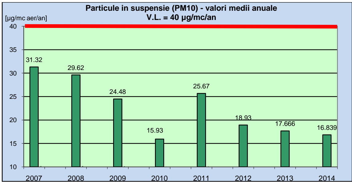
Fig. 2.8.3 Evoluția particulelor în suspensie (PM 10 ), în perioada 2007 – 2014, obținute prin determinări semiautomate la punctul situat în Deva, str. Aurel Vlaicu, nr.25
