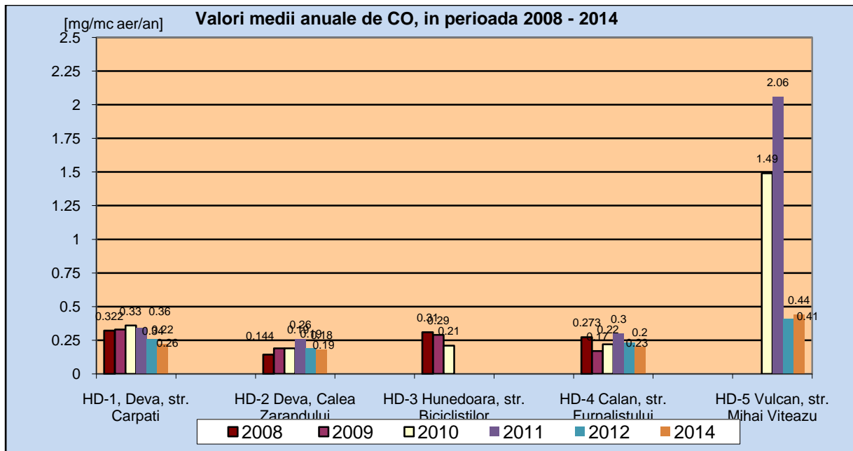
Figura nr. 2.8.5. Evoluția valorilor medii anuale de monoxid de carbon obținute prin rețeaua automată de monitorizare a calității aerului, în perioada 2008 – 2014
