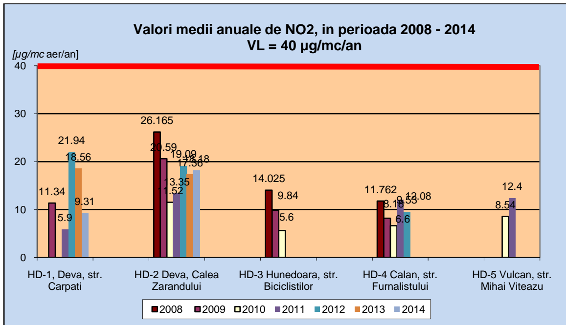
Figura nr. 2.8.1. Evoluția valorilor medii anuale de dioxid de azot obținute prin rețeaua automată de monitorizare a calității aerului, în perioada 2008 - 2014
