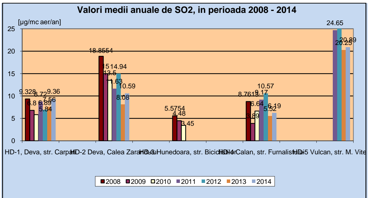
Figura nr. 2.8.2. Evoluția valorilor medii anuale de dioxid de sulf obținute prin rețeaua automată de monitorizare a calității aerului, în perioada 2008 – 2014
