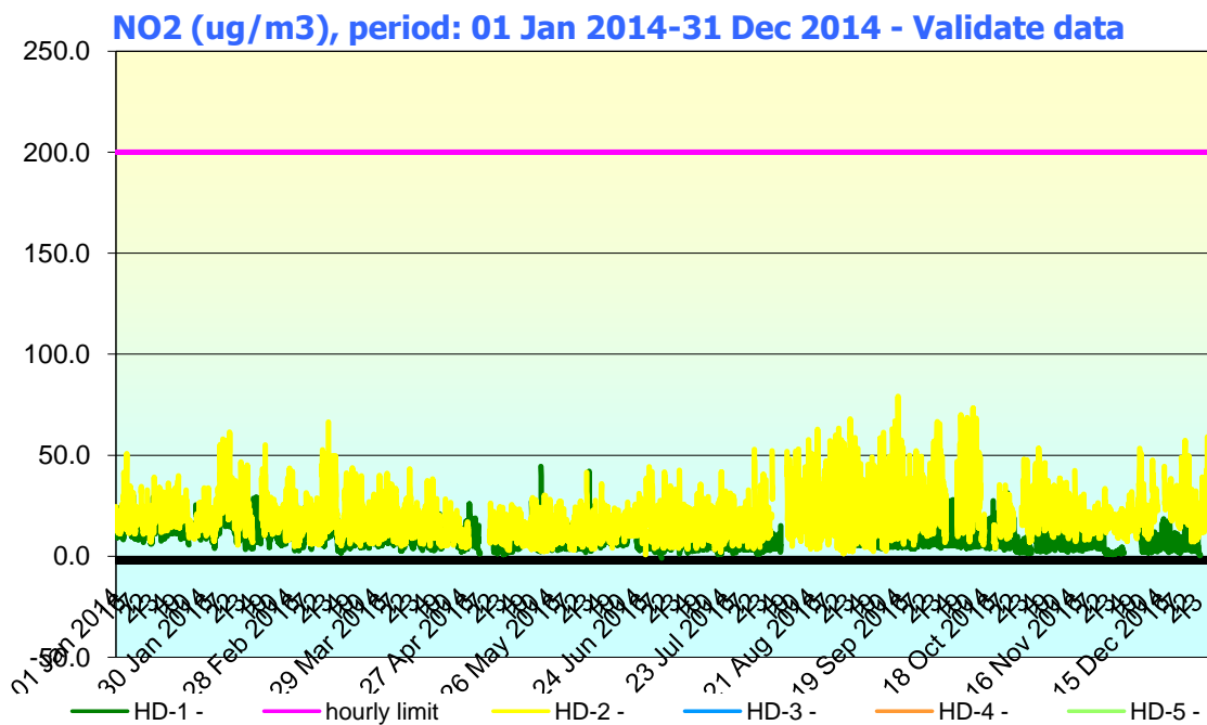
Figura nr. 2 1.1. Evoluția valorilor orare de NO 2 (μg/mc), în anul 2014, la stațiile automate de monitorizare
