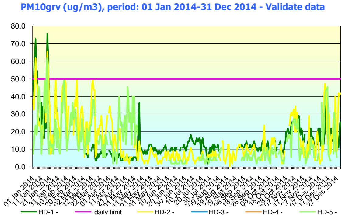
Figura nr. 2.3.2. Evoluția zilnică a valorilor de \text{PM}_{10} ( \mu\text{g}/\text{mc} ) determinat gravimetric în anul 2014, la stațiile automate de monitorizare
