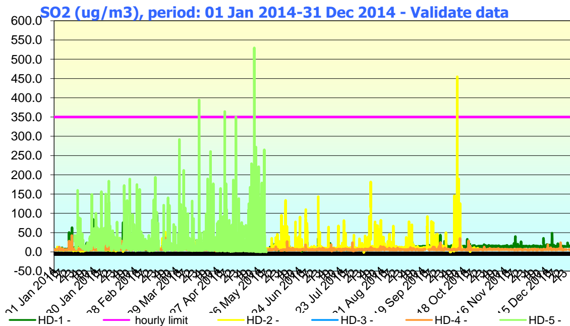
Figura nr. 2.2.1. Evoluția valorilor orare de SO 2 (μg/mc) în anul 2014, la stațiile automate de monitorizare
