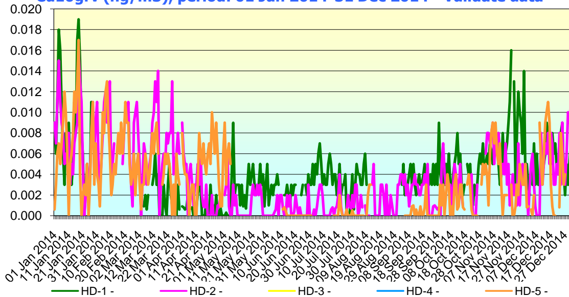
Figura nr. 2.4.2. Evoluția valorilor zilnice de Cd (μg/mc) din PM 10 gravimetric în anul 2014, la stațiile automate de monitorizare
