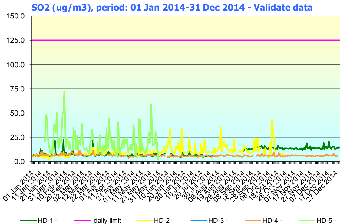
Figura nr. 2.2.2. Evoluția valorilor zilnice de SO 2 (μg/mc) în anul 2014, la stațiile automate de monitorizare
