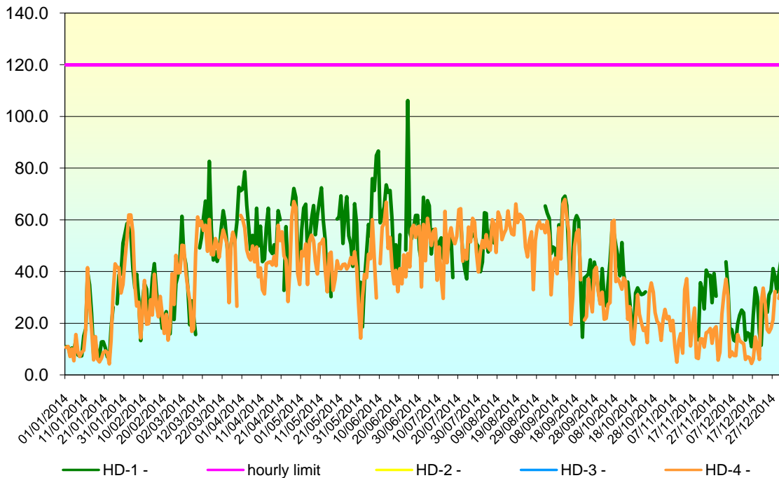
Figura nr. 2.7.2. Evoluția valorilor maxime zilnice a mediilor pe 8 h la ozon ( \mu\text{g}/\text{mc} ) în anul 2014 la stațiile automate de monitorizare
