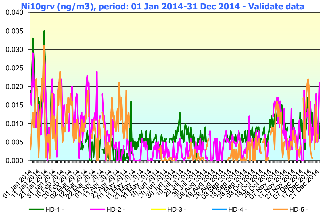
Figura nr. 2.4.3. Evoluția valorilor zilnice de Ni ( \mu\text{g}/\text{mc} ) din \text{PM}_{10} gravimetric în anul 2014, la stațiile automate de monitorizare
