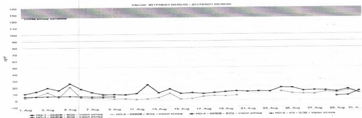
Figura nr. 1.3.3. Evoluția valorilor zilnice de SO 2 (µg/mc), în luna august 2017, la stațiile automate de monitorizare
