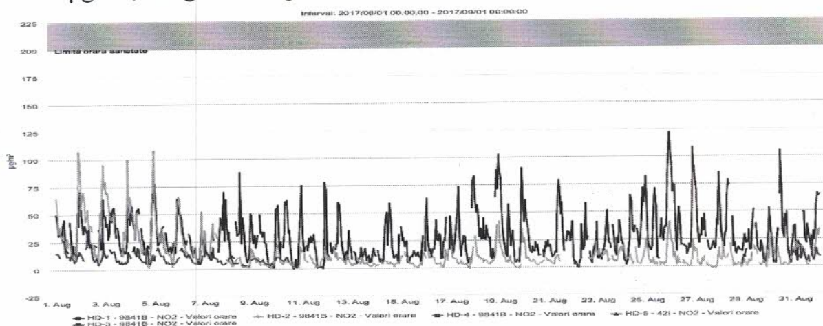
Figura nr. 1.3.4. Evoluția valorilor orare de NO 2 (µg/mc), în luna august 2017, la stațiile automate de monitorizare
