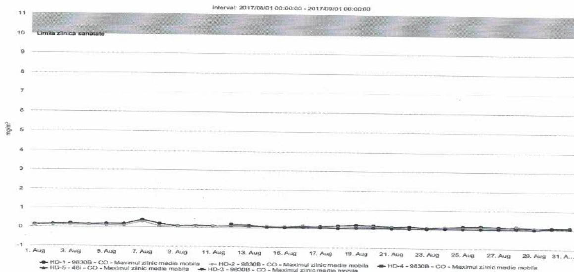
Figura nr. 1.3.5. Evoluția valorilor maxime zilnice a mediilor pe 8 ore la CO (mg/mc), în luna august 2017, la stațiile automate de monitorizare
