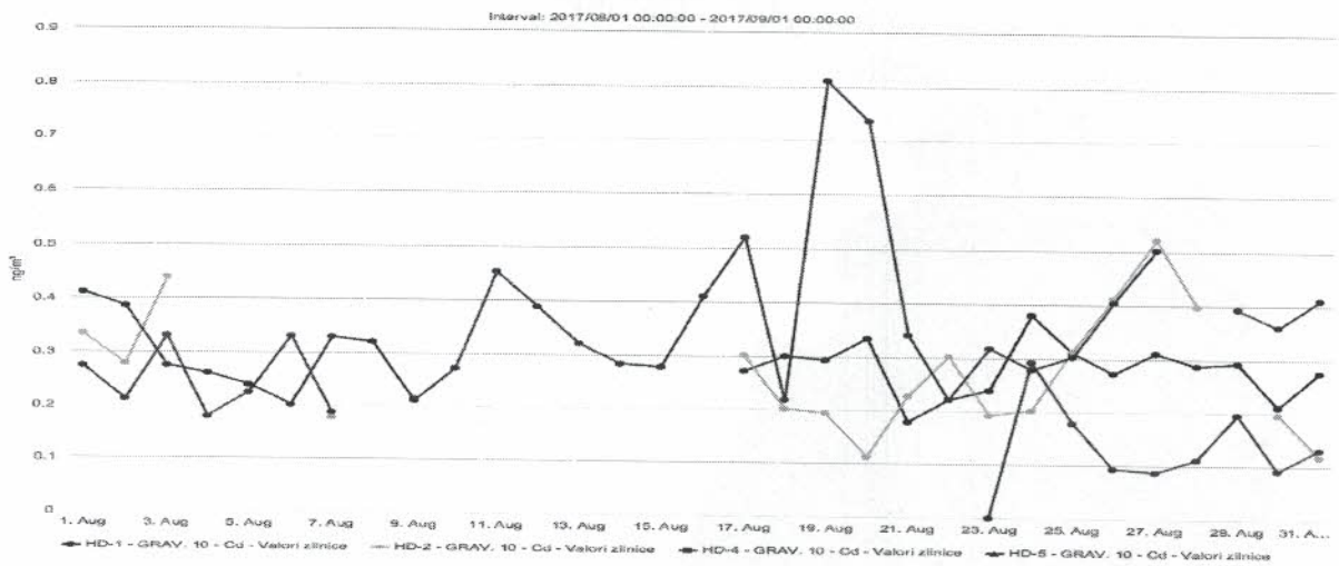
Figura nr. 1.3.9. Evoluția valorilor zilnice de Cd ( \mu\text{g}/\text{mc} ) din \text{PM}_{10} gravimetric, în luna august 2017, la stațiile automate de monitorizare
