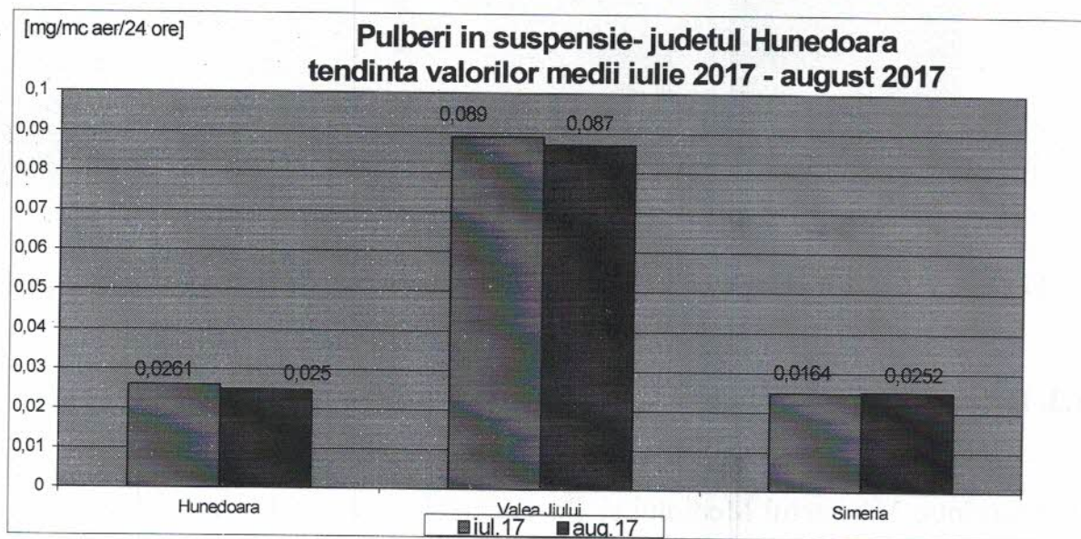
Fig. nr. 1.2.1.1. Evoluția calității pulberilor în suspensie în perioada iulie 2017 – august 2017
