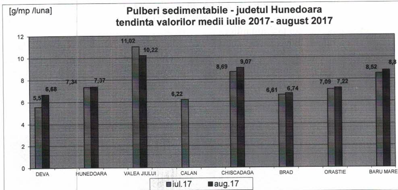
Fig. nr. 1.2.1.2. Evoluția calității pulberilor sedimentabile în perioada iulie 2017 – august 2017
