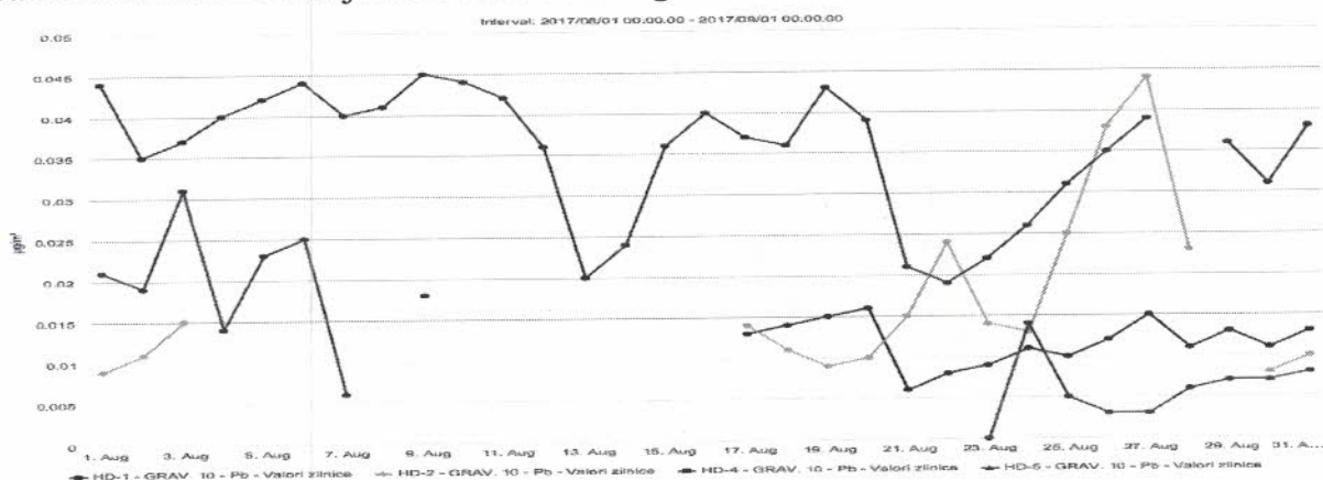
Figura nr. 1.3.8. Evoluția valorilor zilnice de Pb ( \mu\text{g}/\text{mc} ) din PM_{10} gravimetric, în luna august 2017, la stațiile automate de monitorizare
