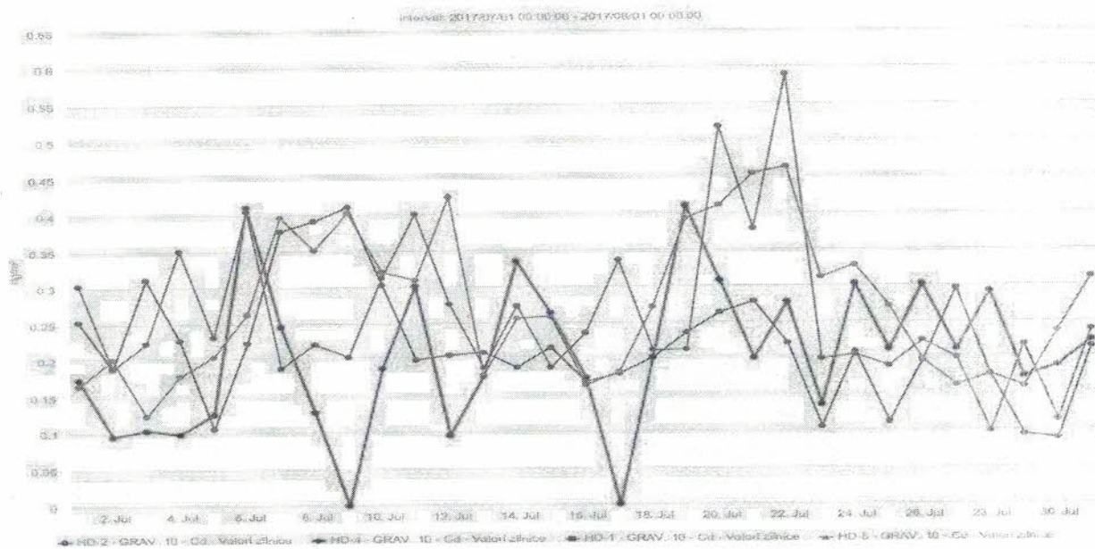
Figura nr. 1.3.9. Evoluția valorilor zilnice de Cd ( \mu\text{g}/\text{mc} ) din \text{PM}_{10} gravimetric, în luna iulie 2017, la stațiile automate de monitorizare
