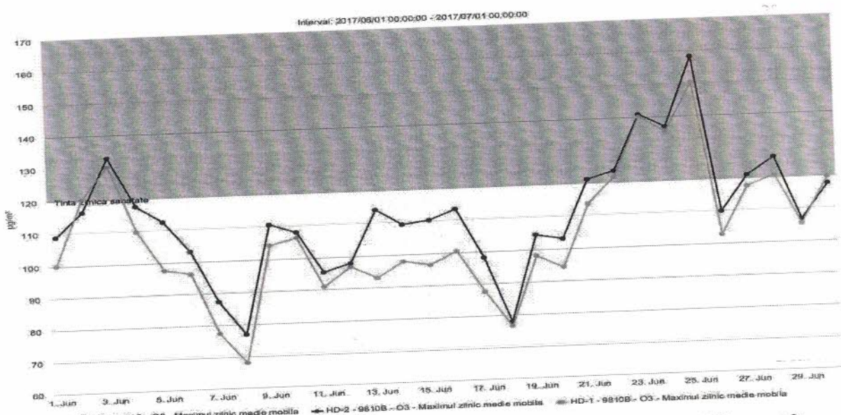
Figura nr. 1.3.6. Evoluția valorilor maxime zilnice a mediilor pe 8 ore la ozon (µg/mc), în luna iunie 2017, la stațiile automate de monitorizare
