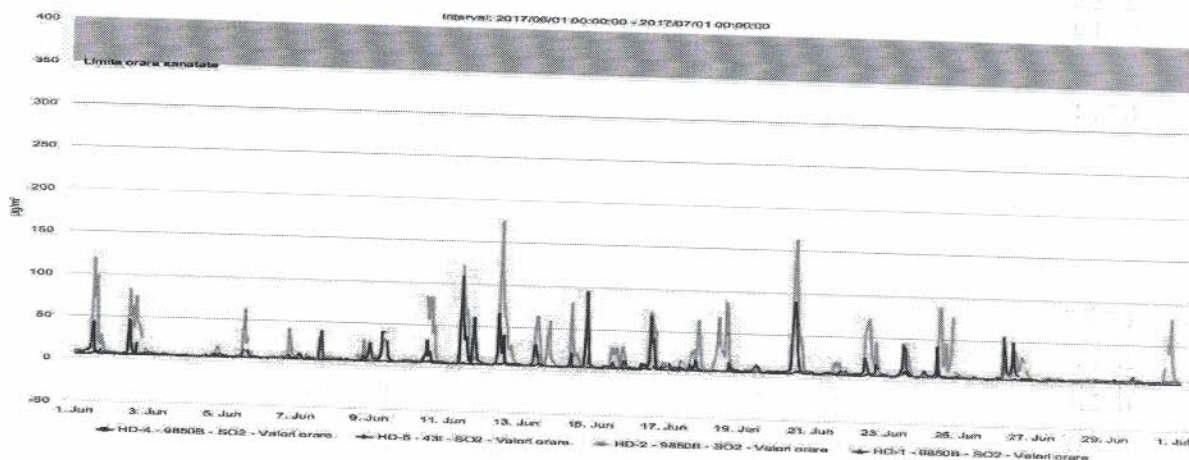
Figura nr. 1.3.2. Evoluția valorilor orare de SO 2 ( \mu\text{g}/\text{mc} ), în luna iunie 2017 la stațiile automate de monitorizare
