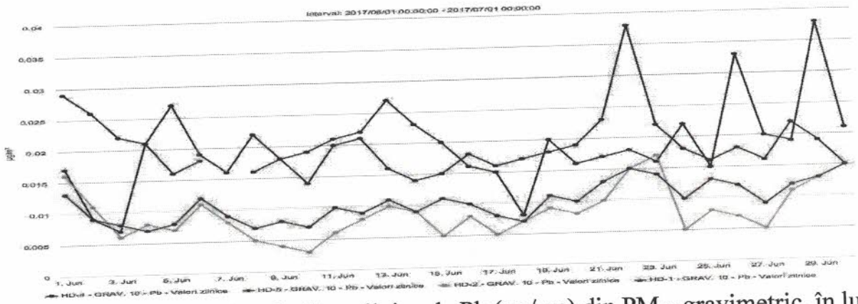
Figura nr. 1.3.8. Evoluția valorilor zilnice de Pb ( \mu\text{g}/\text{mc} ) din \text{PM}_{10} gravimetric, în luna iunie 2017, la stațiile automate de monitorizare
