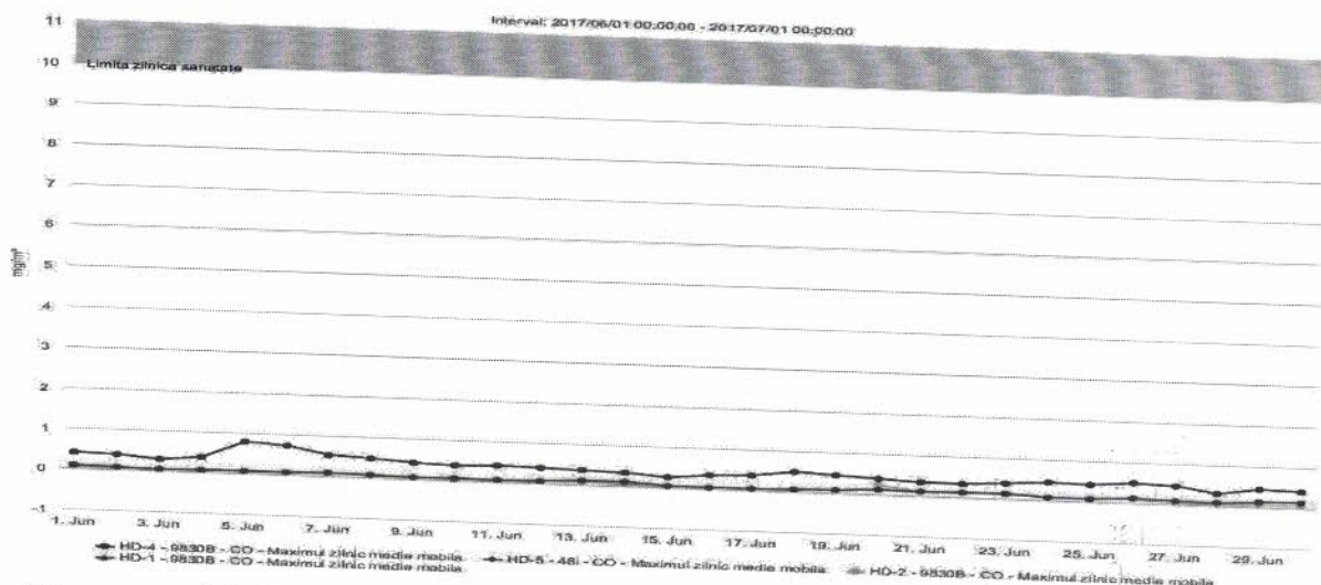
Figura nr. 1.3.5. Evoluția valorilor maxime zilnice a mediilor pe 8 ore la CO (mg/mc), în luna iunie 2017, la stațiile automate de monitorizare
