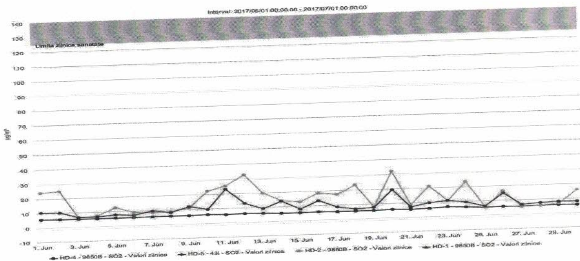
Figura nr. 1.3.3. Evoluția valorilor zilnice de SO2 ( \mu\text{g}/\text{mc} ), în luna iunie 2017, la stațiile automate de monitorizare
