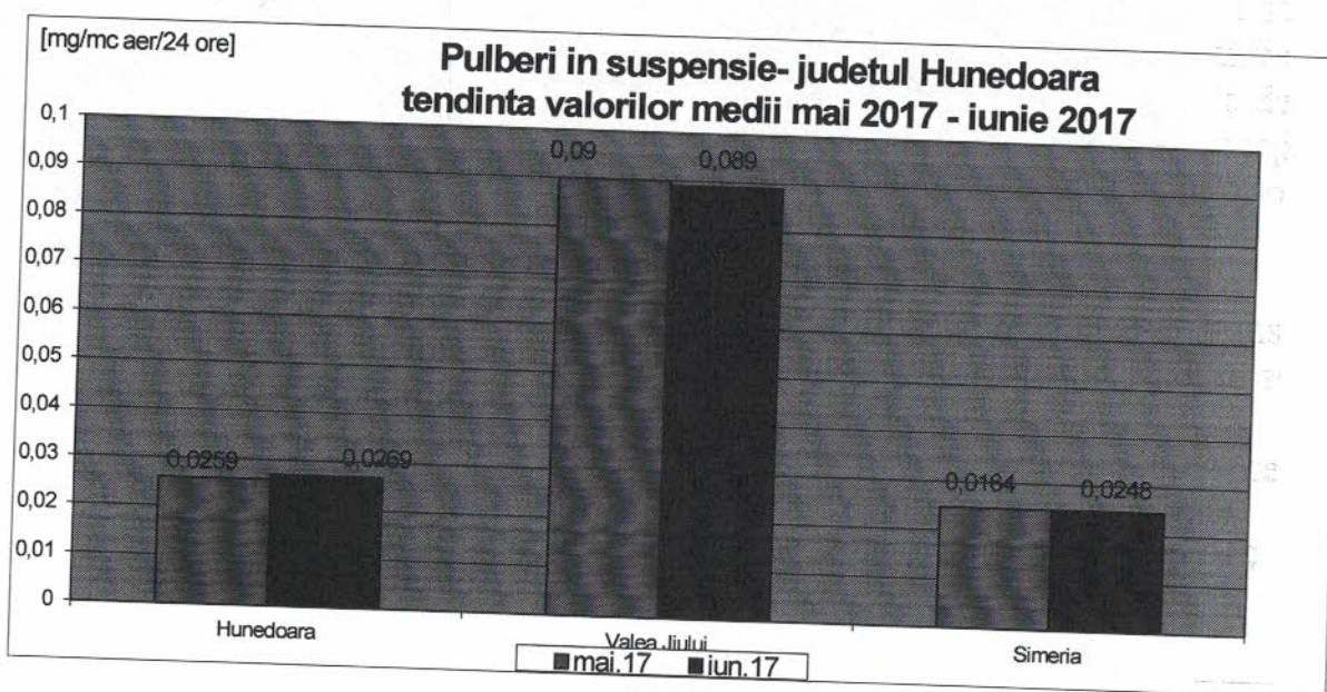
Fig. nr. 1.2.1.1. Evoluția calității pulberilor în suspensie în perioada mai 2017 – iunie 2017
