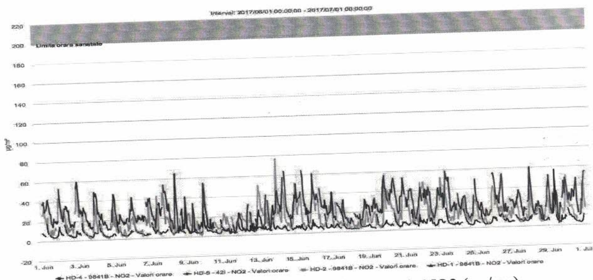
Figura nr. 1.3.4. Evoluția valorilor orare de NO2 ( \mu\text{g}/\text{mc} ), în luna iunie 2017, la stațiile automate de monitorizare
