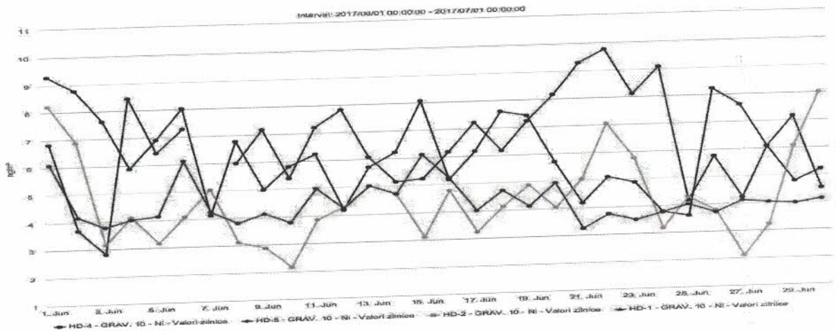
Figura nr.1.3.10. Evoluția valorilor zilnice de Ni ( \mu\text{g}/\text{mc} ) din \text{PM}_{10} gravimetric, în luna iunie 2017, la stațiile automate de monitorizare
