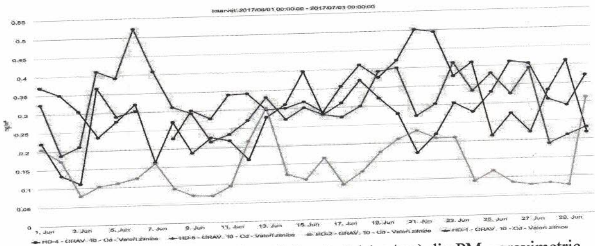
Figura nr. 1.3.9. Evoluția valorilor zilnice de Cd ( \mu\text{g}/\text{mc} ) din \text{PM}_{10} gravimetric, în luna iunie 2017, la stațiile automate de monitorizare
