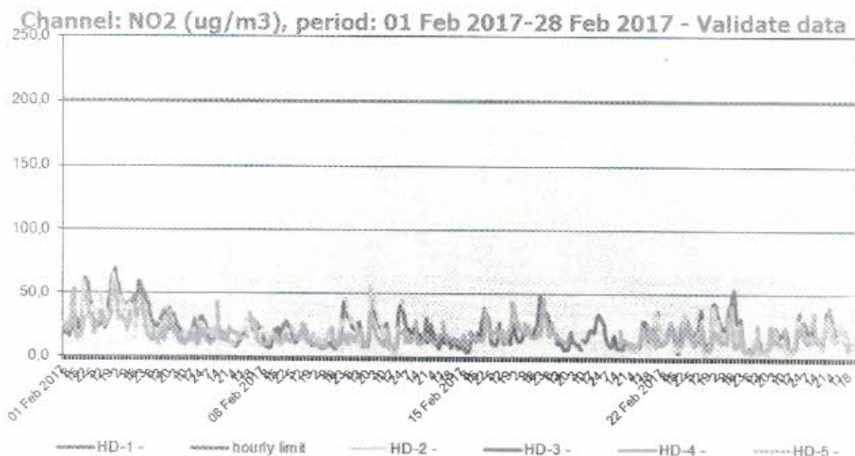
Figura nr. 1.3.4. Evoluția valorilor orare de NO 2 ( \mu\text{g}/\text{mc} ), în luna februarie 2017, la stațiile automate de monitorizare
