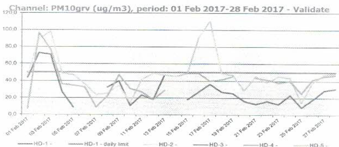
Figura nr. 1.3.7. Evoluția zilnică a valorilor de PM 10 (μg/mc) determinat gravimetric, în luna februarie 2017, la stațiile automate de monitorizare
