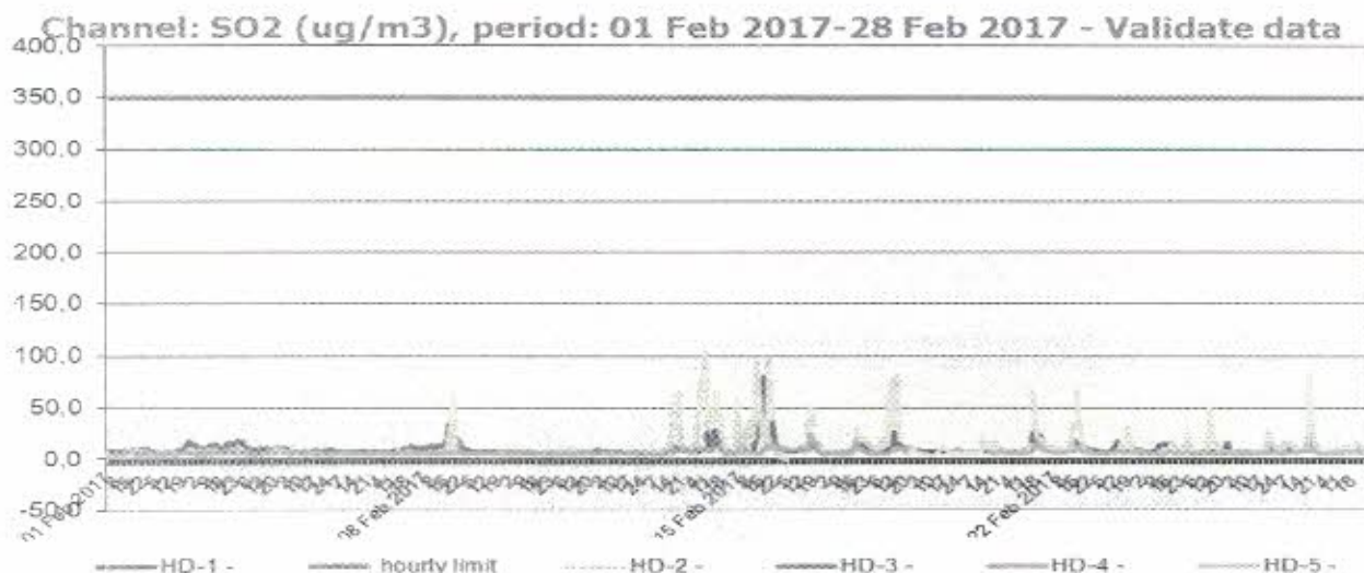
Figura nr. 1.3.2. Evoluția valorilor orare de SO2 ( \mu\text{g}/\text{mc} ), în luna februarie 2017 la stațiile automate de monitorizare
