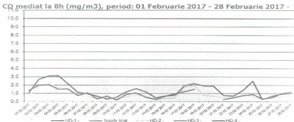
Figura nr. 1.3.5. Evoluția valorilor maxime zilnice a mediilor pe 8 ore la CO (mg/mc), în luna februarie 2017, la stațiile automate de monitorizare
