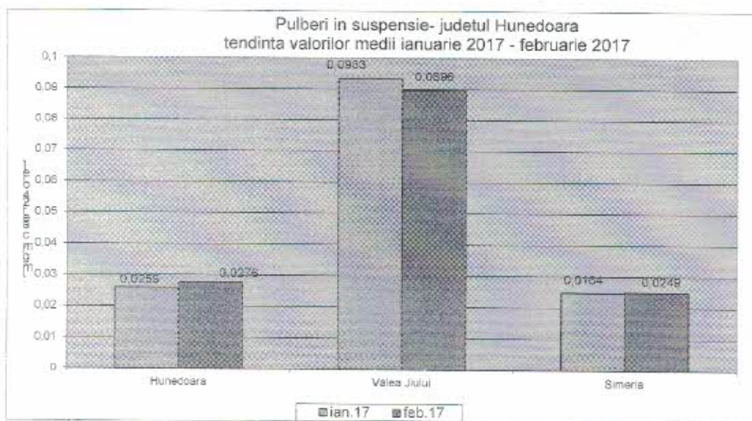
Fig. nr. 1.2.1.1. Evoluția calității pulberilor în suspensie în perioada ianuarie 2017 – februarie 2017
