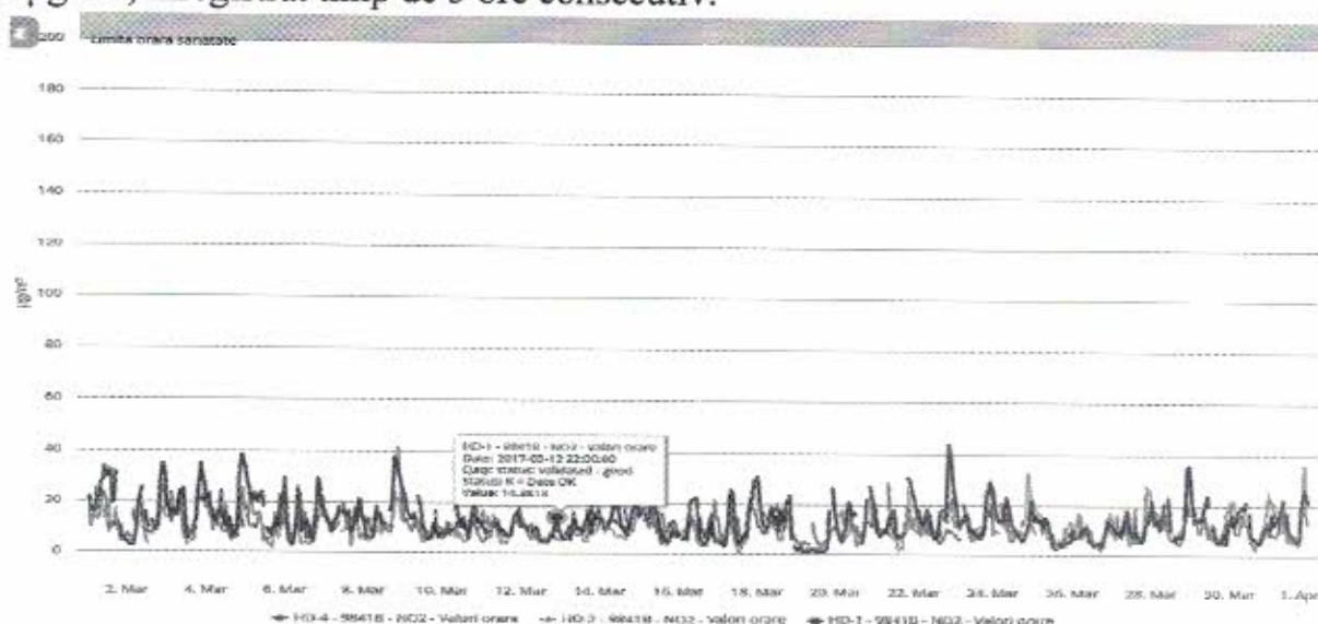
Figura nr. 1.3.4. Evoluția valorilor orare de NO2 ( \mu\text{g}/\text{mc} ), în luna martie 2017, la stațiile automate de monitorizare
