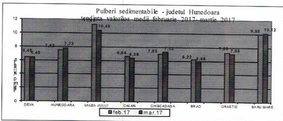
Fig. nr. 1.2.1.2. Evoluția calității pulberilor sedimentabile în perioada februarie 2017 - martie 2017
