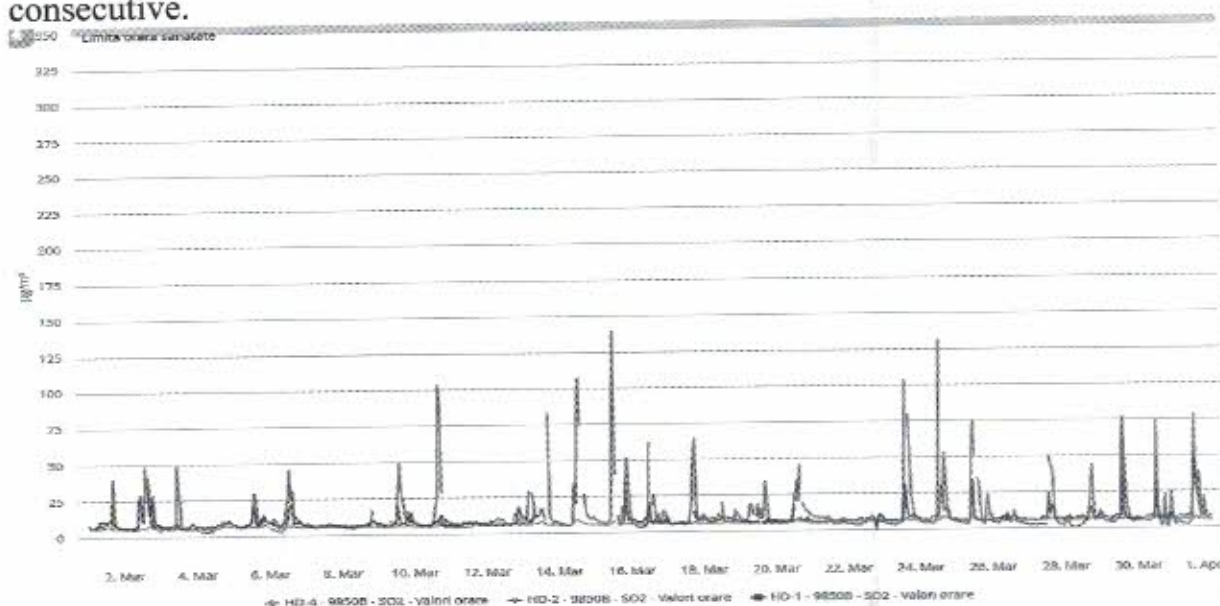
Figura nr. 1.3.2. Evoluția valorilor orare de SO 2 (μg/mc), în luna martie 2017 la stațiile automate de monitorizare
