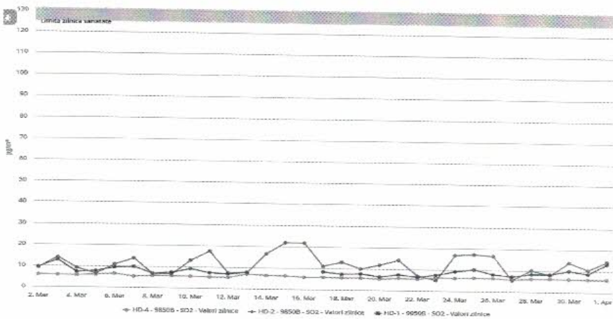
Figura nr. 1.3.3. Evoluția valorilor zilnice de SO2 ( \mu\text{g}/\text{mc} ), în luna martie 2017, la stațiile automate de monitorizare
