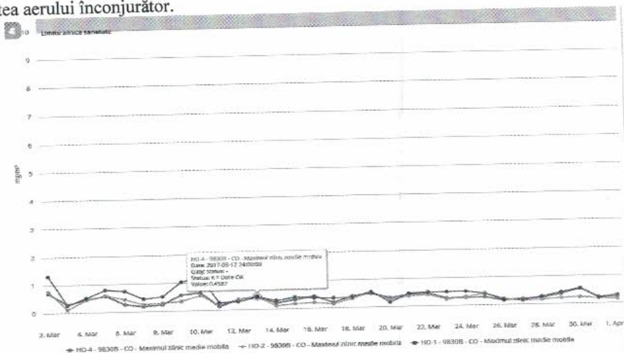
Figura nr. 1.3.5. Evoluția valorilor maxime zilnice a mediilor pe 8 ore la CO (mg/mc), în luna martie 2017, la stațiile automate de monitorizare
