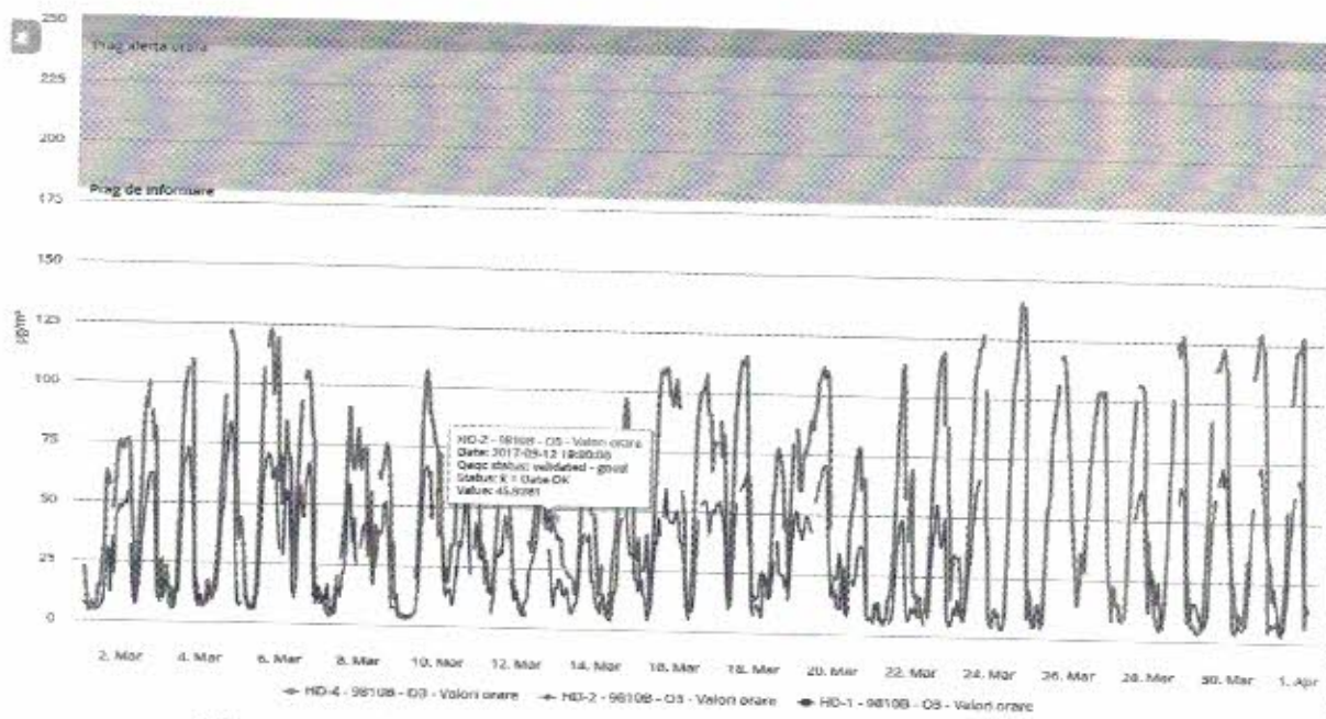
Figura nr. 1.3.6. Evoluția valorilor maxime zilnice a mediilor pe 8 ore la ozon ( \mu\text{g}/\text{mc} ), în luna martie 2017, la stațiile automate de monitorizare
