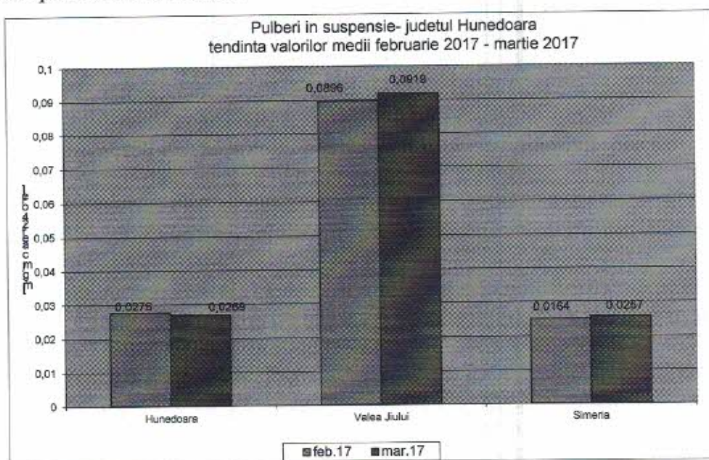
Fig. nr. 1.2.1.1. Evoluția calității pulberilor în suspensie în perioada februarie 2017 – martie 2017
