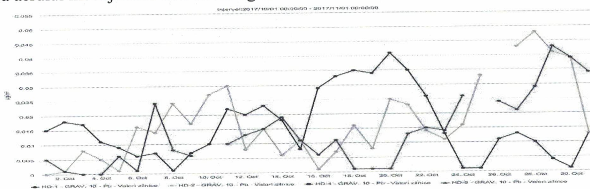
Figura nr. 1.3.8. Evoluția valorilor zilnice de Pb (µg/mc) din PM 10 gravimetric, în luna octombrie 2017, la stațiile automate de monitorizare
