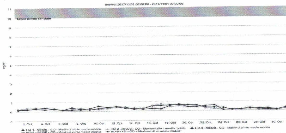
Figura nr. 1.3.5. Evoluția valorilor maxime zilnice a mediilor pe 8 ore la CO (mg/mc), în luna octombrie 2017, la stațiile automate de monitorizare
