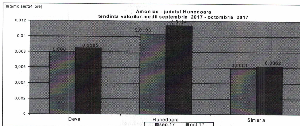
Fig. nr. 1.2.1. Evoluția calității amoniacului în perioada septembrie 2017 – octombrie 2017
