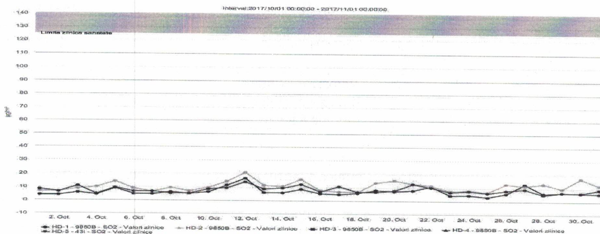
Figura nr. 1.3.3. Evoluția valorilor zilnice de SO2 ( \mu\text{g}/\text{mc} ), în luna octombrie 2017, la stațiile automate de monitorizare
