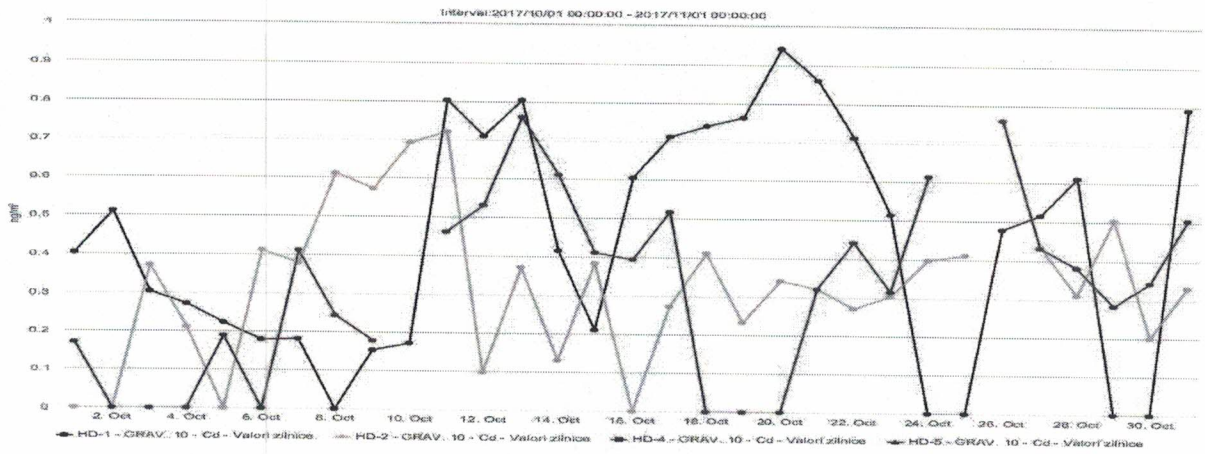
Figura nr. 1.3.9. Evoluția valorilor zilnice de Cd ( \mu\text{g}/\text{mc} ) din \text{PM}_{10} gravimetric, în luna octombrie 2017, la stațiile automate de monitorizare
