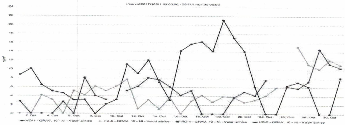
Figura nr.1.3.10. Evoluția valorilor zilnice de Ni ( \mu\text{g}/\text{mc} ) din \text{PM}_{10} gravimetric, în luna octombrie 2017, la stațiile automate de monitorizare
