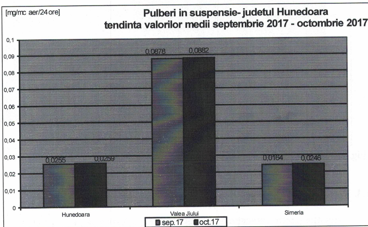
Fig. nr. 1.2.1.1. Evoluția calității pulberilor în suspensie în perioada septembrie 2017 – octombrie 2017
