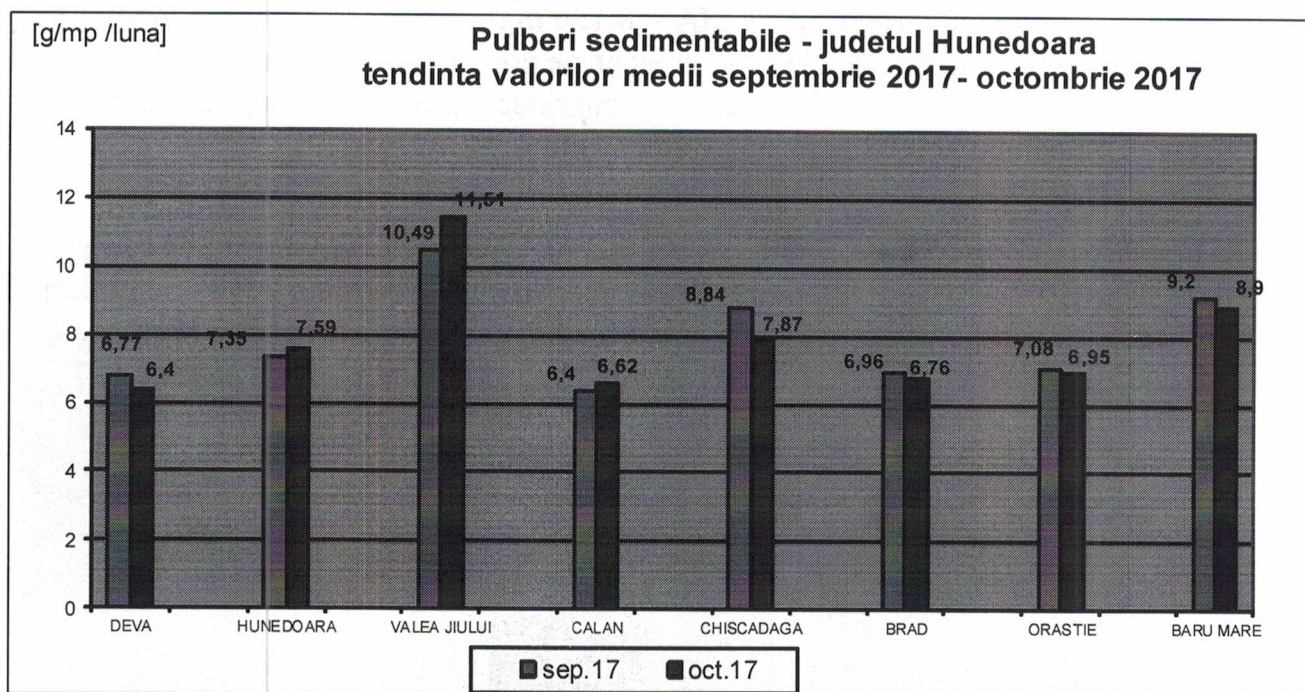
Fig. nr. 1.2.1.2. Evoluția calității pulberilor sedimentabile în perioada septembrie 2017 – octombrie 2017
