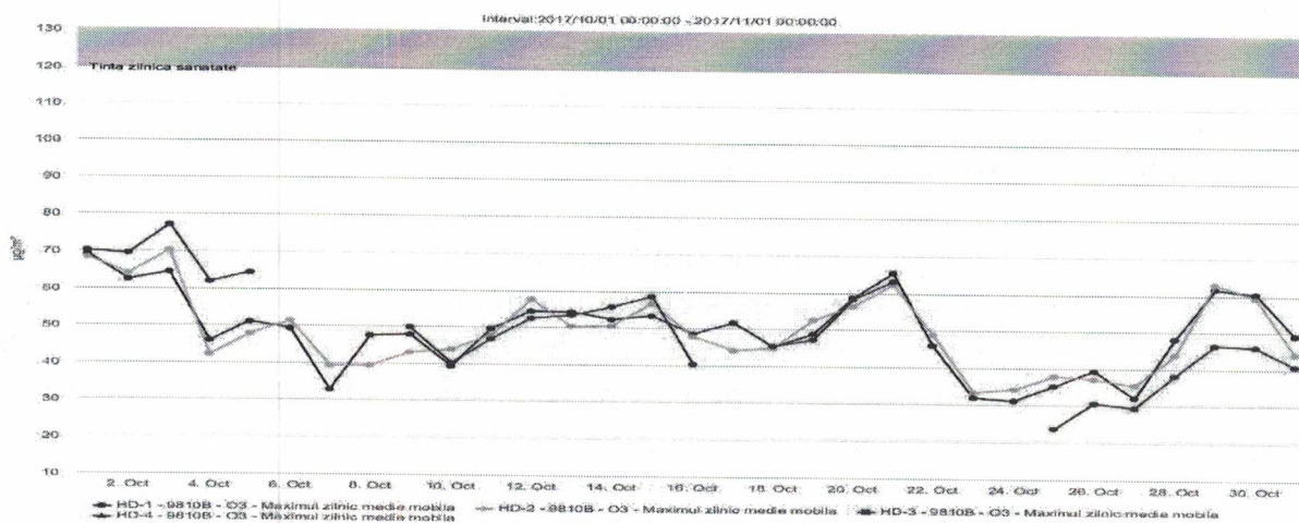
Figura nr. 1.3.6. Evoluția valorilor maxime zilnice a mediilor pe 8 ore la ozon ( \mu\text{g}/\text{mc} ), în luna octombrie 2017, la stațiile automate de monitorizare
