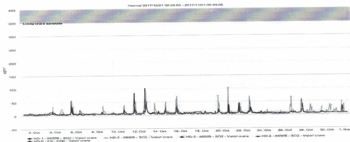
Figura nr. 1.3.2. Evoluția valorilor orare de SO 2 ( \mu\text{g}/\text{mc} ), în luna octombrie 2017 la stațiile automate de monitorizare
