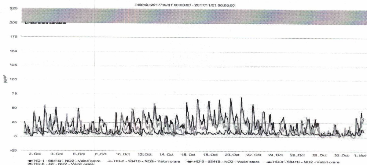
Figura nr. 1.3.4. Evoluția valorilor orare de NO2 ( \mu\text{g}/\text{mc} ), în luna octombrie 2017, la stațiile automate de monitorizare
