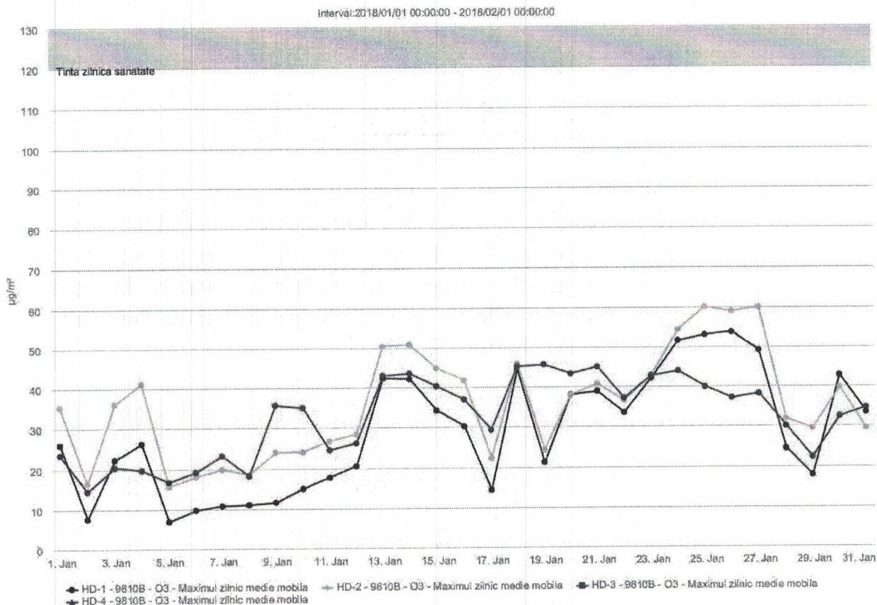
Figura nr. 1.3.6. Evoluția valorilor maxime zilnice a mediilor pe 8 ore la ozon ( \mu\text{g}/\text{m}^3 ), în luna ianuarie 2018, la stațiile automate de monitorizare
