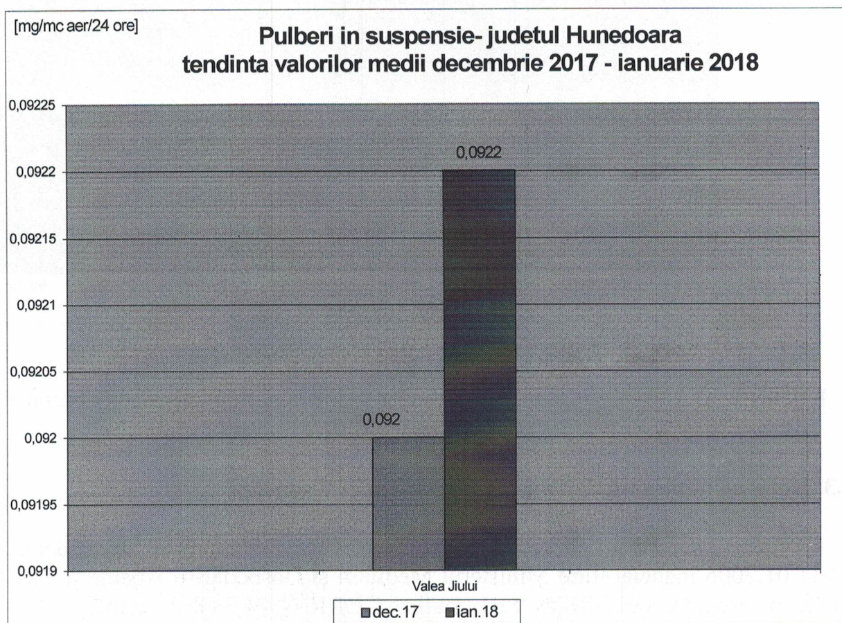
Fig. nr. 1.2.1.1. Evoluția calității pulberilor în suspensie în perioada decembrie 2017 – ianuarie 2018
