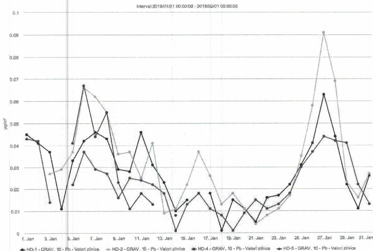
Figura nr. 1.3.8. Evoluția valorilor zilnice de Pb (μg/mc) din PM 10 gravimetric, în luna ianuarie 2018, la stațiile automate de monitorizare
