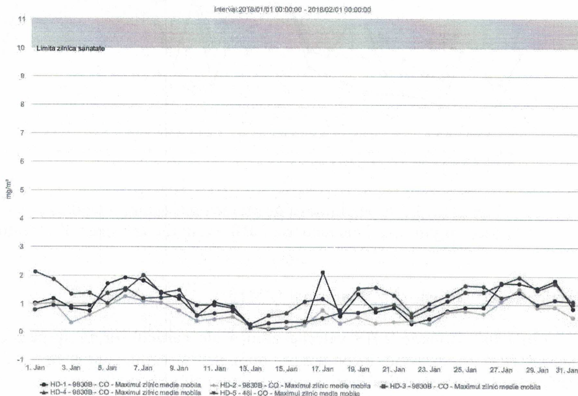
Figura nr. 1.3.5. Evoluția valorilor maxime zilnice a mediilor pe 8 ore la CO (mg/mc), în luna ianuarie 2018, la stațiile automate de monitorizare
