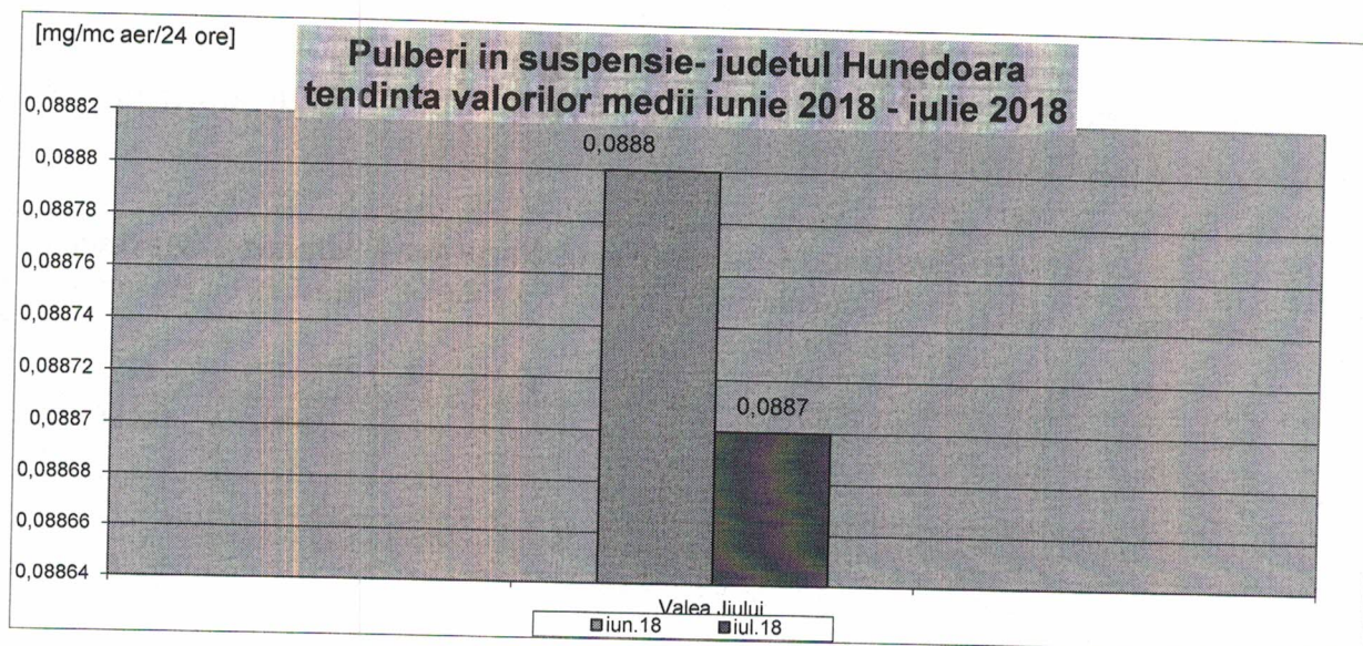
Fig. nr. 1.2.1.1. Evoluția calității pulberilor în suspensie în perioada iunie 2018 – iulie 2018
