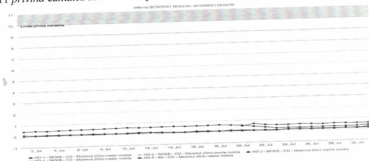
Figura nr. 1.3.5. Evoluția valorilor maxime zilnice a mediilor pe 8 ore la CO (mg/mc), în luna iulie 2018, la stațiile automate de monitorizare
