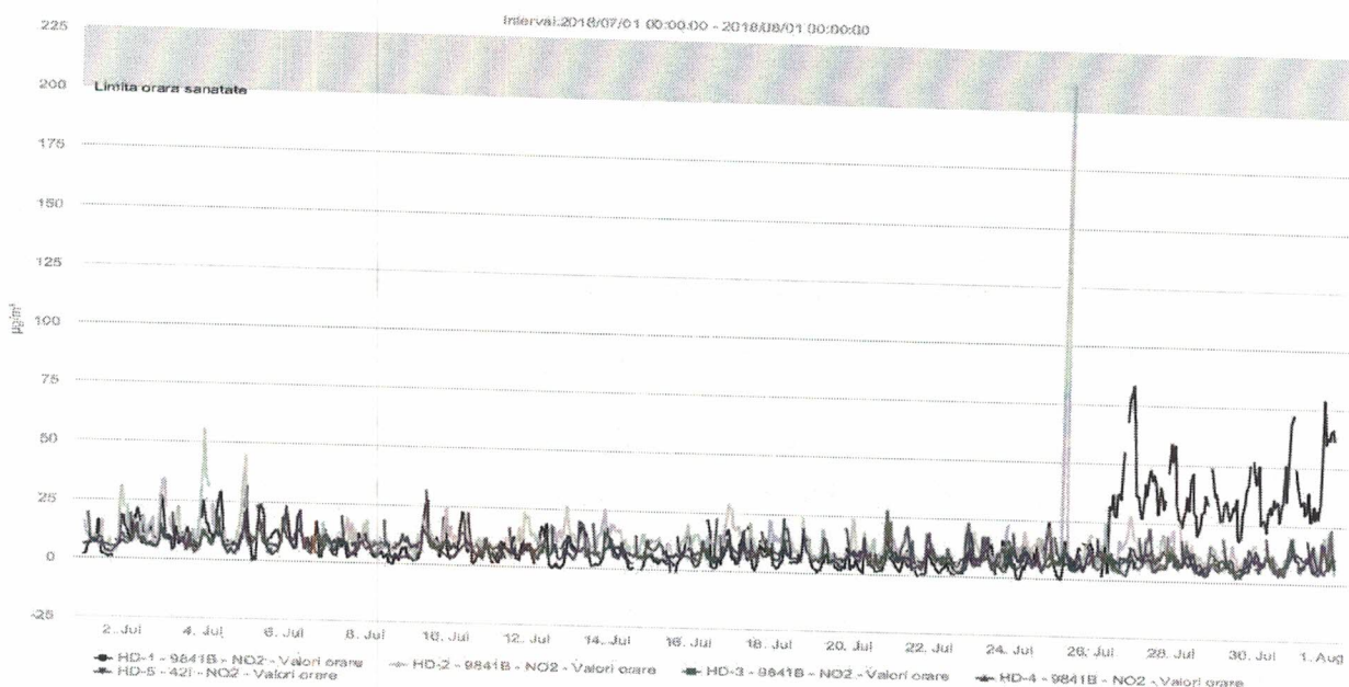
Figura nr. 1.3.4. Evoluția valorilor orare de NO 2 (µg/mc), în luna iulie 2018, la stațiile automate de monitorizare
