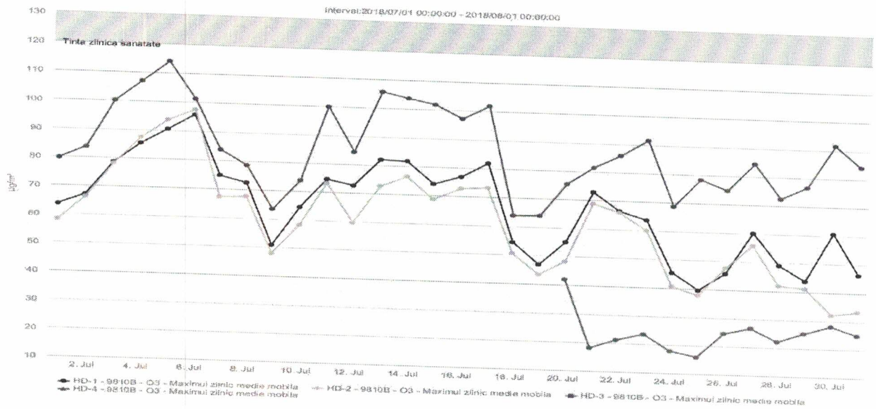
Figura nr. 1.3.6. Evoluția valorilor maxime zilnice a mediilor pe 8 ore la ozon ( \mu\text{g}/\text{mc} ), în luna iulie 2018, la stațiile automate de monitorizare
