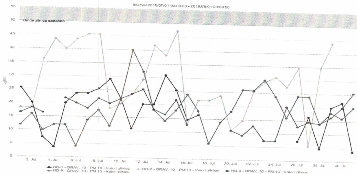
Figura nr. 1.3.7. Evoluția zilnică a valorilor de PM 10 ( \mu\text{g}/\text{mc} ) determinat gravimetric, în luna iulie 2018, la stațiile automate de monitorizare
