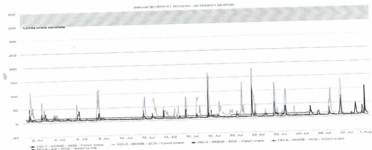
Figura nr. 1.3.2. Evoluția valorilor orare de SO 2 ( \mu\text{g}/\text{mc} ), în luna iulie 2018 la stațiile automate de monitorizare
