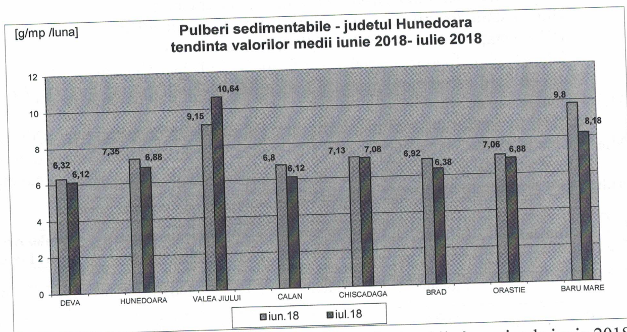
Fig. nr. 1.2.1.2. Evoluția calității pulberilor sedimentabile în perioada iunie 2018 – iulie 2018
