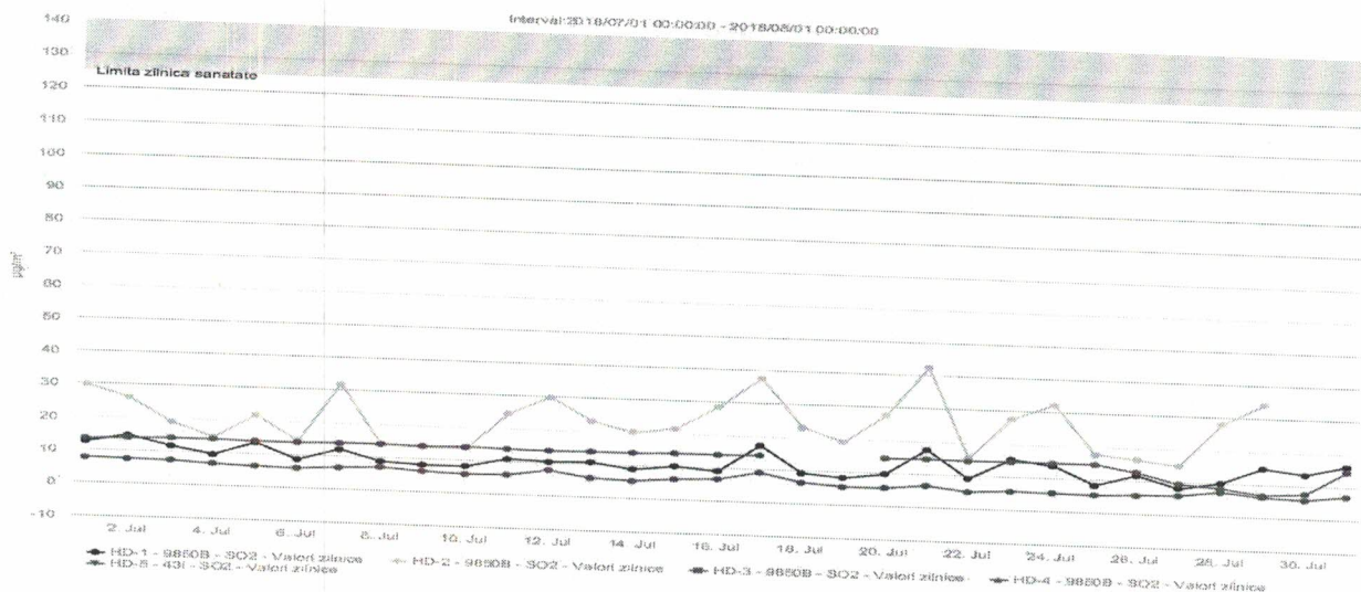
Figura nr. 1.3.3. Evoluția valorilor zilnice de SO 2 (µg/mc), în luna iulie 2018, la stațiile automate de monitorizare
