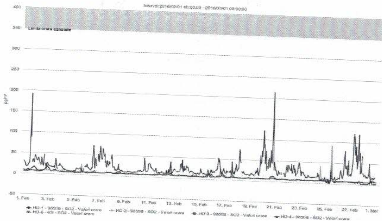
Figura nr. 1.3.2. Evoluția valorilor orare de SO 2 (µg/mc), în luna februarie 2018 la stațiile automate de monitorizare
