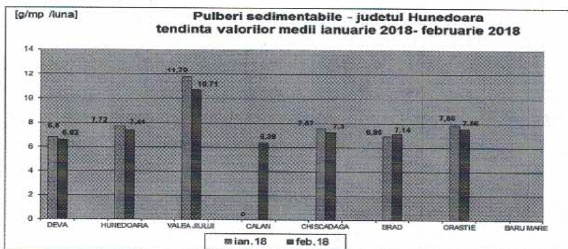
Fig. nr. 1.2.1.2. Evoluția calității pulberilor sedimentabile în perioada ianuarie 2018 – februarie 2018
