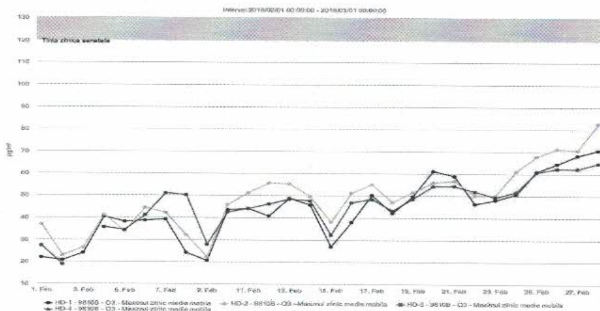
Figura nr. 1.3.6. Evoluția valorilor maxime zilnice a mediilor pe 8 ore la ozon ( \mu\text{g}/\text{mc} ), în luna februarie 2018, la stațiile automate de monitorizare
