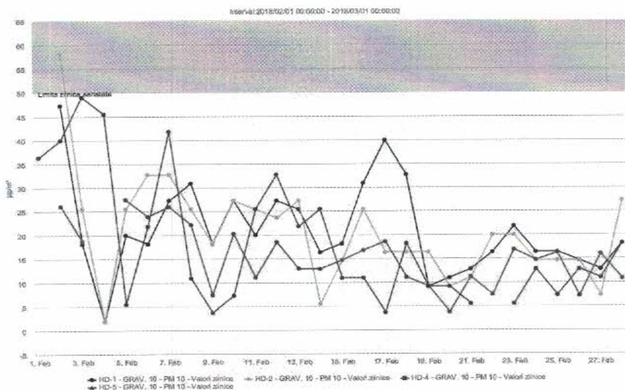
Figura nr. 1.3.7. Evoluția zilnică a valorilor de PM 10 (µg/mc) determinat gravimetric, în luna februarie 2018, la stațiile automate de monitorizare
