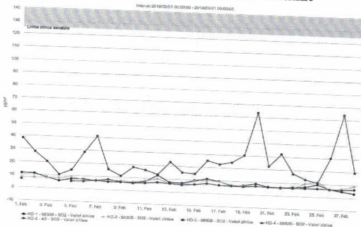
Figura nr. 1.3.3. Evoluția valorilor zilnice de SO 2 (µg/mc), în luna februarie 2018, la stațiile automate de monitorizare
