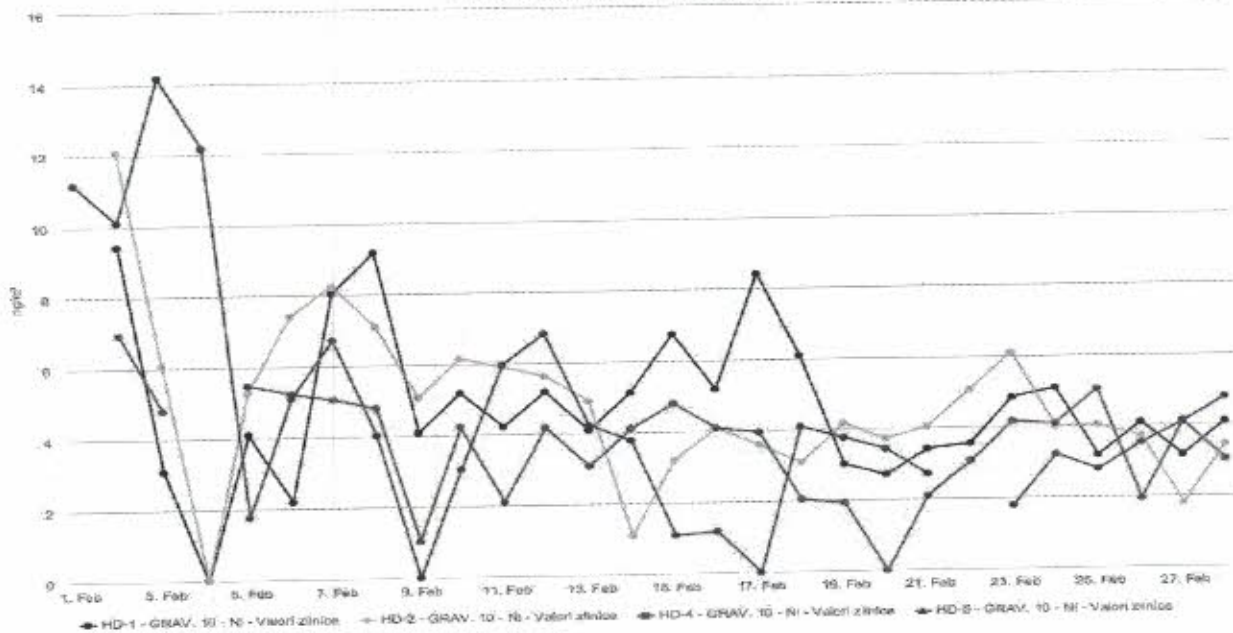
Figura nr.1.3.10. Evoluția valorilor zilnice de Ni ( \mu\text{g}/\text{mc} ) din \text{PM}_{10} gravimetric, în luna februarie 2018, la stațiile automate de monitorizare
