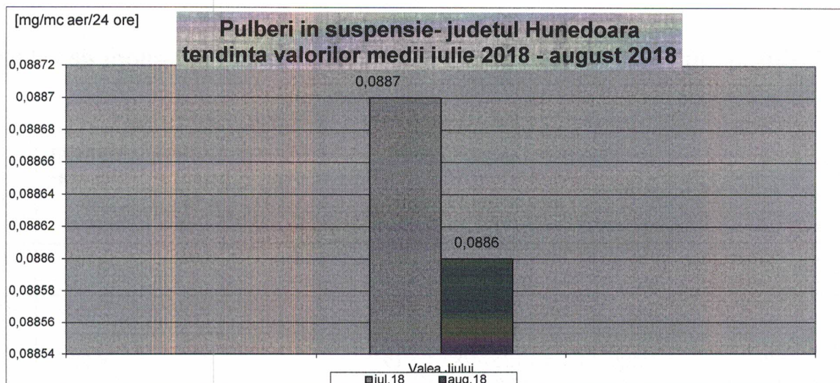
Fig. nr. 1.2.1.1. Evoluția calității pulberilor în suspensie în perioada iulie 2018 – august 2018
