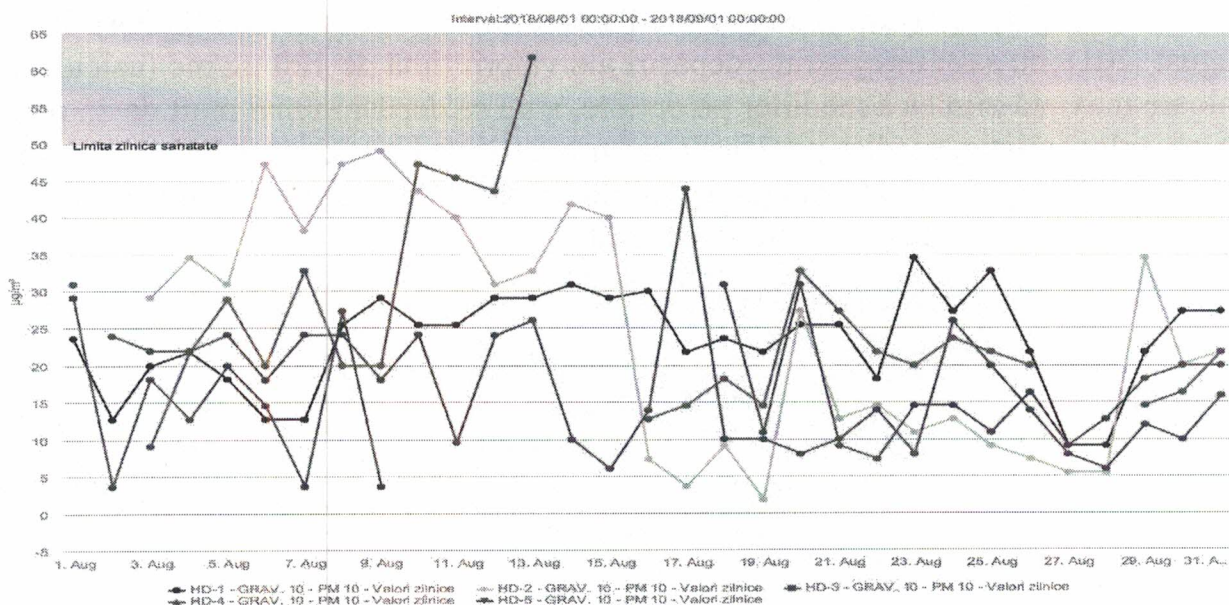
Figura nr. 1.3.7. Evoluția zilnică a valorilor de PM 10 ( \mu\text{g}/\text{mc} ) determinat gravimetric, în luna august 2018, la stațiile automate de monitorizare
