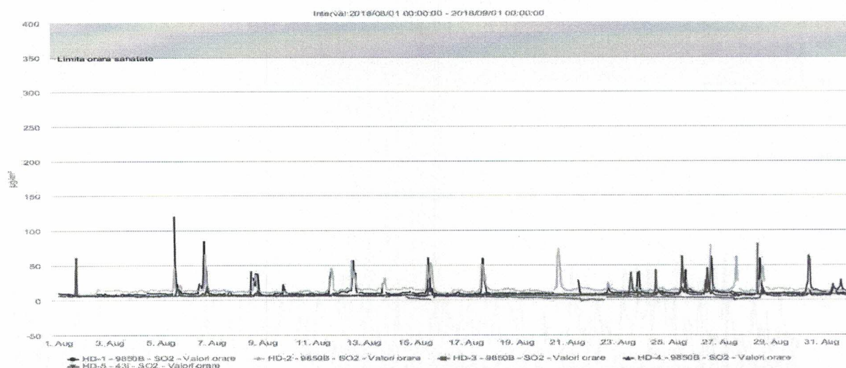
Figura nr. 1.3.2. Evoluția valorilor orare de SO 2 ( \mu\text{g}/\text{mc} ), în luna august 2018 la stațiile automate de monitorizare
