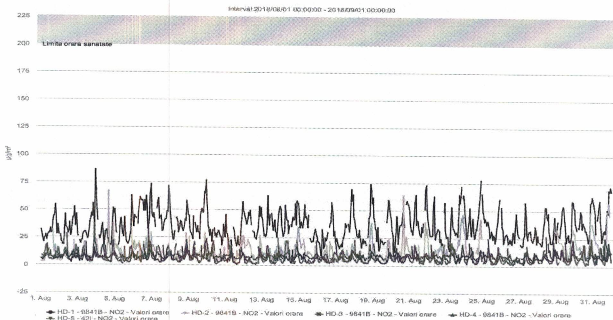
Figura nr. 1.3.4. Evoluția valorilor orare de NO 2 (µg/mc), în luna august 2018, la stațiile automate de monitorizare
