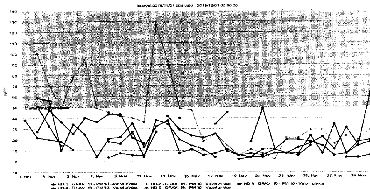
Figura nr. 1.3.7. Evoluția zilnică a valorilor de PM 10 (µg/mc) determinat gravimetric, în luna noiembrie 2018, la stațiile automate de monitorizare
