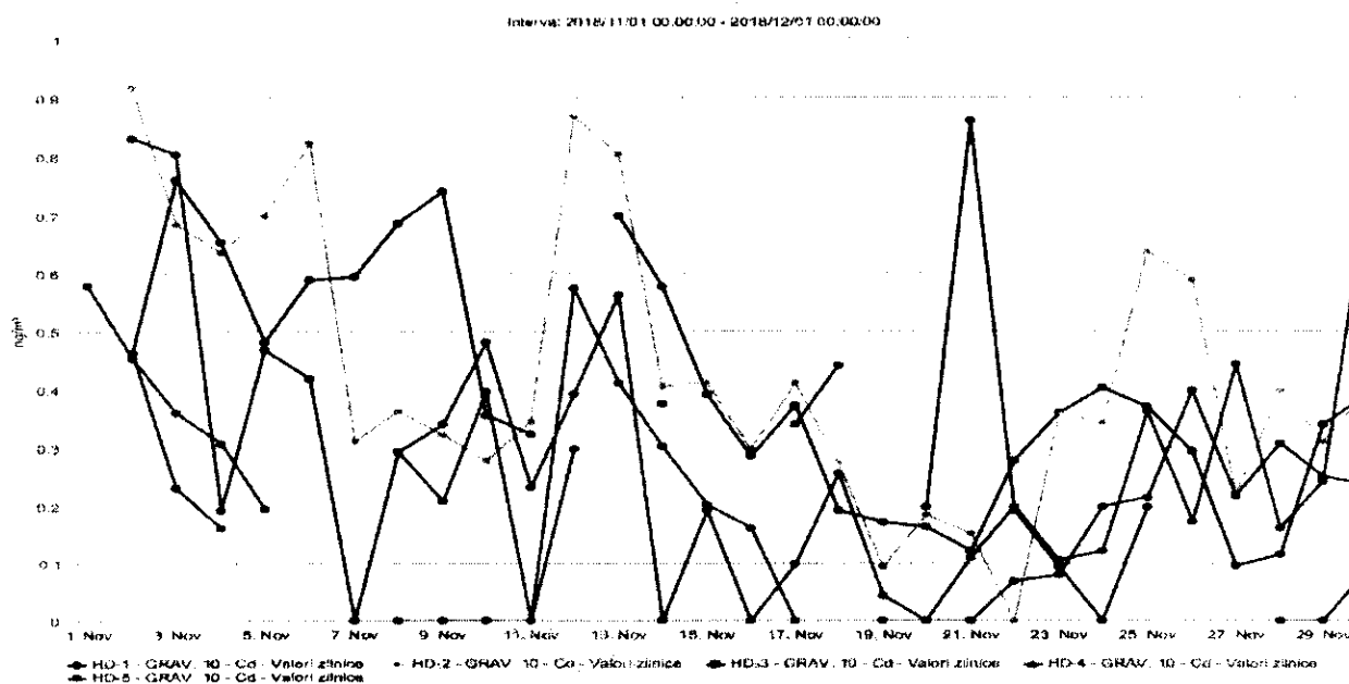
Figura nr. 1.3.9. Evoluția valorilor zilnice de Cd ( \mu\text{g}/\text{mc} ) din \text{PM}_{10} gravimetric, în luna noiembrie 2018, la stațiile automate de monitorizare
