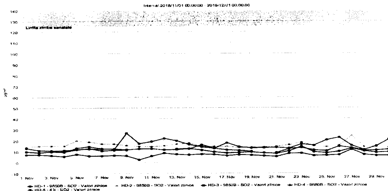
Figura nr. 1.3.3. Evoluția valorilor zilnice de SO 2 (µg/mc), în luna noiembrie 2018, la stațiile automate de monitorizare
