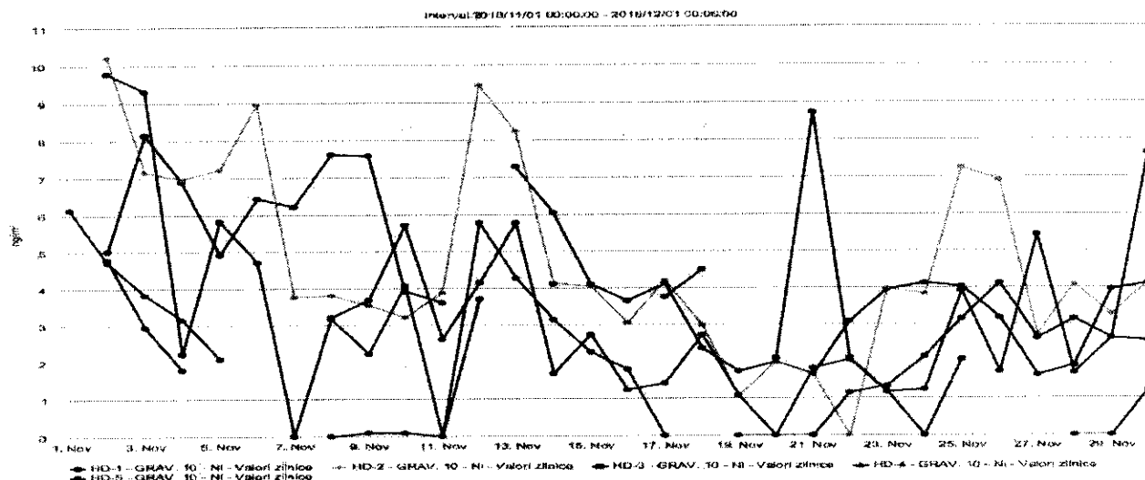
Figura nr.1.3.10. Evoluția valorilor zilnice de Ni ( \mu\text{g}/\text{mc} ) din \text{PM}_{10} gravimetric, în luna noiembrie 2018, la stațiile automate de monitorizare
