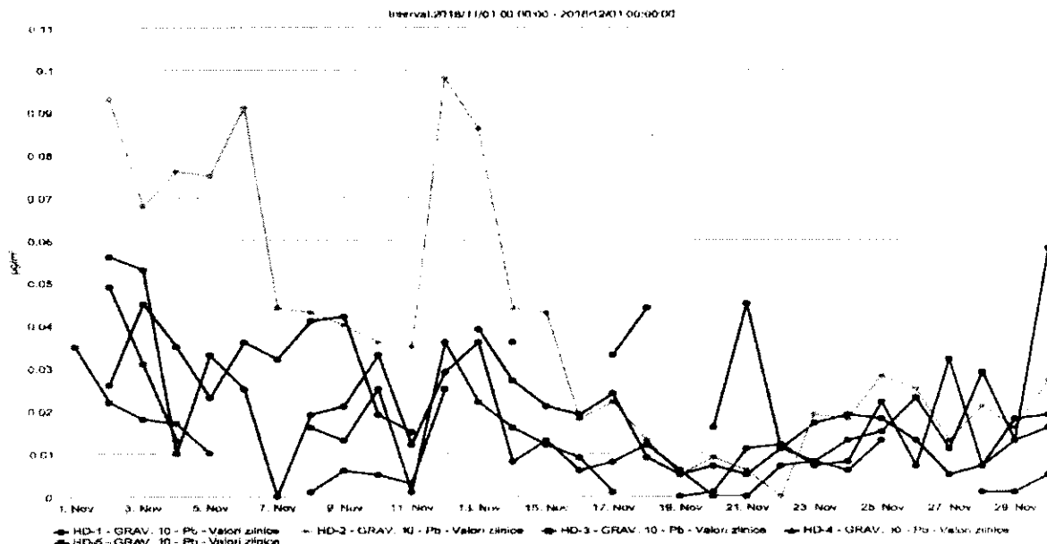
Figura nr. 1.3.8. Evoluția valorilor zilnice de Pb ( \mu\text{g}/\text{mc} ) din \text{PM}_{10} gravimetric, în luna noiembrie 2018, la stațiile automate de monitorizare
