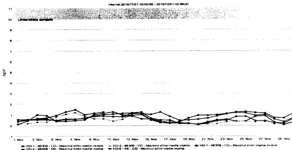
Figura nr. 1.3.5. Evoluția valorilor maxime zilnice a mediilor pe 8 ore la CO (mg/mc), în luna noiembrie 2018, la stațiile automate de monitorizare
