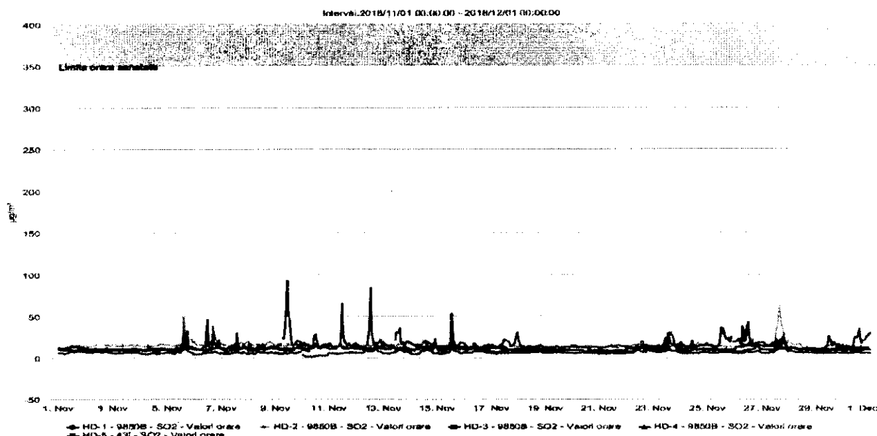
Figura nr. 1.3.2. Evoluția valorilor orare de SO 2 ( \mu\text{g}/\text{mc} ), în luna noiembrie 2018 la stațiile automate de monitorizare
