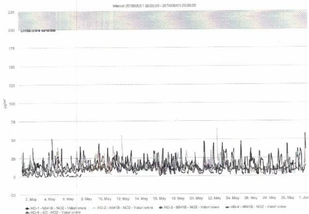
Figura nr. 1.3.4. Evoluția valorilor orare de NO 2 ( \mu\text{g}/\text{mc} ), în luna mai 2018, la stațiile automate de monitorizare
