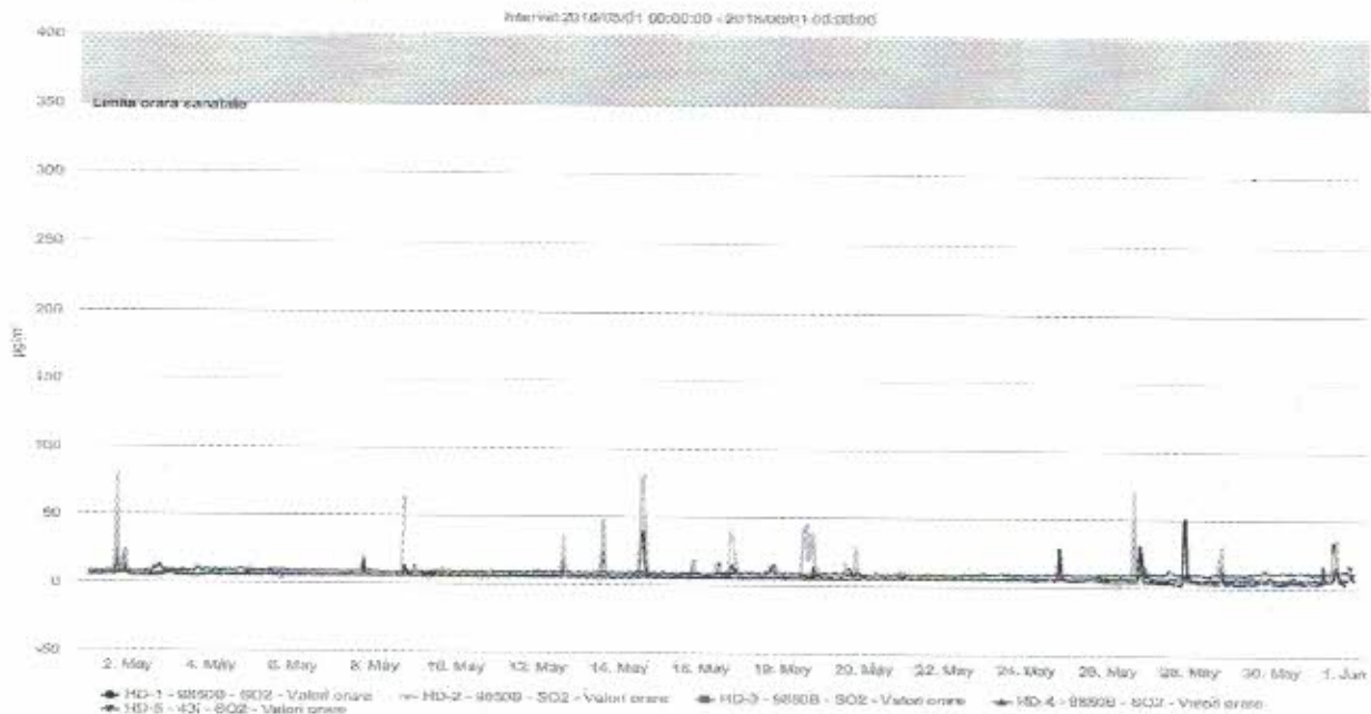
Figura nr. 1.3.2. Evoluția valorilor orare de SO 2 ( \mu\text{g}/\text{mc} ), în luna mai 2018 la stațiile automate de monitorizare
