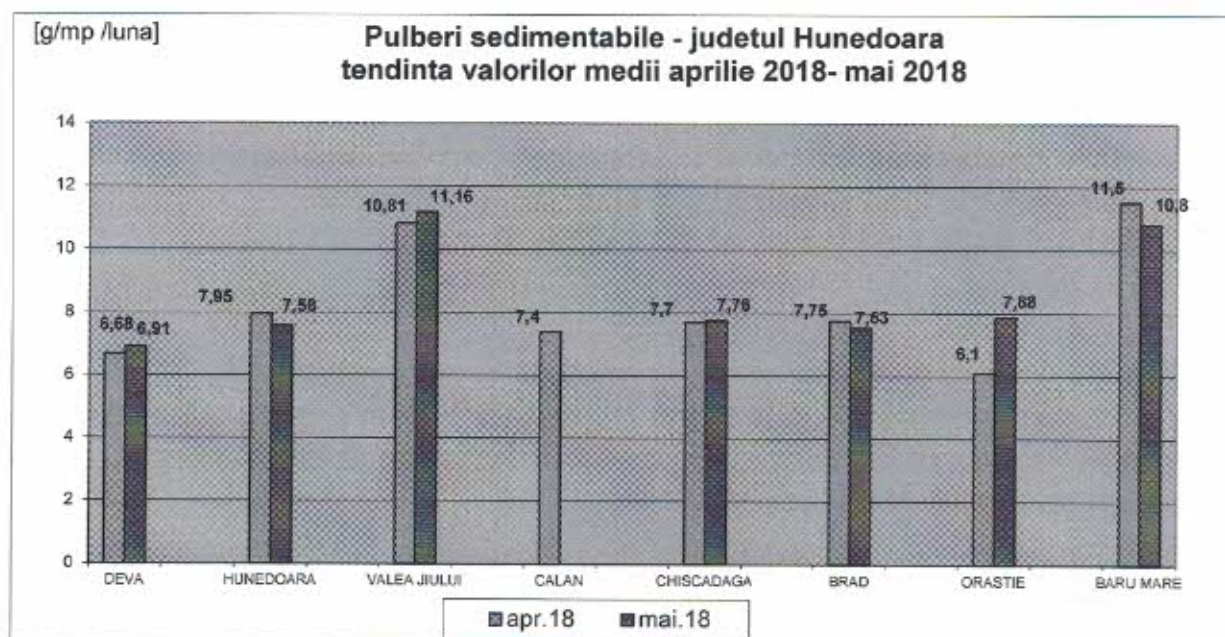
Fig. nr. 1.2.1.2. Evoluția calității pulberilor sedimentabile în perioada aprilie 2018 – mai 2018
