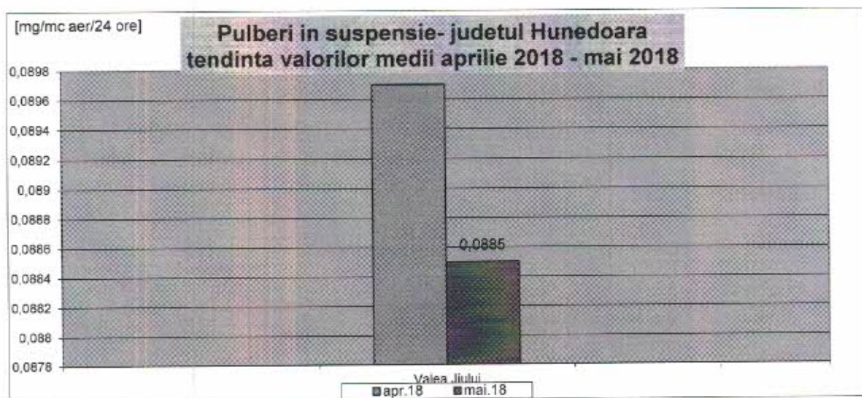
Fig. nr. 1.2.1.1. Evoluția calității pulberilor în suspensie în perioada aprilie 2018 – mai 2018
