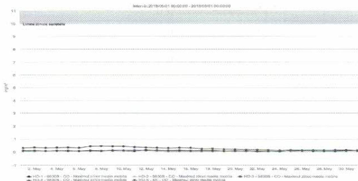
Figura nr. 1.3.5. Evoluția valorilor maxime zilnice a mediilor pe 8 ore la CO (mg/mc), în luna mai 2018, la stațiile automate de monitorizare
