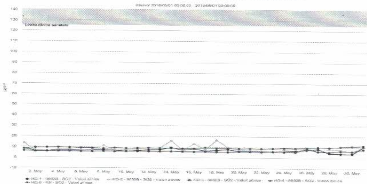
Figura nr. 1.3.3. Evoluția valorilor zilnice de SO 2 ( \mu\text{g}/\text{mc} ), în luna mai 2018, la stațiile automate de monitorizare
