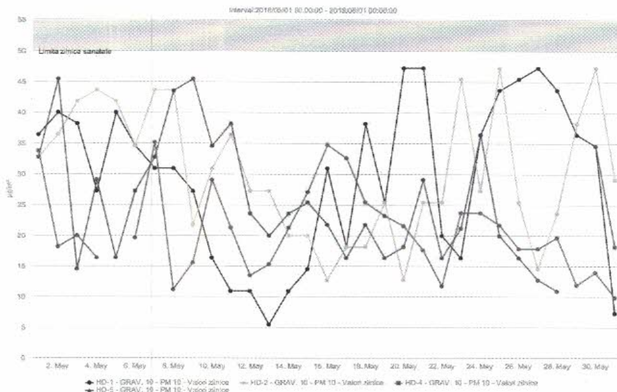
Figura nr. 1.3.7. Evoluția zilnică a valorilor de PM 10 ( \mu\text{g}/\text{mc} ) determinat gravimetric, în luna mai 2018, la stațiile automate de monitorizare
