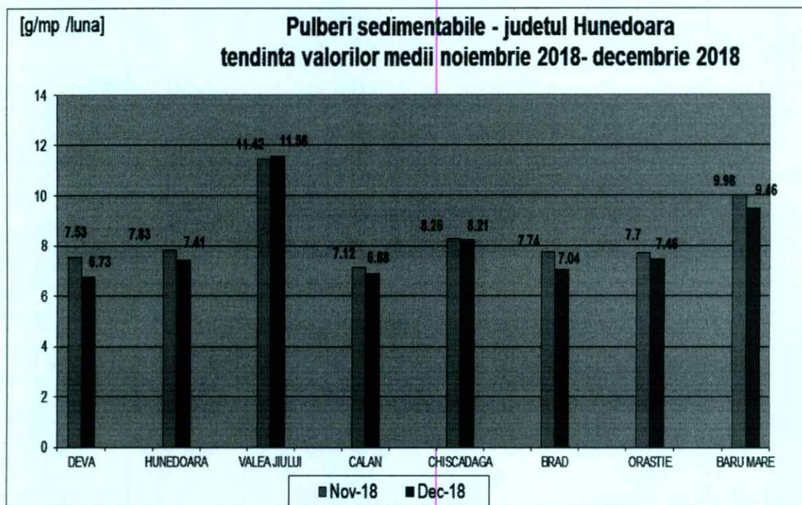
Fig. nr. 1.2.1.2. Evoluția calității pulberilor sedimentabile în perioada noiembrie 2018 – decembrie 2018
