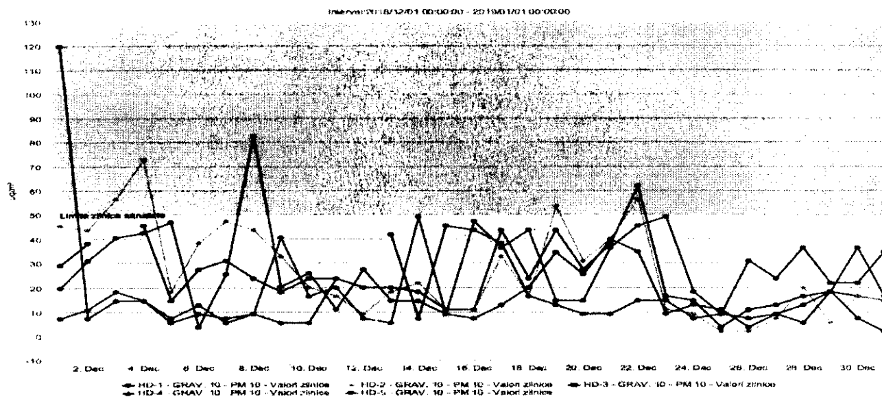
Figura nr. 1.3.7. Evoluția zilnică a valorilor de PM 10 (µg/mc) determinat gravimetric, în luna decembrie 2018, la stațiile automate de monitorizare
