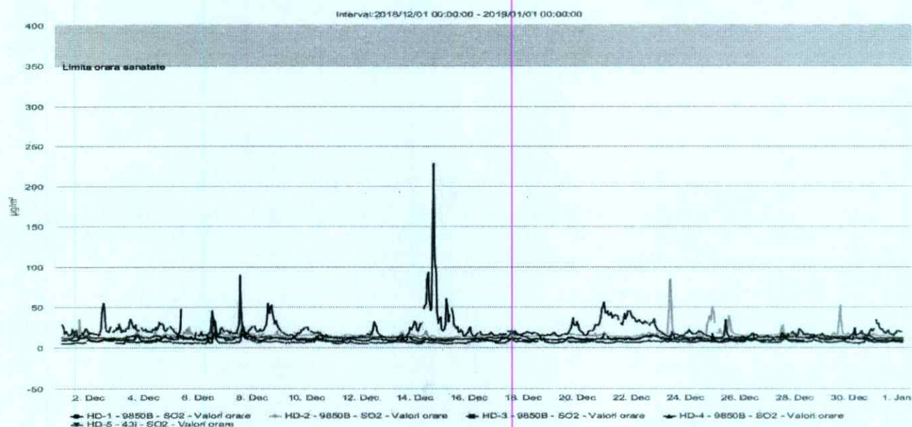
Figura nr. 1.3.2. Evoluția valorilor orare de SO 2 ( \mu\text{g}/\text{mc} ), în luna decembrie 2018 la stațiile automate de monitorizare
