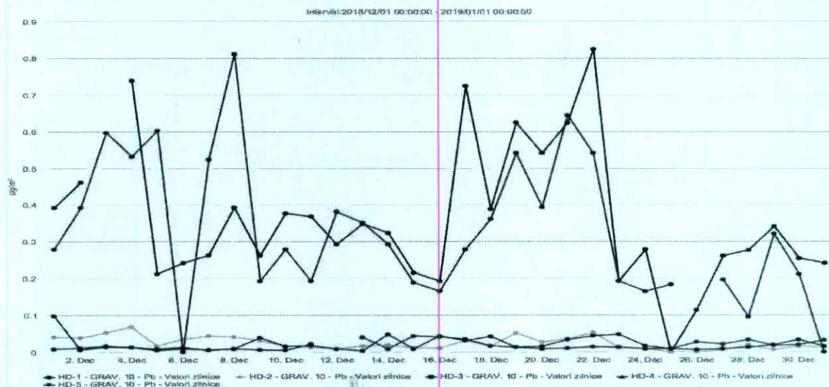
Figura nr. 1.3.8. Evoluția valorilor zilnice de Pb (μg/mc) din PM 10 gravimetric, în luna decembrie 2018, la stațiile automate de monitorizare
