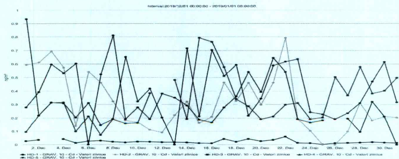
Figura nr. 1.3.9. Evoluția valorilor zilnice de Cd (μg/mc) din PM 10 gravimetric, în luna decembrie 2018, la stațiile automate de monitorizare
