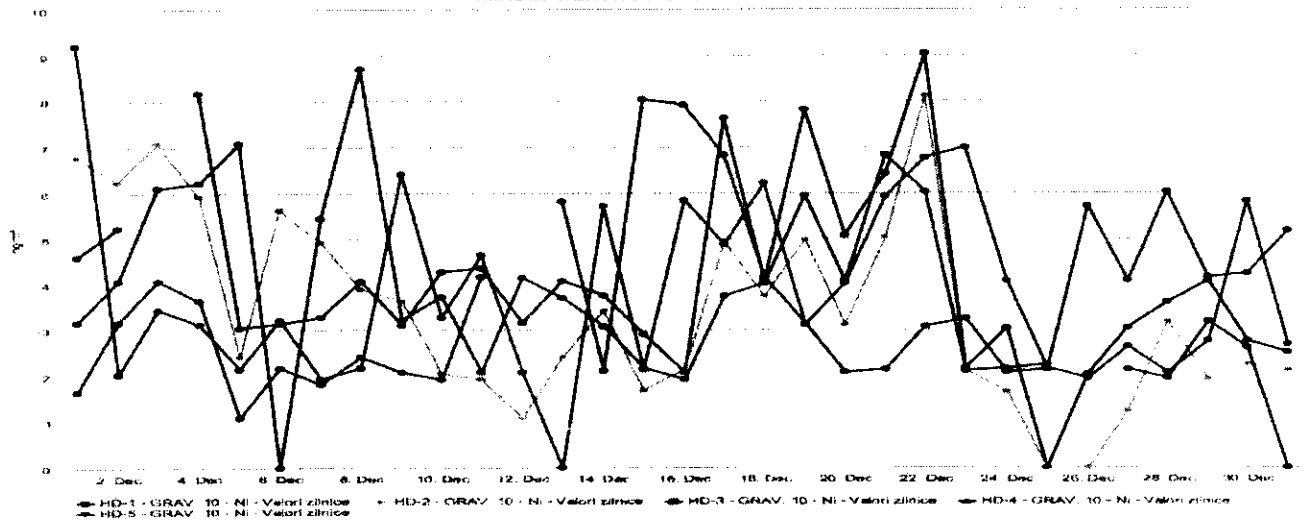
Figura nr.1.3.10. Evoluția valorilor zilnice de Ni ( \mu\text{g}/\text{mc} ) din \text{PM}_{10} gravimetric, în luna decembrie 2018, la stațiile automate de monitorizare
