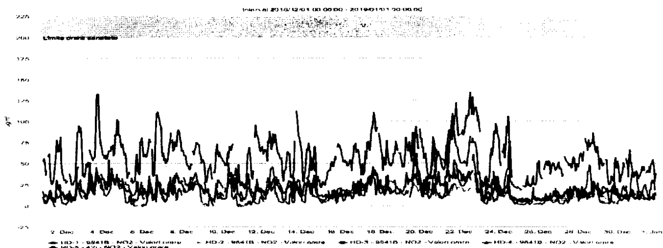
Figura nr. 1.3.4. Evoluția valorilor orare de NO 2 ( \mu\text{g}/\text{mc} ), în luna decembrie 2018, la stațiile automate de monitorizare
