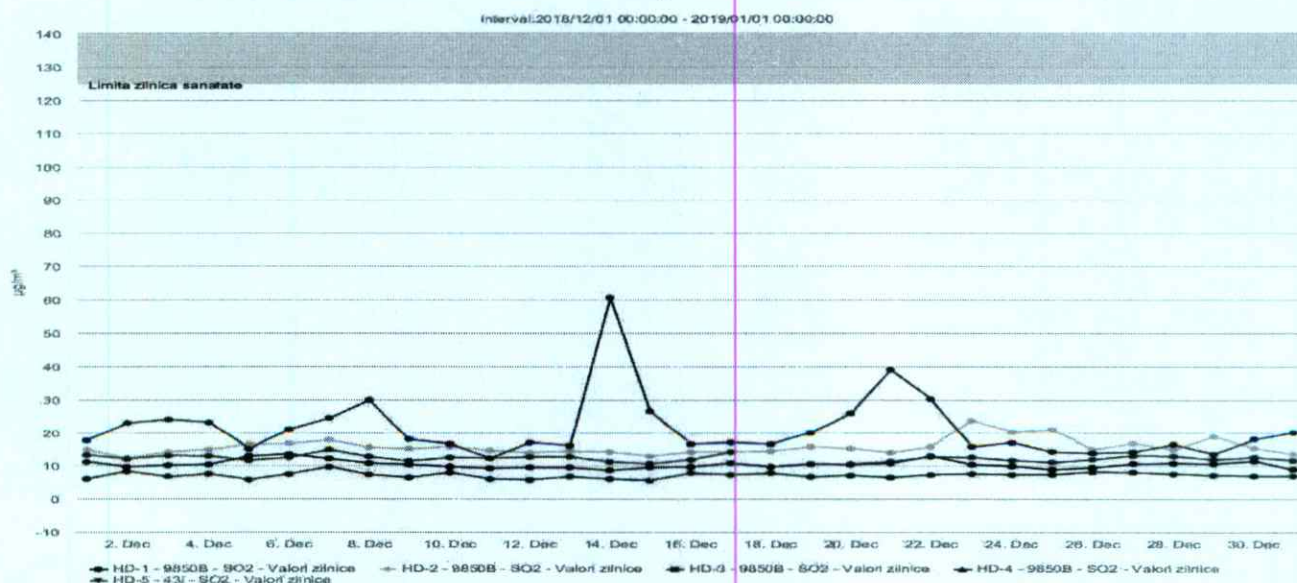
Figura nr. 1.3.3. Evoluția valorilor zilnice de SO 2 ( \mu\text{g}/\text{mc} ), în luna decembrie 2018, la stațiile automate de monitorizare
