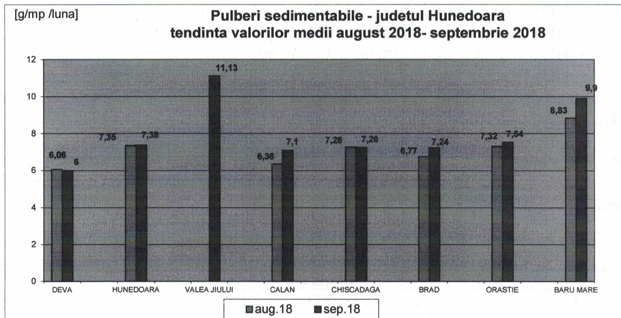
Fig. nr. 1.2.1.2. Evoluția calității pulberilor sedimentabile în perioada august 2018 – septembrie 2018
