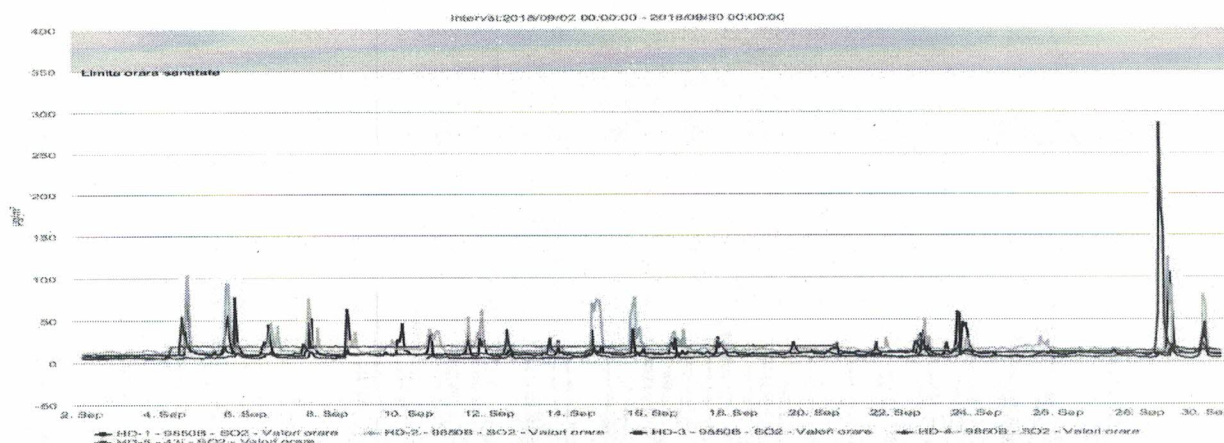
Figura nr. 1.3.2. Evoluția valorilor orare de SO 2 ( \mu\text{g}/\text{mc} ), în luna septembrie 2018 la stațiile automate de monitorizare
