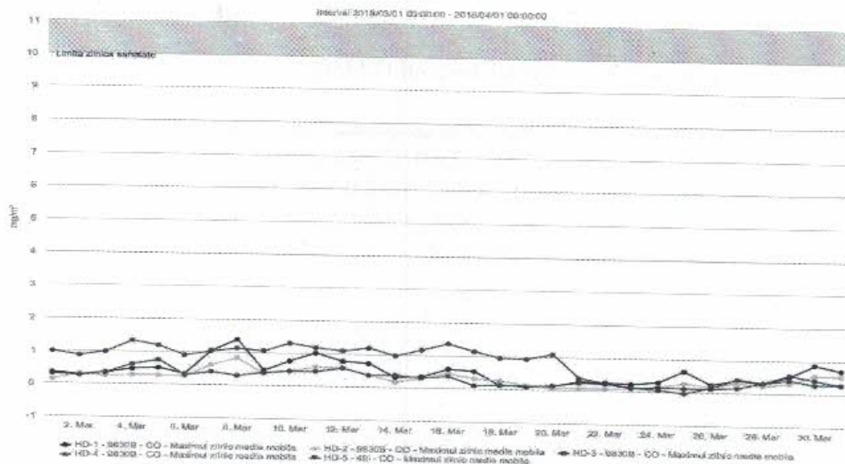
Figura nr. 1.3.5. Evoluția valorilor maxime zilnice a mediilor pe 8 ore la CO (mg/mc), în luna martie 2018, la stațiile automate de monitorizare
