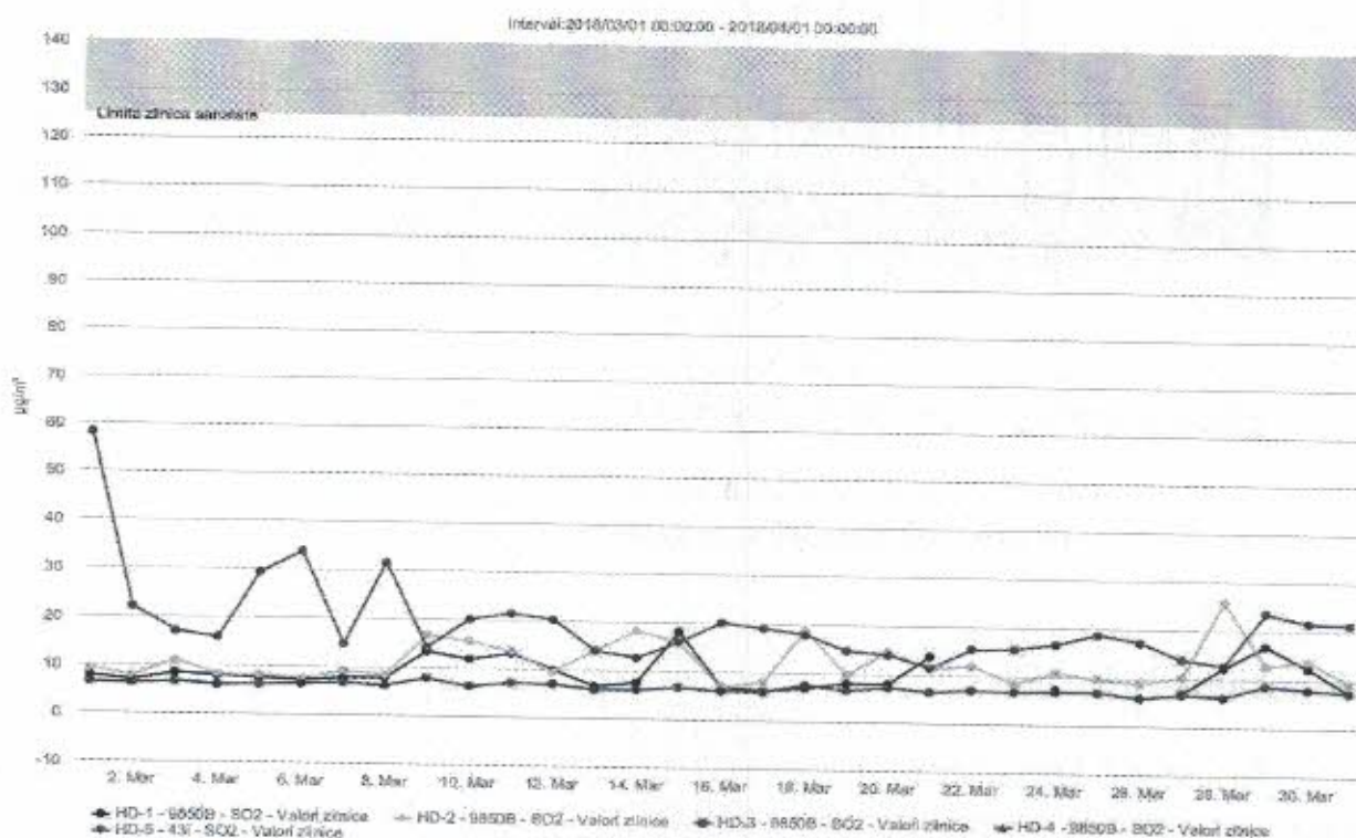
Figura nr. 1.3.3. Evoluția valorilor zilnice de SO 2 (µg/mc), în luna martie 2018, la stațiile automate de monitorizare
