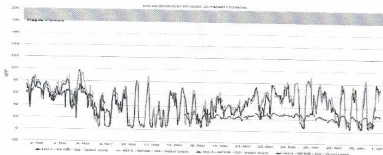
Figura nr. 1.3.6. Evoluția valorilor maxime zilnice a mediilor pe 8 ore la ozon ( \mu\text{g}/\text{mc} ), în luna martie 2018, la stațiile automate de monitorizare
