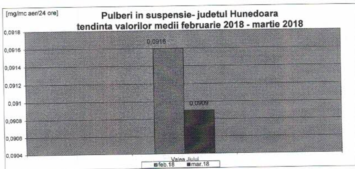
Fig. nr. 1.2.1.1. Evoluția calității pulberilor în suspensie în perioada februarie 2018 – martie 2018
