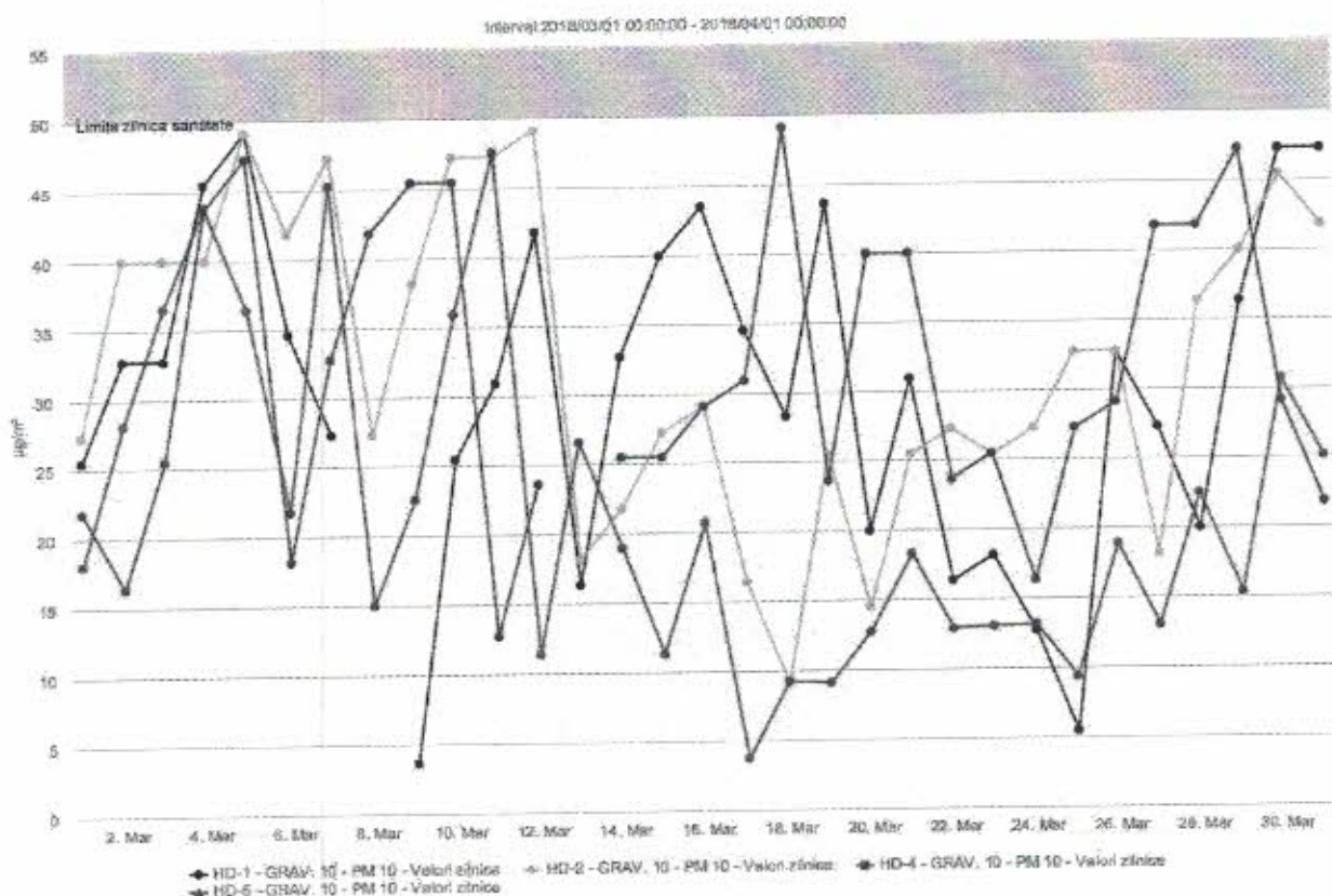
Figura nr. 1.3.7. Evoluția zilnică a valorilor de PM 10 ( \mu\text{g}/\text{mc} ) determinat gravimetric, în luna martie 2018, la stațiile automate de monitorizare
