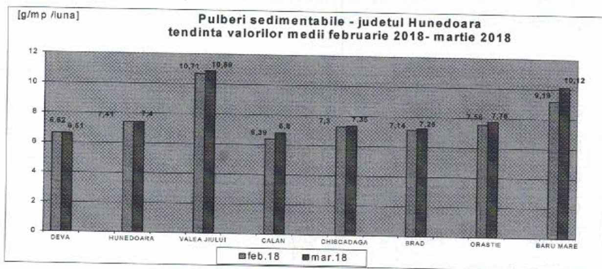
Fig. nr. 1.2.1.2. Evoluția calității pulberilor sedimentabile în perioada februarie 2018 – martie 2018
