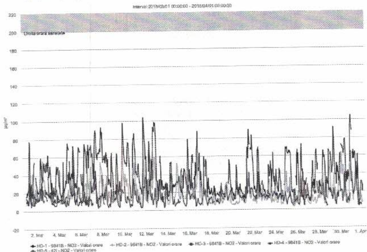
Figura nr. 1.3.4. Evoluția valorilor orare de NO 2 ( \mu\text{g}/\text{mc} ), în luna martie 2018, la stațiile automate de monitorizare
