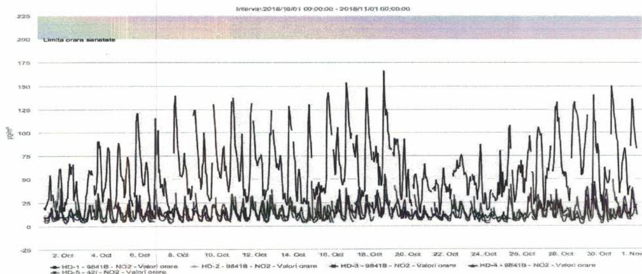
Figura nr. 1.3.4. Evoluția valorilor orare de NO 2 (µg/mc), în luna octombrie 2018, la stațiile automate de monitorizare
