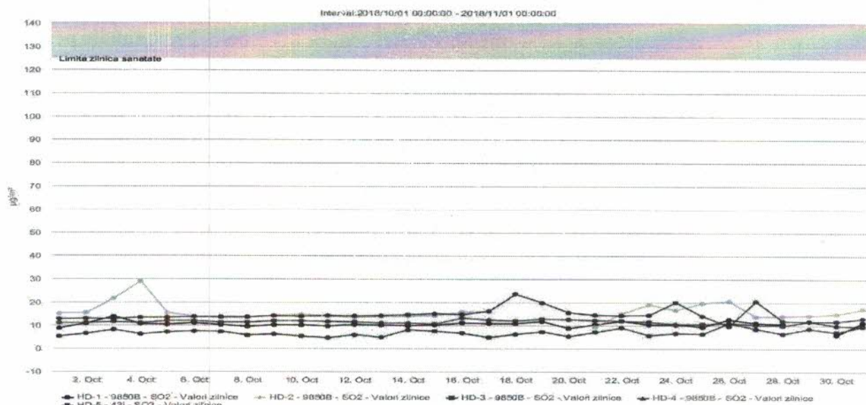
Figura nr. 1.3.3. Evoluția valorilor zilnice de SO 2 (µg/mc), în luna octombrie 2018, la stațiile automate de monitorizare
