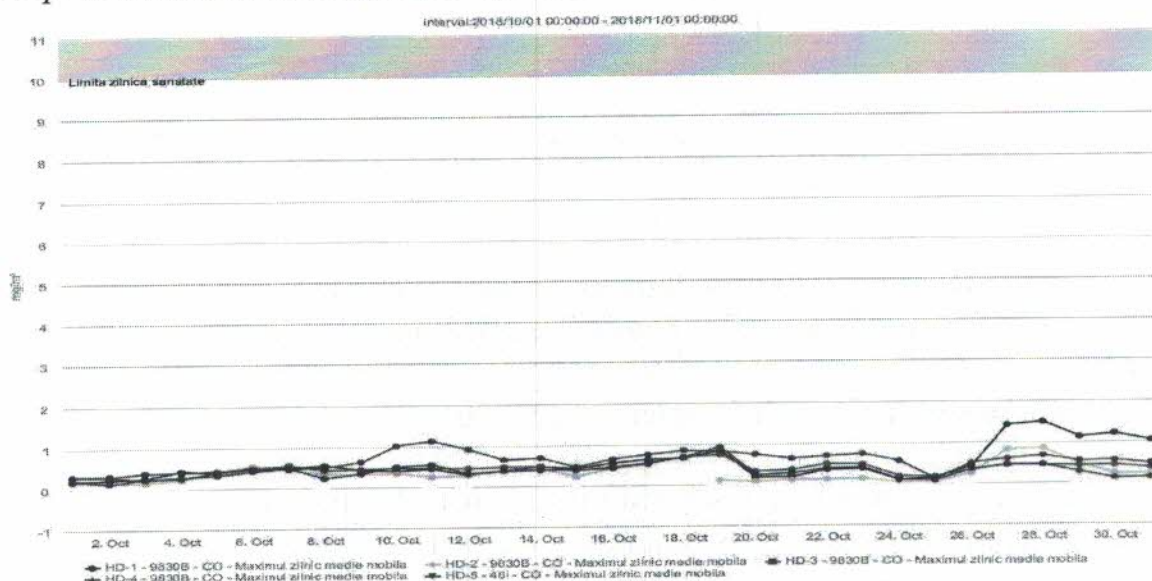
Figura nr. 1.3.5. Evoluția valorilor maxime zilnice a mediilor pe 8 ore la CO (mg/mc), în luna octombrie 2018, la stațiile automate de monitorizare
