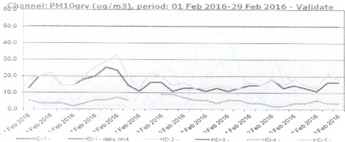
Figura nr. 1.3.7. Evoluția zilnică a valorilor de PM_{10} ( \mu\text{g}/\text{mc} ) determinat gravimetric, în luna februarie 2016, la stațiile automate de monitorizare
