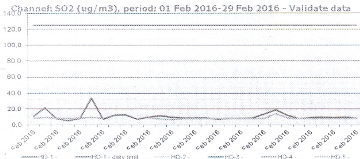
Figura nr. 1.3.3. Evoluția valorilor zilnice de SO 2 ( \mu\text{g}/\text{mc} ), în luna februarie 2016, la stațiile automate de monitorizare
