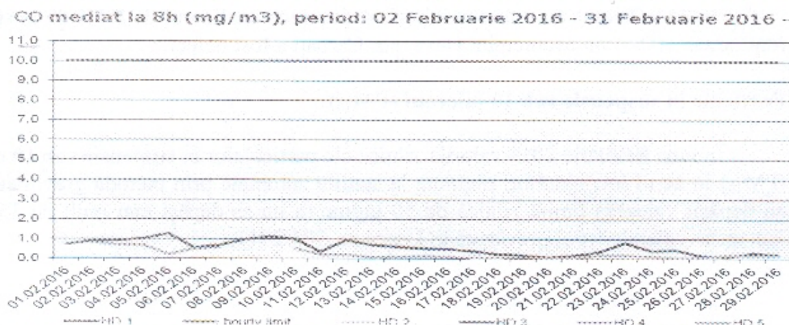
Figura nr. 1.3.5. Evoluția valorilor maxime zilnice a mediilor pe 8 ore la CO ( \text{mg}/\text{mc} ), în luna februarie 2016, la stațiile automate de monitorizare
