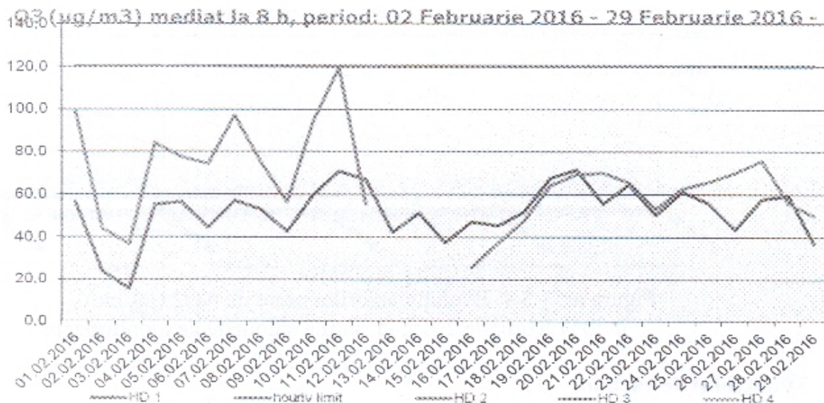
Figura nr. 1.3.6. Evoluția valorilor maxime zilnice a mediilor pe 8 ore la ozon ( \mu\text{g}/\text{mc} ), în luna februarie 2016, la stațiile automate de monitorizare
