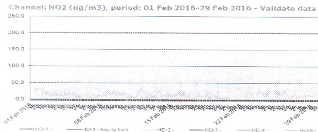
Figura nr. 1.3.4. Evoluția valorilor orare de NO 2 ( \mu\text{g}/\text{mc} ), în luna februarie 2016, la stațiile automate de monitorizare
