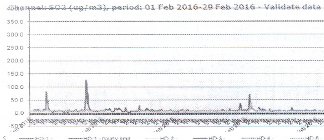
Figura nr. 1.3.2. Evoluția valorilor orare de SO 2 ( \mu\text{g}/\text{mc} ), în luna februarie 2016, la stațiile automate de monitorizare
