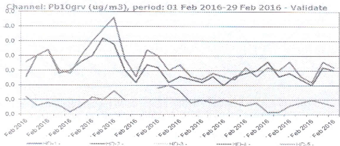
Figura nr. 1.3.8. Evoluția valorilor zilnice de Pb ( \mu\text{g}/\text{mc} ) din PM_{10} gravimetric, în luna februarie 2016, la stațiile automate de monitorizare
