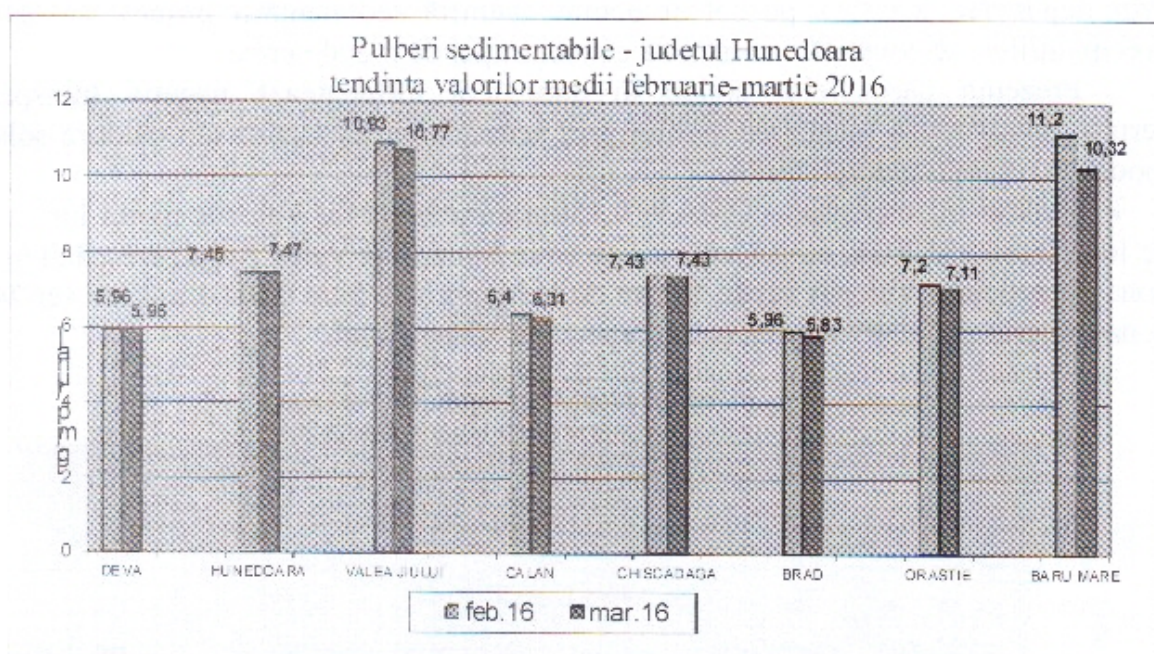
Fig. nr. 1.2.1.2. Evoluția calității pulberilor sedimentabile în perioada februarie – martie 2016
