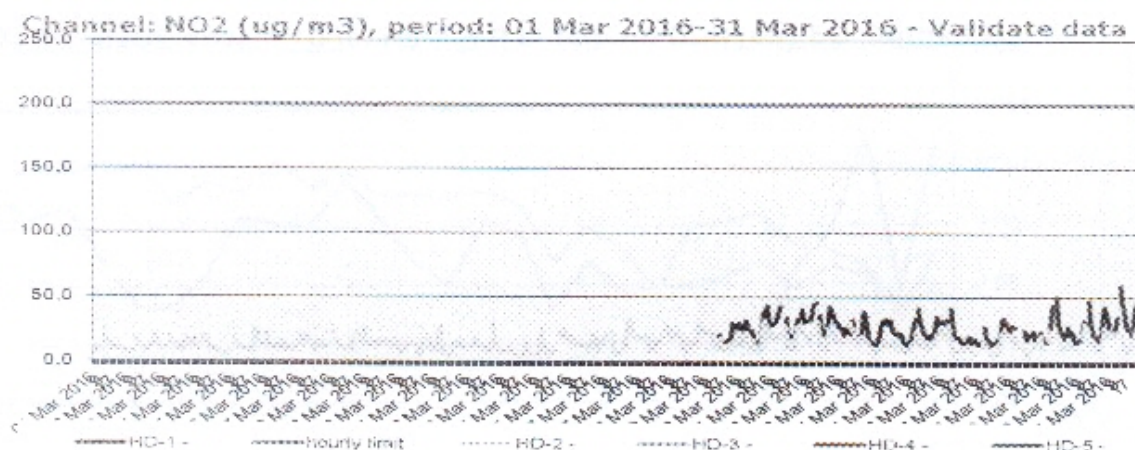
Figura nr. 1.3.4. Evoluția valorilor orare de NO 2 ( \mu\text{g}/\text{mc} ), în luna martie 2016, la stațiile automate de monitorizare
