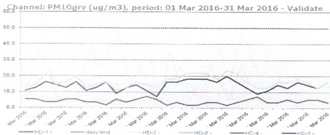
Figura nr. 1.3.7. Evoluția zilnică a valorilor de PM 10 (μg/mc) determinat gravimetric, în luna martie 2016, la stațiile automate de monitorizare
