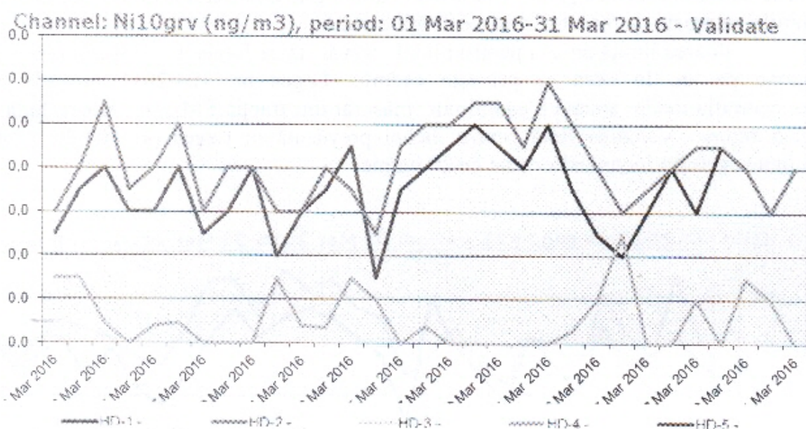
Figura nr.1.3.10. Evoluția valorilor zilnice de Ni ( \mu\text{g}/\text{m}^3 ) din \text{PM}_{10} gravimetric, în luna martie 2016, la stațiile automate de monitorizare
