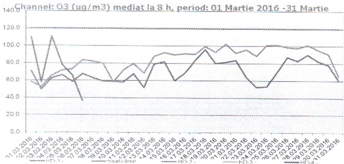
Figura nr. 1.3.6. Evoluția valorilor maxime zilnice a mediilor pe 8 ore la ozon ( \mu\text{g}/\text{mc} ), în luna martie 2016, la stațiile automate de monitorizare
