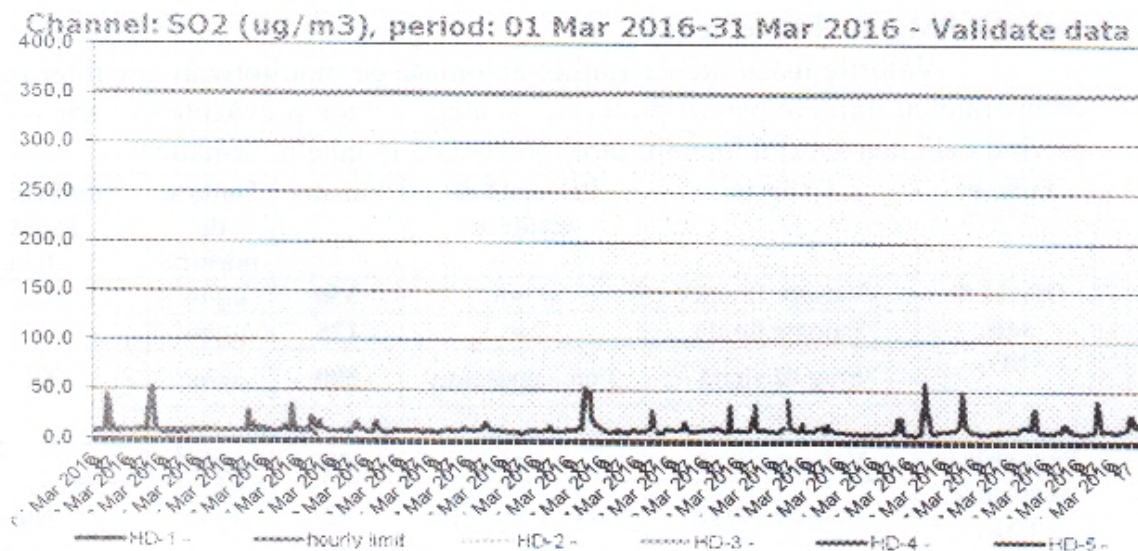
Figura nr. 1.3.2. Evoluția valorilor orare de SO2 ( \mu\text{g}/\text{mc} ), în luna martie 2016, la stațiile automate de monitorizare
