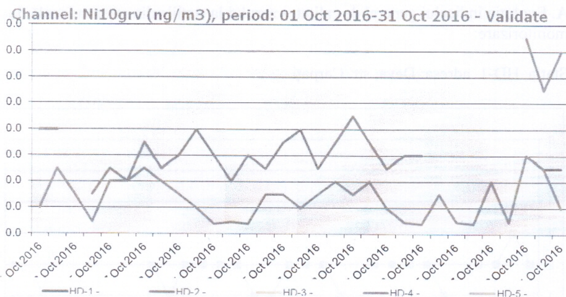
Figura nr.1.3.10. Evoluția valorilor zilnice de Ni ( \mu\text{g}/\text{mc} ) din \text{PM}_{10} gravimetric, în luna octombrie 2016, la stațiile automate de monitorizare
