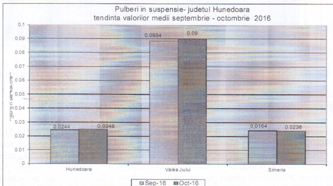
Fig. nr. 1.2.1.1. Evoluția calității pulberilor în suspensie în perioada septembrie – octombrie 2016
