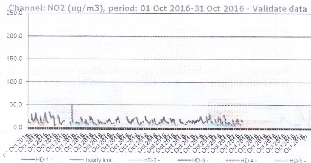
Figura nr. 1.3.4. Evoluția valorilor orare de NO 2 ( \mu\text{g}/\text{mc} ), în luna octombrie 2016, la stațiile automate de monitorizare
