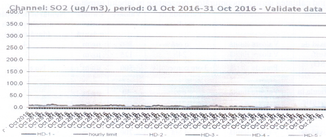
Figura nr. 1.3.2. Evoluția valorilor orare de SO2 ( \mu\text{g}/\text{mc} ), în luna octombrie 2016, la stațiile automate de monitorizare
