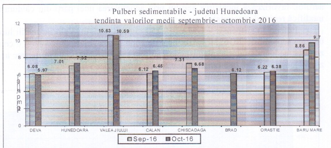
Fig. nr. 1.2.1.2. Evoluția calității pulberilor sedimentabile în perioada septembrie - octombrie 2016
