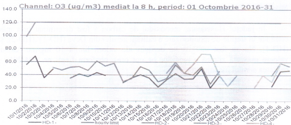
Figura nr. 1.3.6. Evoluția valorilor maxime zilnice a mediilor pe 8 ore la ozon ( \mu\text{g}/\text{mc} ), în luna octombrie 2016, la stațiile automate de monitorizare
