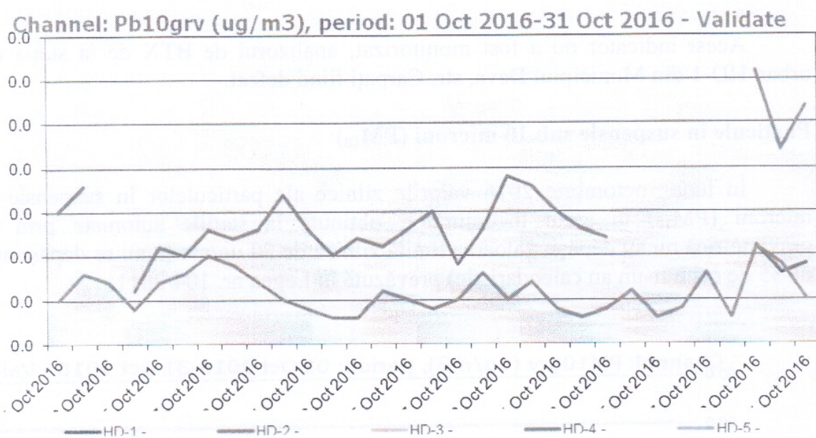
Figura nr. 1.3.8. Evoluția valorilor zilnice de Pb ( \mu\text{g}/\text{mc} ) din \text{PM}_{10} gravimetric, în luna octombrie 2016, la stațiile automate de monitorizare
