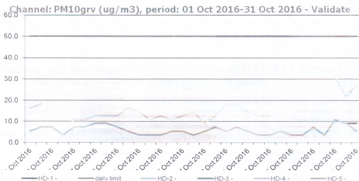
Figura nr. 1.3.7. Evoluția zilnică a valorilor de PM 10 (μg/mc) determinat gravimetric, în luna octombrie 2016, la stațiile automate de monitorizare
