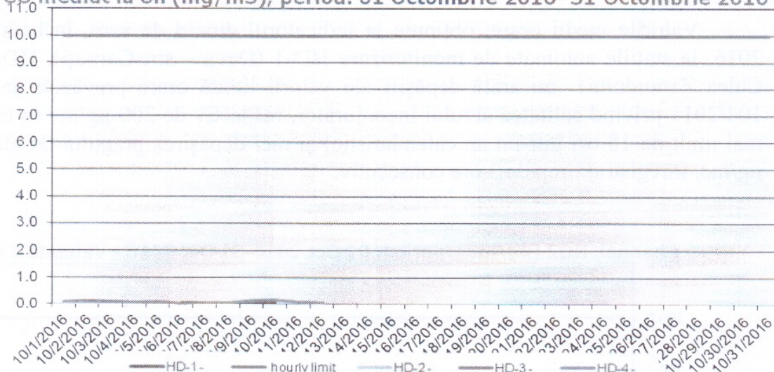
Figura nr. 1.3.5. Evoluția valorilor maxime zilnice a mediilor pe 8 ore la CO (mg/mc), în luna octombrie 2016, la stațiile automate de monitorizare
