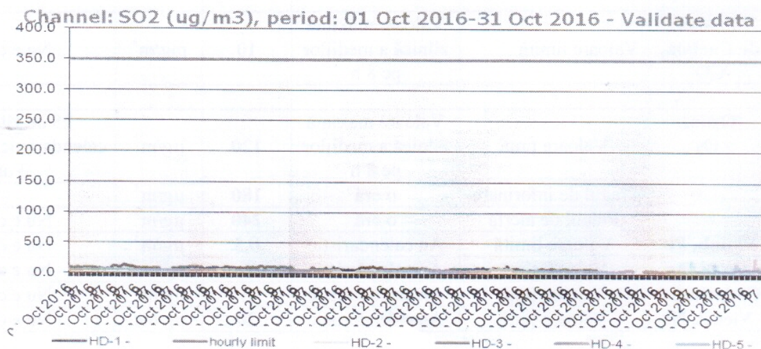
Figura nr. 1.3.3. Evoluția valorilor zilnice de SO2 ( \mu\text{g}/\text{mc} ), în luna octombrie 2016, la stațiile automate de monitorizare
