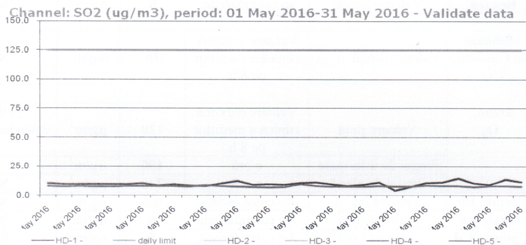
Figura nr. 1.3.3. Evoluția valorilor zilnice de SO 2 ( \mu\text{g}/\text{mc} ), în luna mai 2016, la stațiile automate de monitorizare
