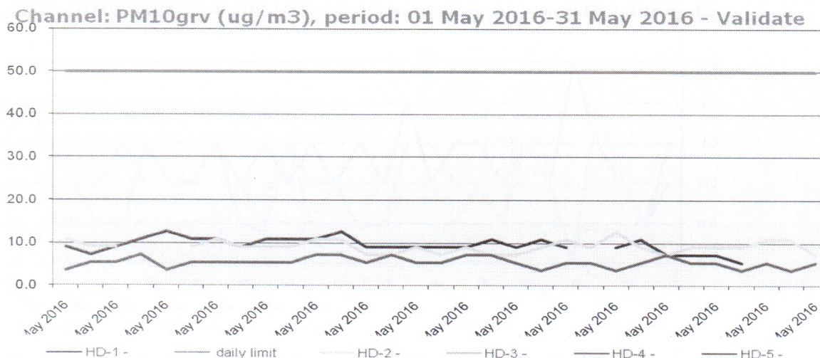
Figura nr. 1.3.7. Evoluția zilnică a valorilor de PM 10 (μg/mc) determinat gravimetric, în luna mai 2016, la stațiile automate de monitorizare
