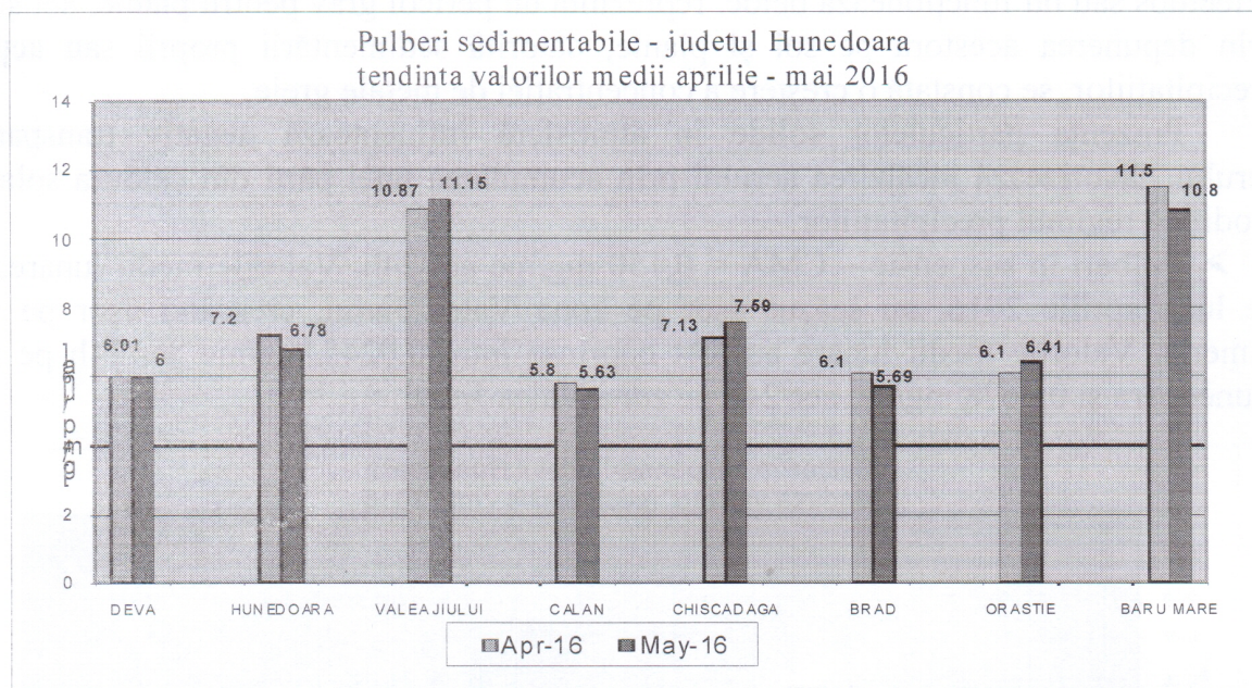
Fig. nr. 1.2.1.2. Evoluția calității pulberilor sedimentabile în perioada aprilie - mai 2016
