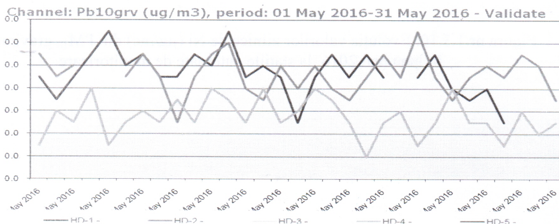
Figura nr. 1.3.8. Evoluția valorilor zilnice de Pb (μg/mc) din PM 10 gravimetric, în luna mai 2016, la stațiile automate de monitorizare
