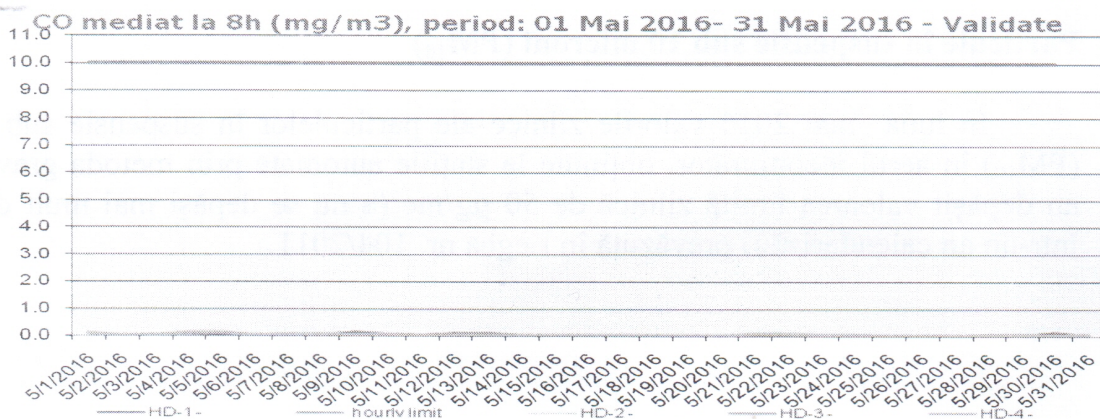
Figura nr. 1.3.5. Evoluția valorilor maxime zilnice a mediilor pe 8 ore la CO ( \text{mg}/\text{mc} ), în luna mai 2016, la stațiile automate de monitorizare
