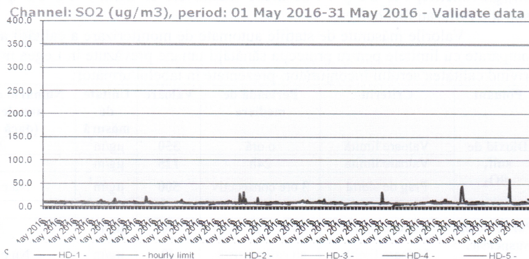
Figura nr. 1.3.2. Evoluția valorilor orare de SO 2 ( \mu\text{g}/\text{mc} ), în luna mai 2016, la stațiile automate de monitorizare
