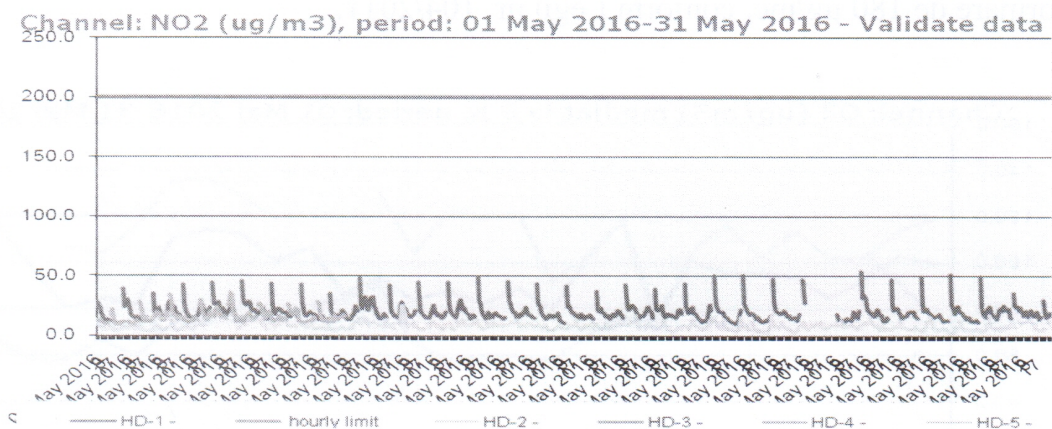
Figura nr. 1.3.4. Evoluția valorilor orare de NO2 ( \mu\text{g}/\text{mc} ), în luna mai 2016, la stațiile automate de monitorizare
