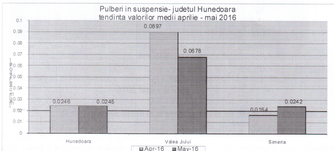
Fig. nr. 1.2.1.1. Evoluția calității pulberilor în suspensie în perioada aprilie – mai 2016
