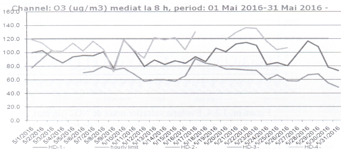
Figura nr. 1.3.6. Evoluția valorilor maxime zilnice a mediilor pe 8 ore la ozon ( \mu\text{g}/\text{mc} ), în luna mai 2016, la stațiile automate de monitorizare
