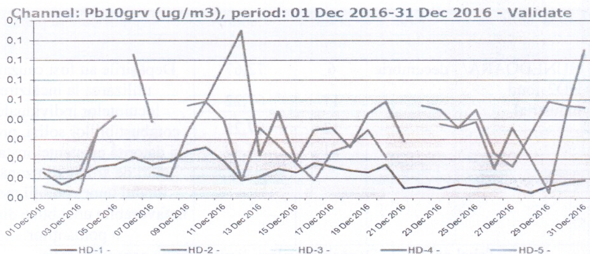
Figura nr. 1.3.8. Evoluția valorilor zilnice de Pb ( \mu\text{g}/\text{mc} ) din PM_{10} gravimetric, în luna decembrie 2016, la stațiile automate de monitorizare
