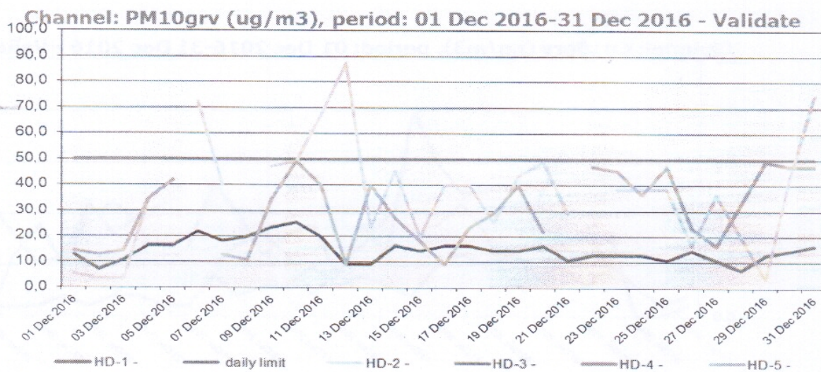
Figura nr. 1.3.7. Evoluția zilnică a valorilor de PM 10 (μg/mc) determinat gravimetric, în luna decembrie 2016, la stațiile automate de monitorizare
