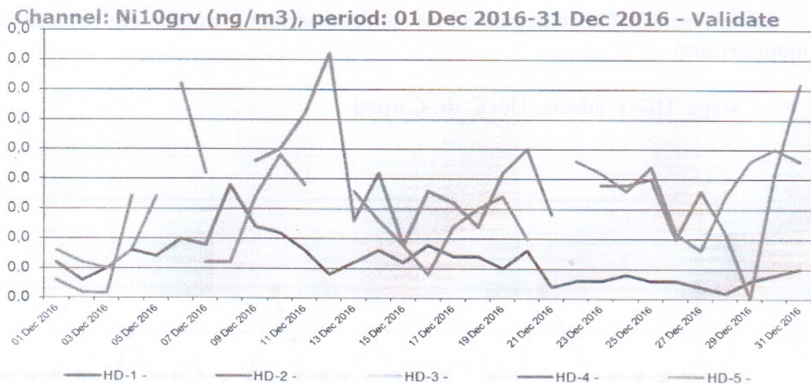
Figura nr.1.3.10. Evoluția valorilor zilnice de Ni ( \mu\text{g}/\text{mc} ) din \text{PM}_{10} gravimetric, în luna decembrie 2016, la stațiile automate de monitorizare
