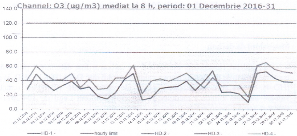
Figura nr. 1.3.6. Evoluția valorilor maxime zilnice a mediilor pe 8 ore la ozon ( \mu\text{g}/\text{mc} ), în luna decembrie 2016, la stațiile automate de monitorizare
