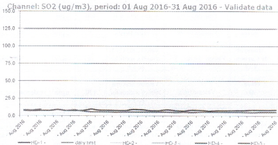
Figura nr. 1.3.3. Evoluția valorilor zilnice de SO 2 ( \mu\text{g}/\text{m}^3 ), în luna august 2016, la stațiile automate de monitorizare
