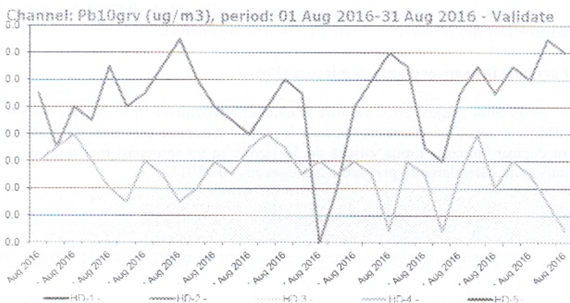
Figura nr. 1.3.8. Evoluția valorilor zilnice de Pb ( \mu\text{g}/\text{mc} ) din \text{PM}_{10} gravimetric, în luna august 2016, la stațiile automate de monitorizare
