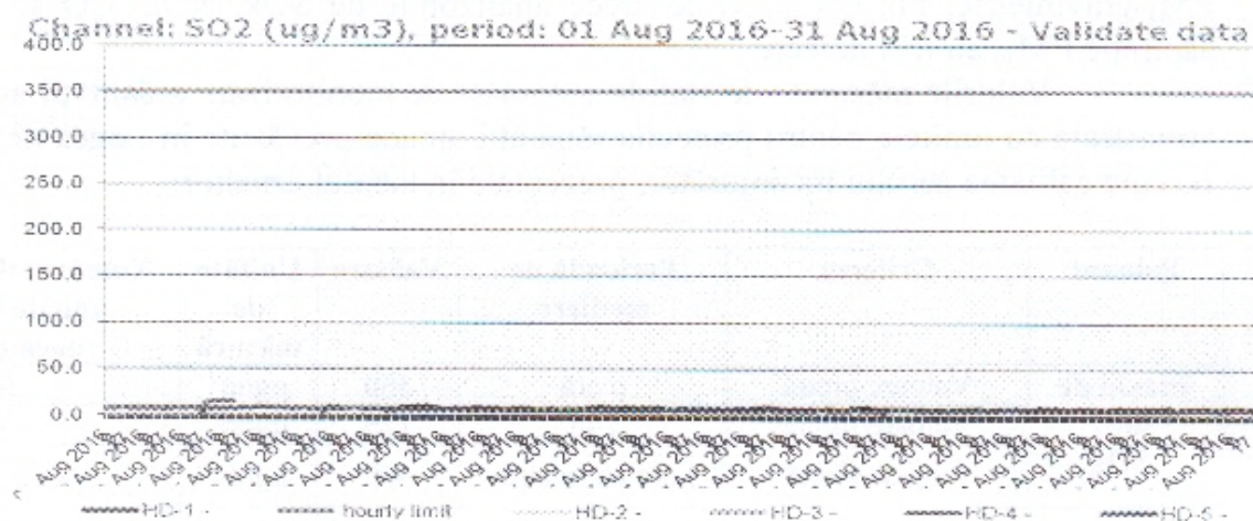
Figura nr. 1.3.2. Evoluția valorilor orare de SO 2 ( \mu\text{g}/\text{m}^3 ), în luna august 2016, la stațiile automate de monitorizare
