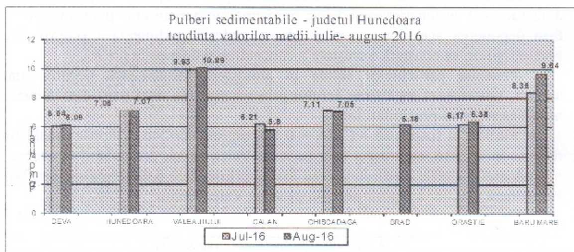
Fig. nr. 1.2.1.2. Evoluția calității pulberilor sedimentabile în perioada iulie - august 2016
