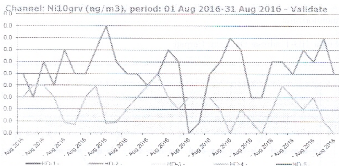
Figura nr.1.3.10. Evoluția valorilor zilnice de Ni ( \mu\text{g}/\text{mc} ) din \text{PM}_{10} gravimetric, în luna august 2016, la stațiile automate de monitorizare
