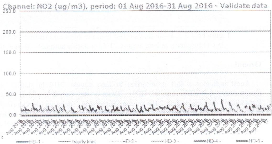
Figura nr. 1.3.4. Evoluția valorilor orare de NO 2 ( \mu\text{g}/\text{mc} ), în luna august 2016, la stațiile automate de monitorizare
