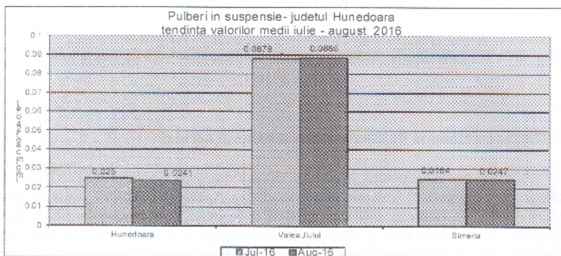
Fig. nr. 1.2.1.1. Evoluția calității pulberilor în suspensie în perioada iulie – august 2016
