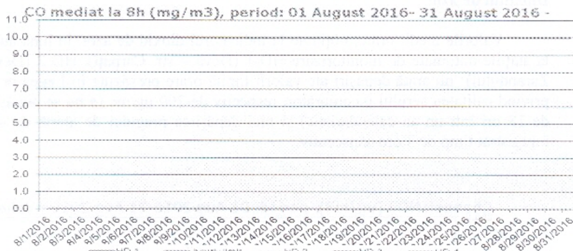
Figura nr. 1.3.5. Evoluția valorilor maxime zilnice a mediilor pe 8 ore la CO (mg/mc), în luna august 2016, la stațiile automate de monitorizare
