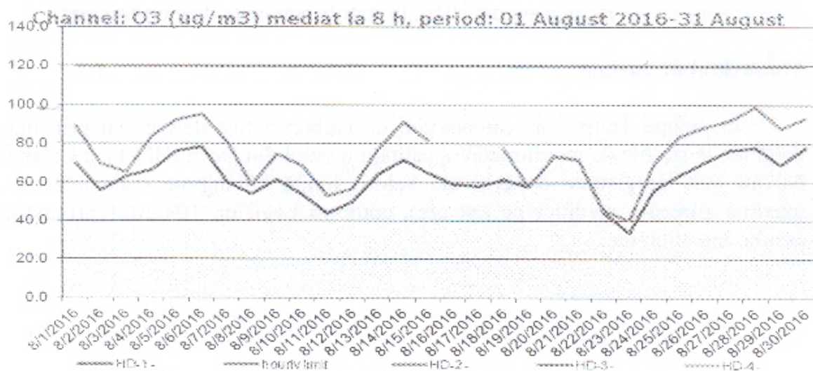
Figura nr. 1.3.6. Evoluția valorilor maxime zilnice a mediilor pe 8 ore la ozon ( \mu\text{g}/\text{mc} ), în luna august 2016, la stațiile automate de monitorizare
