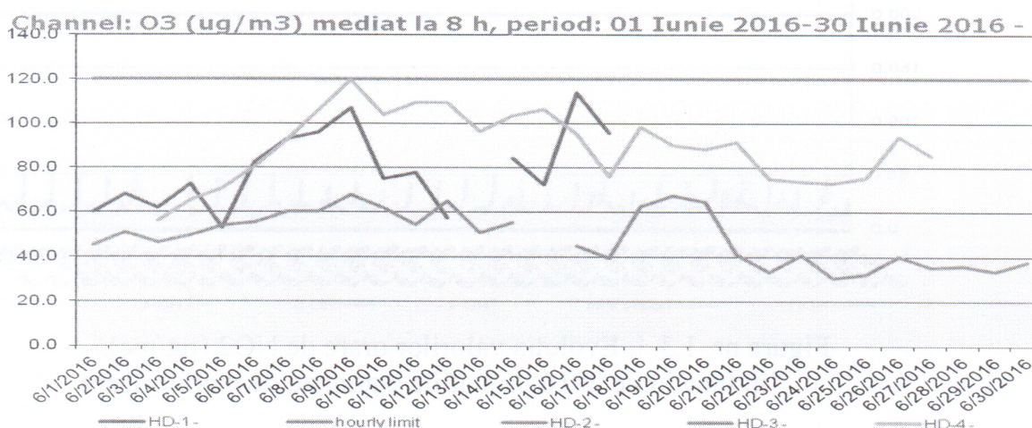
Figura nr. 1.3.6. Evoluția valorilor maxime zilnice a mediilor pe 8 ore la ozon ( \mu\text{g}/\text{mc} ), în luna iunie 2016, la stațiile automate de monitorizare
