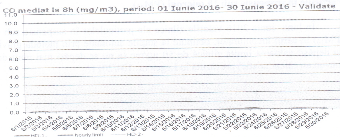
Figura nr. 1.3.5. Evoluția valorilor maxime zilnice a mediilor pe 8 ore la CO ( \text{mg}/\text{mc} ), în luna iunie 2016, la stațiile automate de monitorizare
