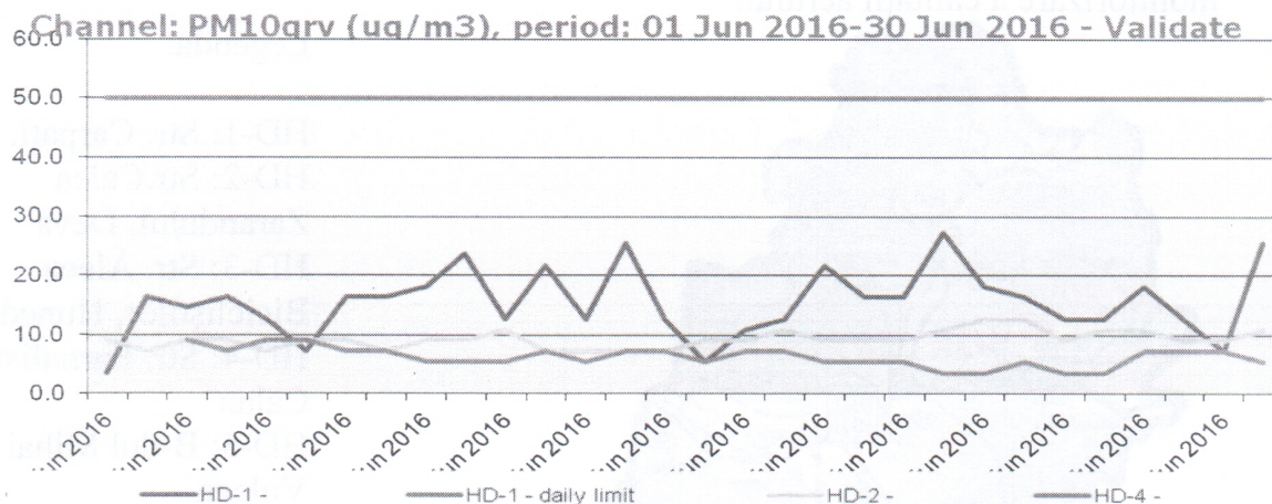
Figura nr. 1.3.7. Evoluția zilnică a valorilor de PM_{10} ( \mu\text{g}/\text{mc} ) determinat gravimetric, în luna iunie 2016, la stațiile automate de monitorizare
