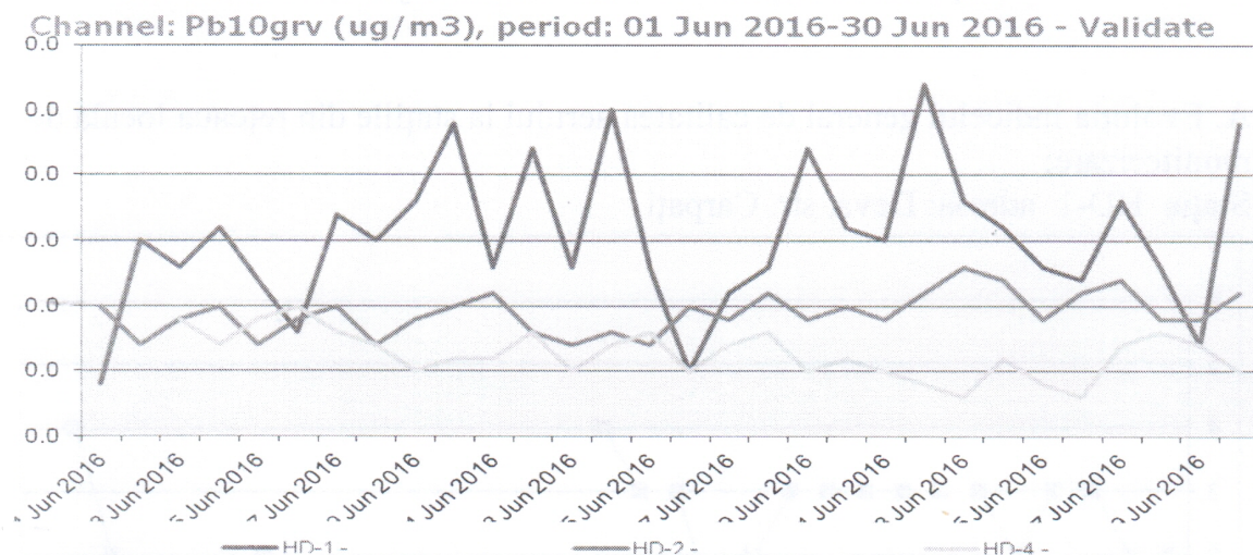
Figura nr. 1.3.8. Evoluția valorilor zilnice de Pb ( \mu\text{g}/\text{mc} ) din PM_{10} gravimetric, în luna iunie 2016, la stațiile automate de monitorizare
