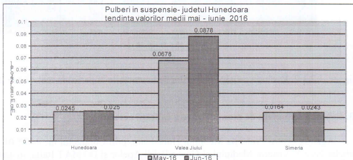
Fig. nr. 1.2.1.1. Evoluția calității pulberilor în suspensie în perioada mai – iunie 2016
