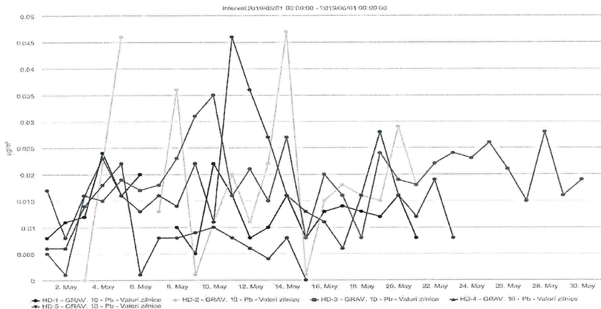
Figura nr. 1.3.8. Evoluția valorilor zilnice de Pb ( \mu\text{g}/\text{mc} ) din \text{PM}_{10} gravimetric, în luna mai 2019, la stațiile automate de monitorizare
