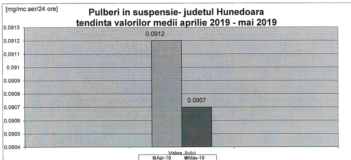
Fig. nr. 1.2.1.1. Evoluția calității pulberilor în suspensie în perioada aprilie 2019 – mai 2019
