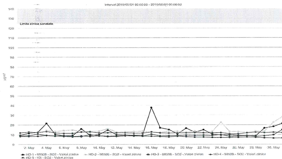
Figura nr. 1.3.3. Evoluția valorilor zilnice de SO 2 (µg/mc), în luna mai 2019, la stațiile automate de monitorizare
