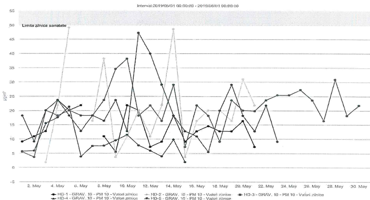
Figura nr. 1.3.7. Evoluția zilnică a valorilor de PM 10 ( \mu\text{g}/\text{mc} ) determinat gravimetric, în luna mai 2019, la stațiile automate de monitorizare
