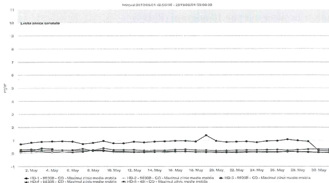
Figura nr. 1.3.5. Evoluția valorilor maxime zilnice a mediilor pe 8 ore la CO (mg/mc), în luna mai 2019, la stațiile automate de monitorizare
