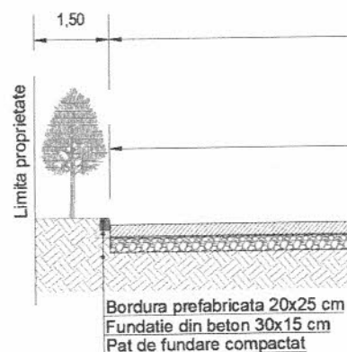
fig.2 Detaliu alcătuire
