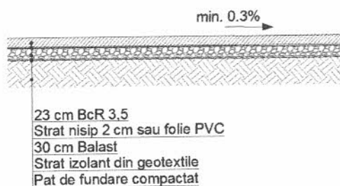
fig.1 Detaliu alcătuire
