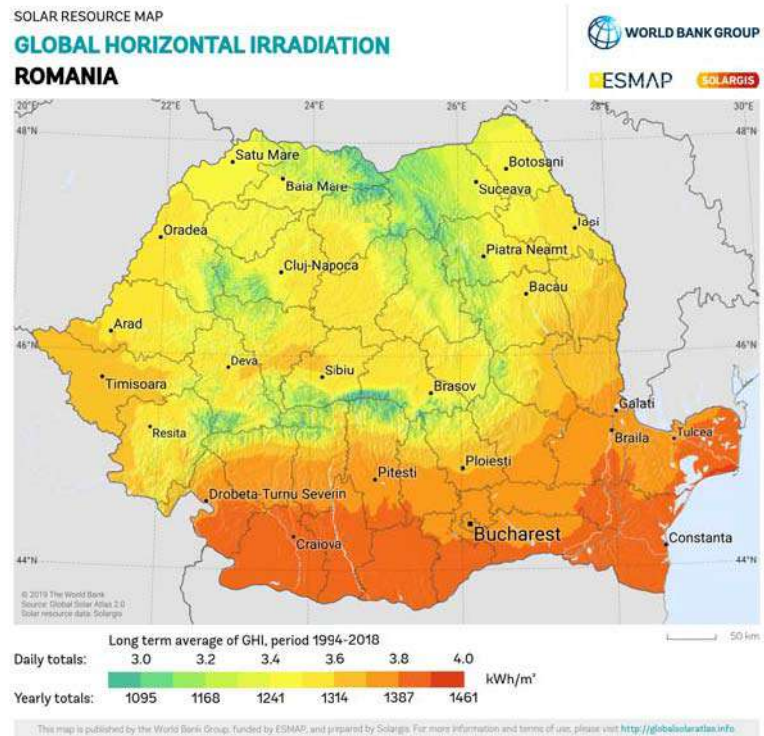
Figura 1 – Radiația globală pe suprafață orizontală (sursa: https://solargis.com/ )
