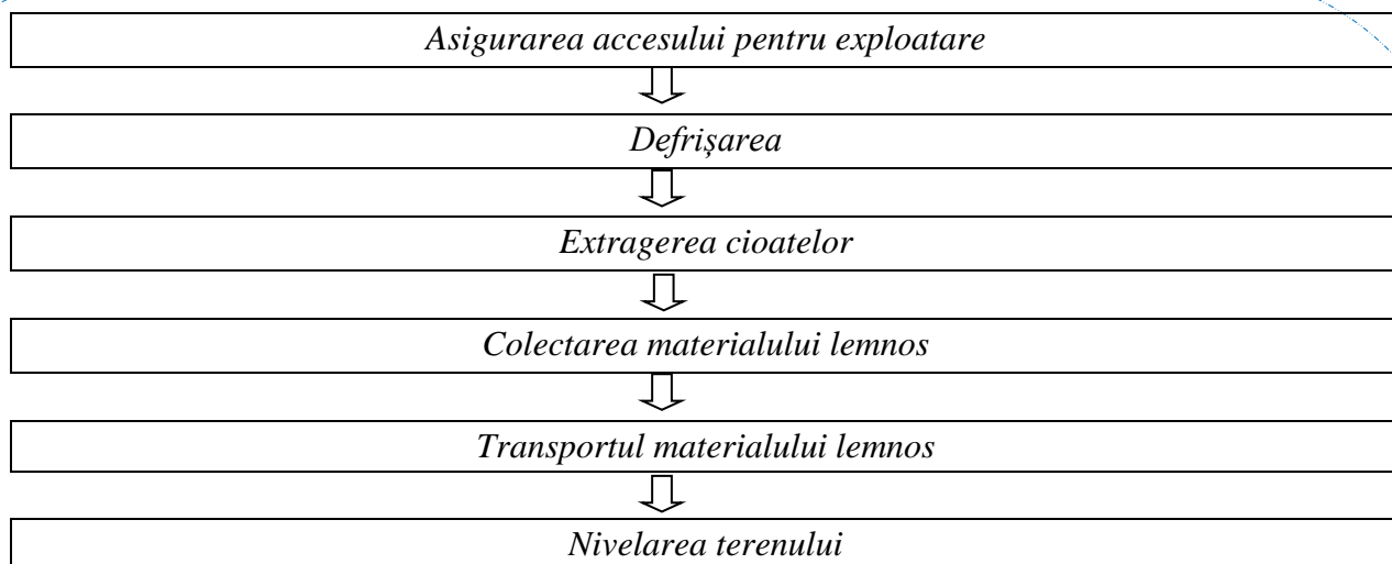
Fig. 2.1 Schema procesului tehnologic
