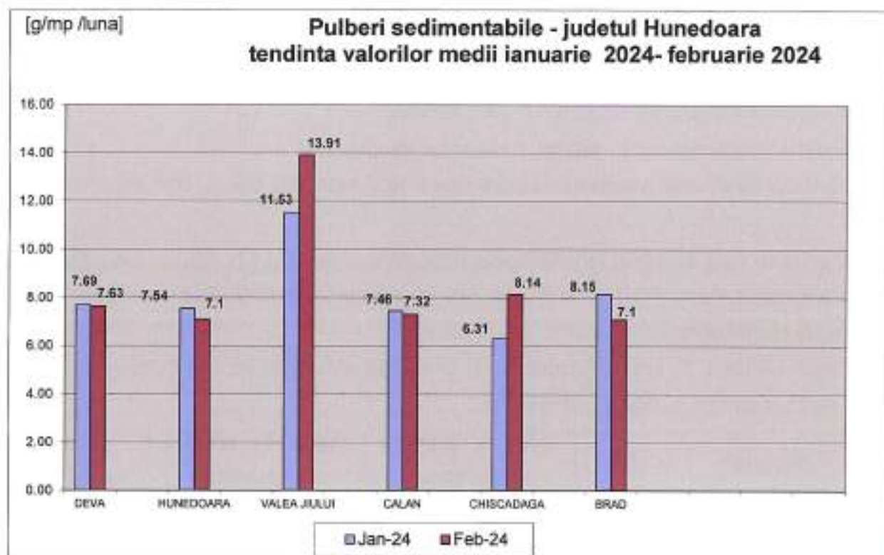
Fig. nr. 1.2.1.1. Evoluția calității pulberilor sedimentabile în perioada ianuarie 2024 - februarie 2024
