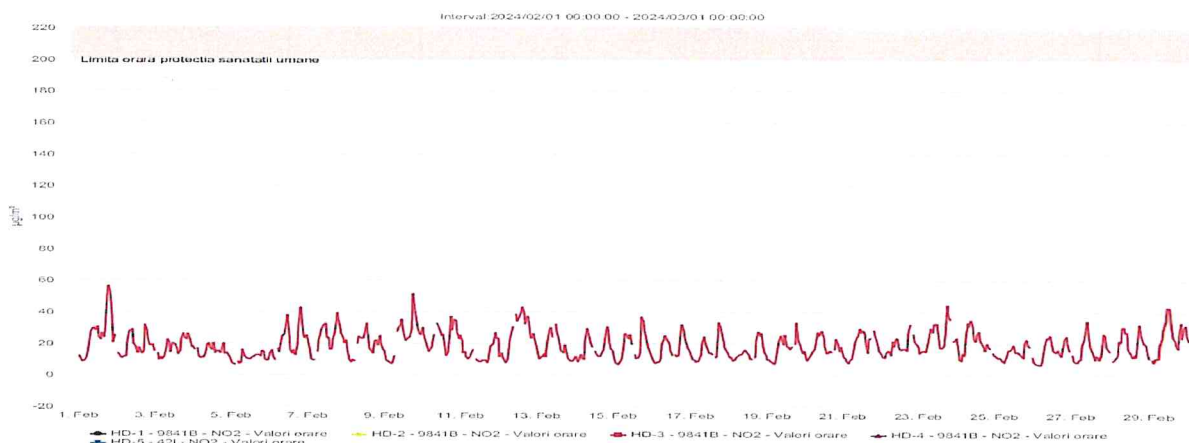
Figura nr. 1.3.4. Evoluția valorilor orare de NO2 ( \mu\text{g}/\text{mc} ), în luna februarie 2024, la stațiile automate de monitorizare
