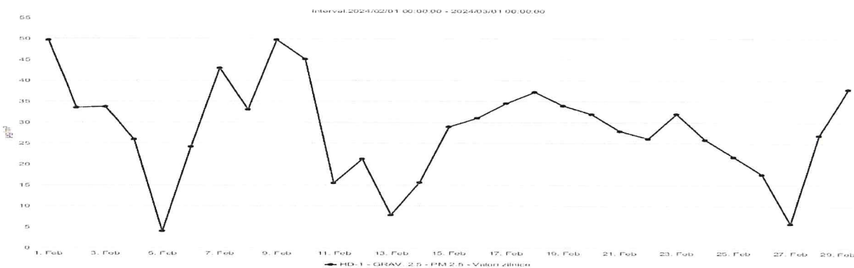
Figura nr. 1.3.8. Evoluția zilnică a valorilor de PM_{2.5} ( \mu\text{g}/\text{mc} ) determinat gravimetric, în luna februarie 2024, la stația automata de monitorizare HD-1
