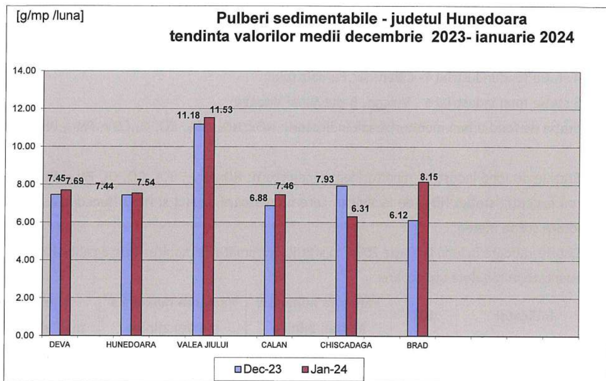
Fig. nr. 1.2.1.1. Evoluția calității pulberilor sedimentabile în perioada decembrie 2023 - ianuarie 2024
