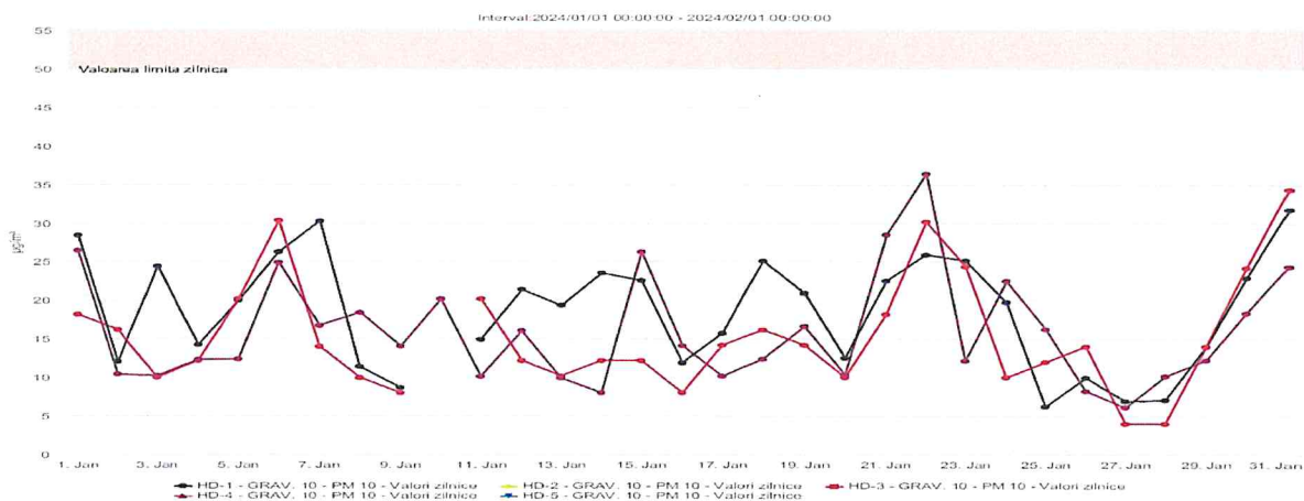
Figura nr. 1.3.8. Evoluția zilnică a valorilor de PM 10 (µg/mc) determinat gravimetric, în luna ianuarie 2024, la stațiile automate de monitorizare
