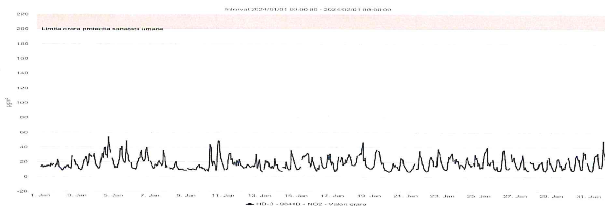
Figura nr. 1.3.4. Evoluția valorilor orare de NO 2 (µg/mc), în luna ianuarie 2024, la stațiile automate de monitorizare
