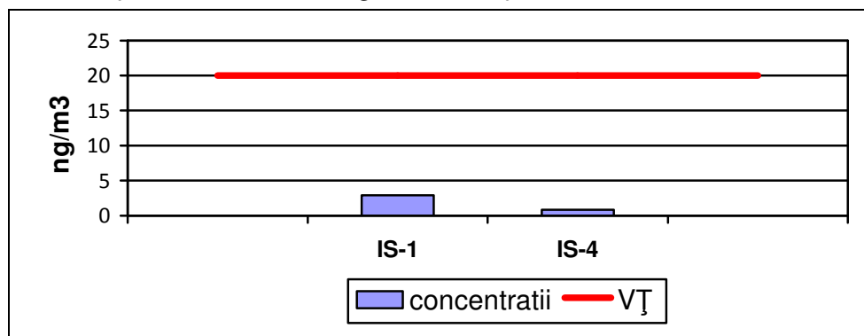
Figura I.3.4.3. Ni gravimetric determinat din fracția PM10 – Concentrațiile medii anuale înregistrate la stațiile de monitorizare, în anul 2015
