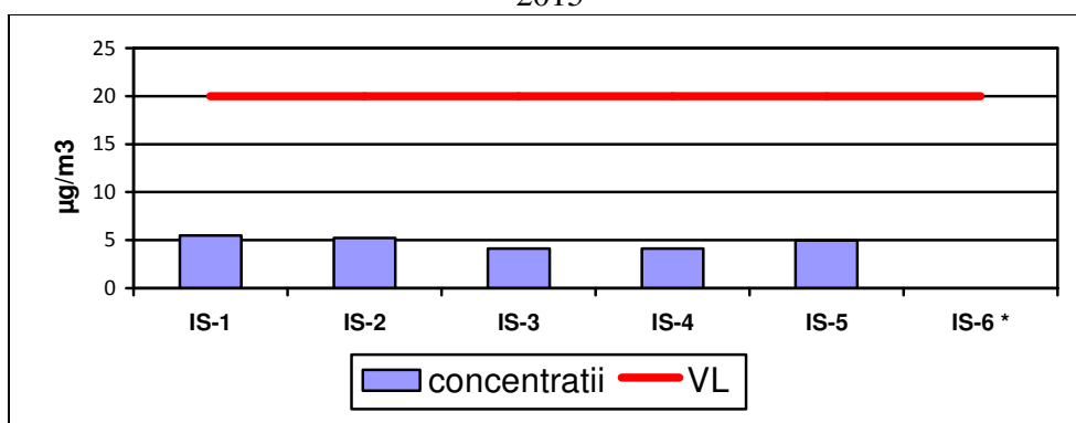
Figura I.3.2.2 SO 2 - Concentrațiile medii anuale înregistrate la stațiile de monitorizare, în anul 2015
