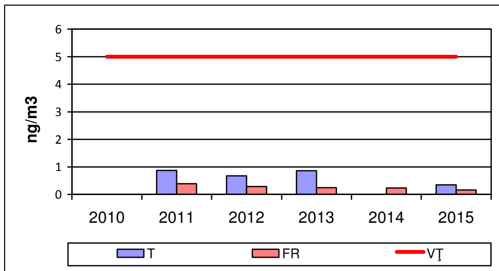
Figura I.I.7. Cd gravimetric determinat din fracția PM10 – Evoluția concentrațiilor medii anuale înregistrate la stațiile de monitorizare în raport cu VL anuală, în perioada 2010 – 2015
