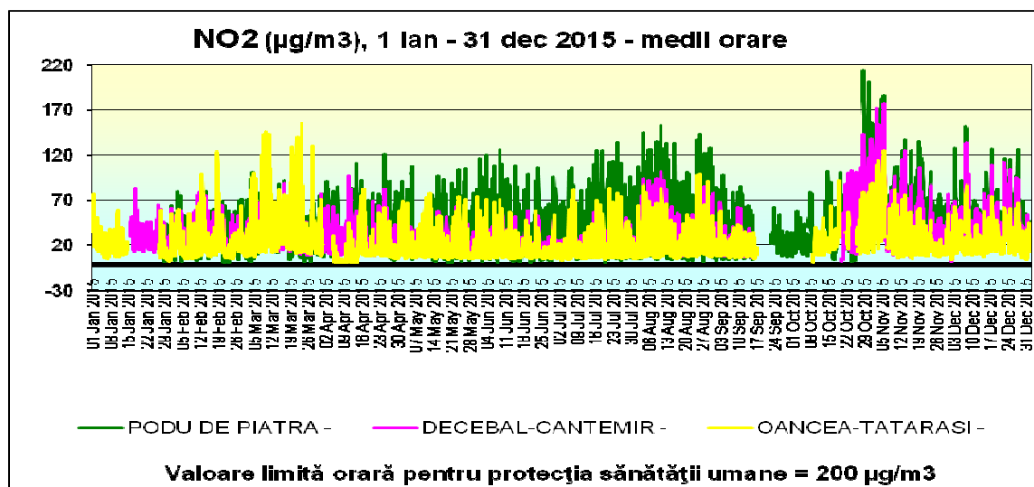
Figura I.3.1.1. Variația mediilor orare ale dioxidului de azot (NO 2 ) în anul 2015
