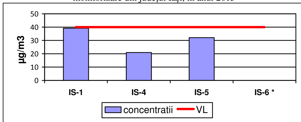
Figura I.3.3.1. PM10 gravimetric - Concentrațiile medii anuale înregistrate la stațiile de monitorizare din județul Iași, în anul 2015
