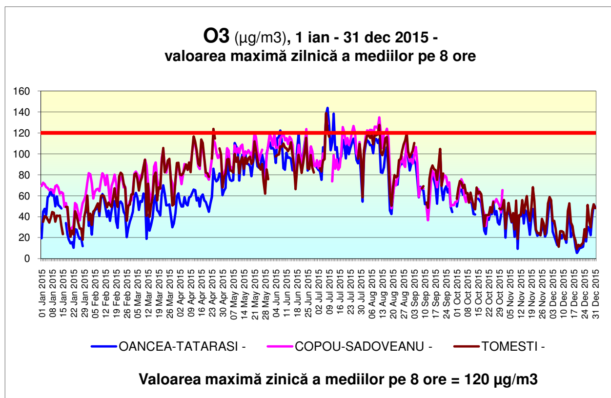
Figura I.3.8.2. Variația valorilor maxime zilnice a mediilor pe 8 ore a concentrației de ozon în anul 2015
