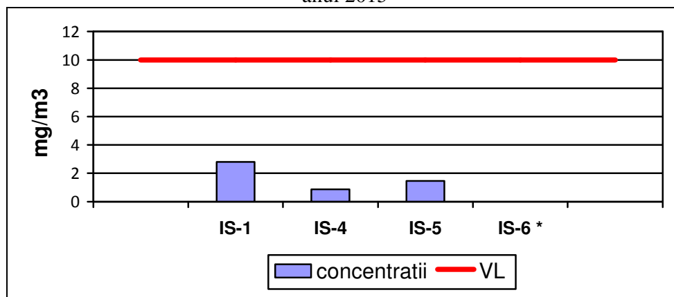
Figura I.3.5.2. CO - Maxima zilnică mediei pe 8 ore, înregistrate la stațiile de monitorizare, în anul 2015
