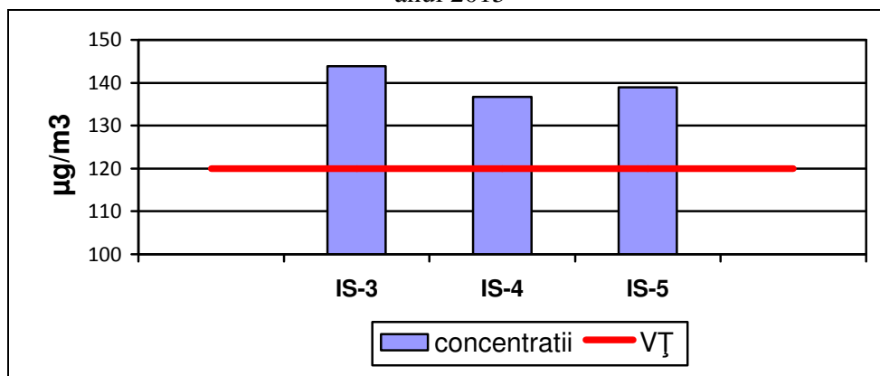
Figura I.3.8.1. Ozon – Maxima zilnică mediei pe 8 ore, înregistrate la stațiile de monitorizare, în anul 2015
