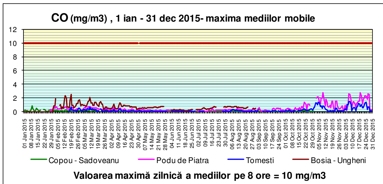
Figura I.3.5.1. Variația valorilor maxime zilnice a mediilor pe 8 ore a concentrației de CO în anul 2015
