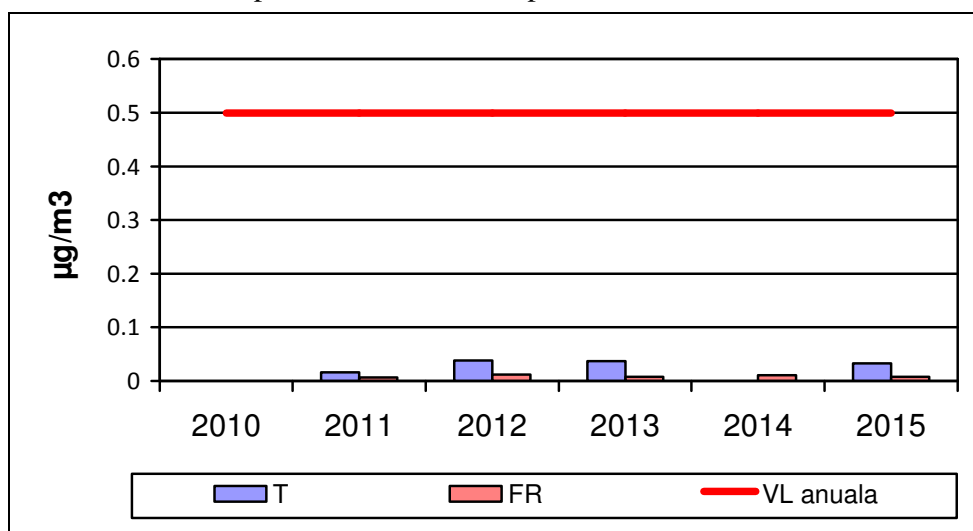
Figura I.I.6. Pb gravimetric determinat din fracția PM 10 – Evoluția concentrațiilor medii anuale înregistrate la stațiile de monitorizare în raport cu VL anuală, în perioada 2010 – 2015
