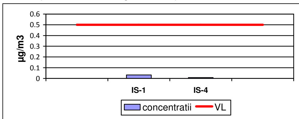
Figura I.3.4.1. Pb gravimetric determinat din fracția PM10 – Concentrațiile medii anuale înregistrate la stațiile de monitorizare, în anul 2015
