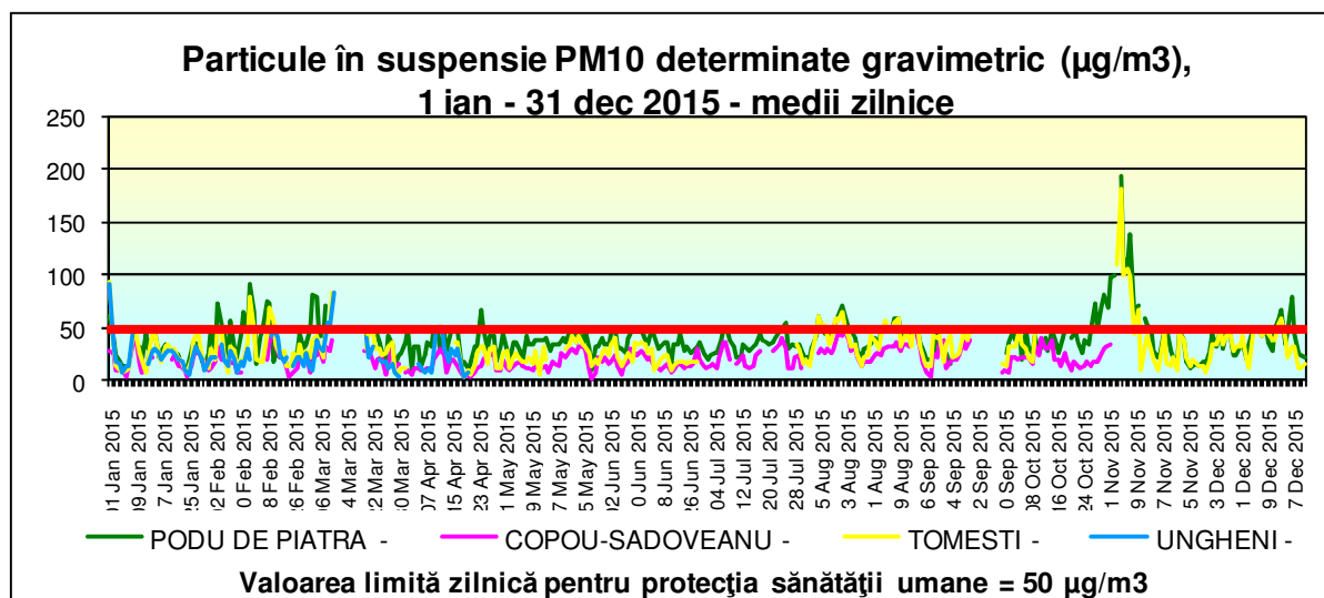
Figura I.3.3.2. Valori medii zilnice particule în suspensie PM10 determinate gravimetric în anul 2015
