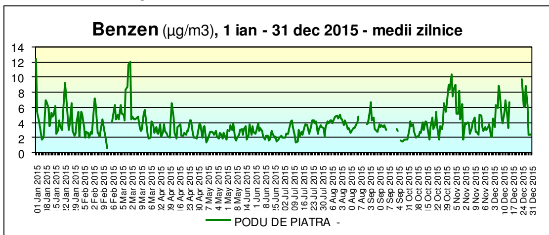
Figura I.3.6.1. Valori medii zilnice ale benzenului
