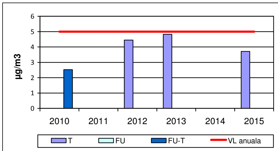
Figura I.I.5. C 6 H 6 – Evoluția concentrațiilor medii anuale înregistrate la stațiile de monitorizare în raport cu VL anuală, în perioada 2010 – 2015
