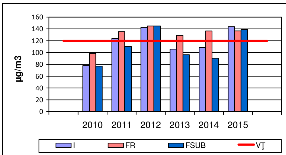
Figura II.4. Ozon – Maxima zilnică mediei pe 8 ore, înregistrate la stațiile de monitorizare în raport cu valoarea țintă, în perioada 2010 – 2015
