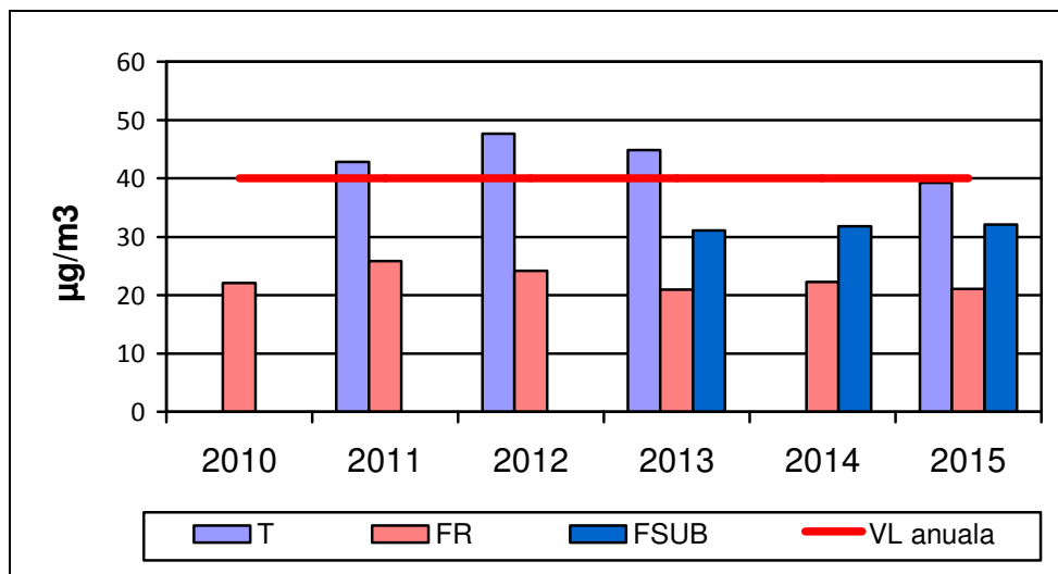
Figura II.3. PM 10 gravimetric – Evoluția concentrațiilor medii anuale înregistrate la stațiile de monitorizare în raport cu VL anuală, în perioada 2010 – 2015
