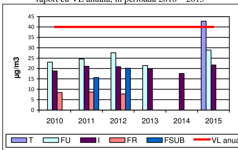
Figura II.1. NO 2 – Evoluția concentrațiilor medii anuale înregistrate la stațiile de monitorizare în raport cu VL anuală, în perioada 2010 – 2015
