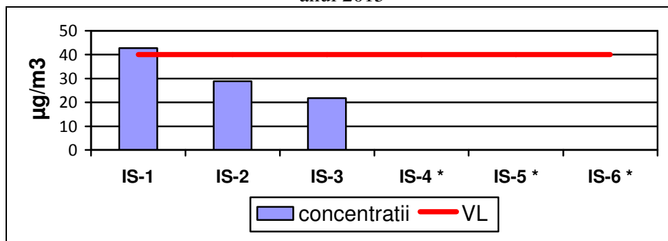
Figura I.3.1.2. \text{NO}_2 - Concentrațiile medii anuale înregistrate la stațiile de monitorizare, în anul 2015
