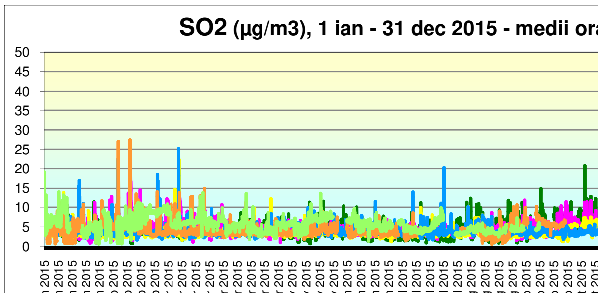
Figura I.3.2.1. Variația mediilor orare a dioxidului de sulf (SO 2 ) în anul 2015
