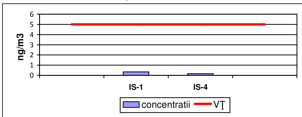
Figura I.3.4.2. Cd gravimetric determinat din fracția PM10 – Concentrațiile medii anuale înregistrate la stațiile de monitorizare, în anul 2015
