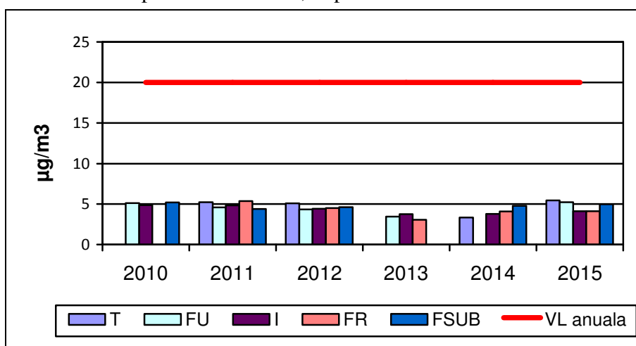
Figura II.2. SO 2 – Evoluția concentrațiilor medii anuale înregistrate la stațiile de monitorizare în raport cu VL anuală, în perioada 2010 – 2015
