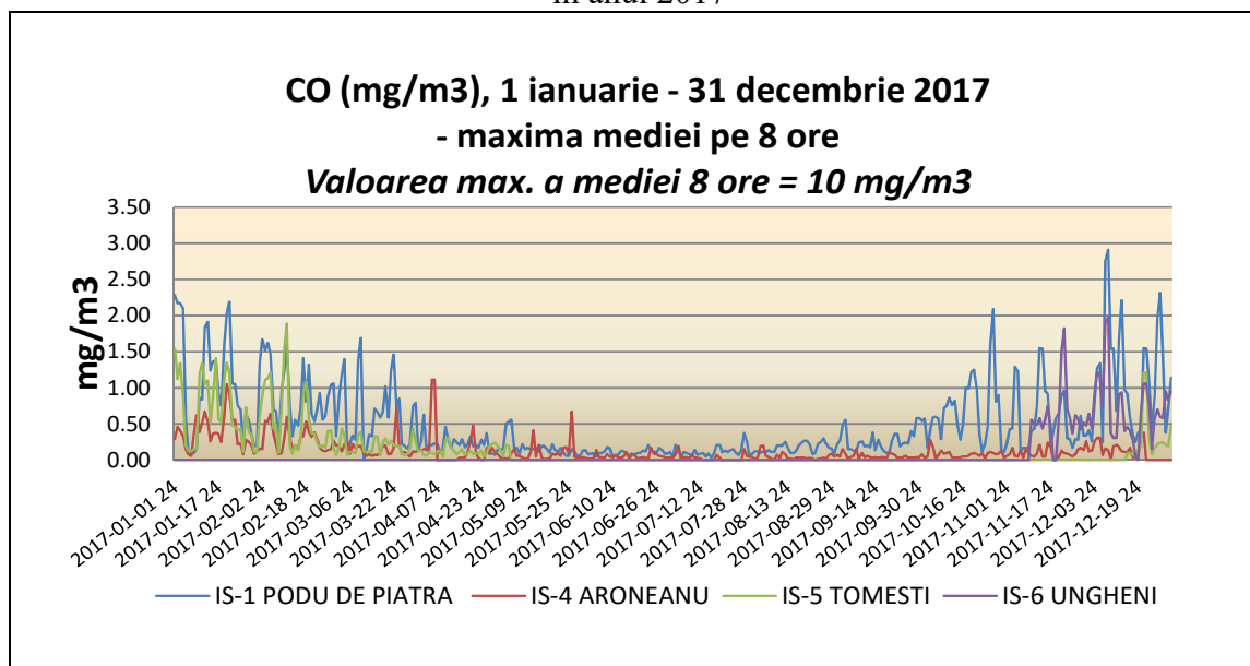
Figura I.3.5.1. Variația valorilor maxime zilnice a mediilor pe 8 ore a concentrației de CO, în anul 2017
