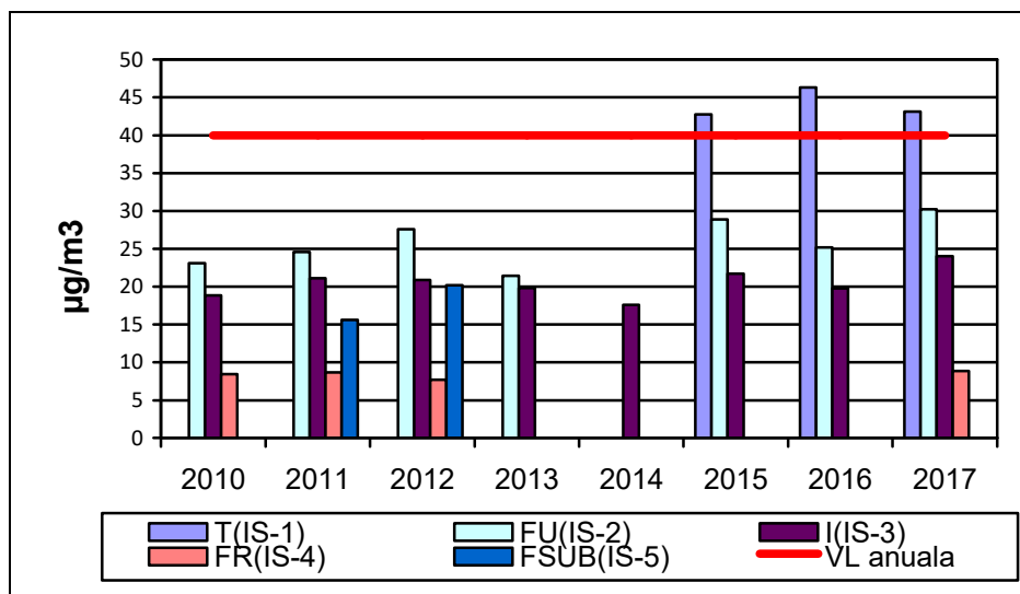
Figura II.1. NO 2 – Evoluția concentrațiilor medii anuale înregistrate la stațiile de monitorizare în raport cu VL anuală, în perioada 2010 – 2017
