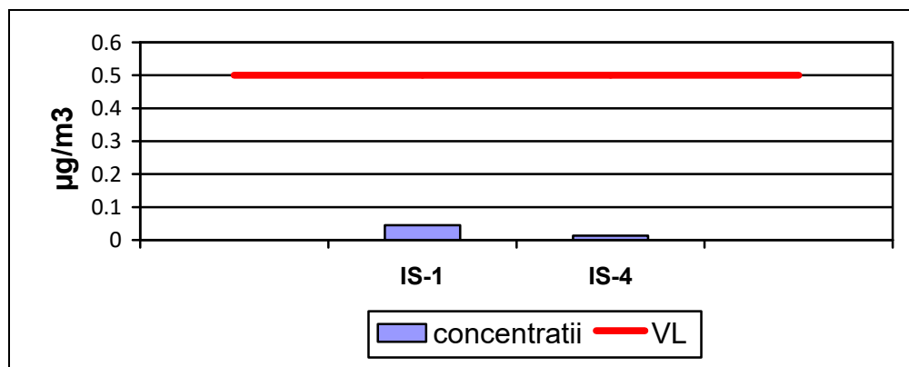
Figura I.3.4.1. Pb gravimetric determinat din fracția PM10 – Concentrațiile medii anuale înregistrate la stațiile de monitorizare, în anul 2017
