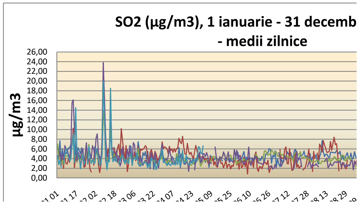
Figura I.3.2.2. Variația mediilor zilnice a dioxidului de sulf (SO 2 ) în anul 2017
