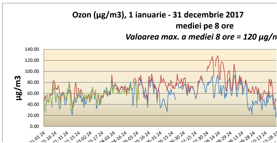
Figura I.3.8.2. Variația valorilor maxime zilnice a mediilor pe 8 ore a concentrației de ozon în anul 2017
