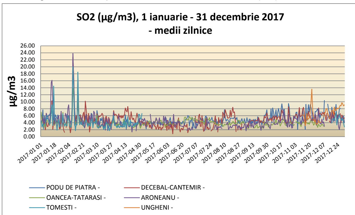
Figura I.3.2.2. Variația mediilor zilnice a dioxidului de sulf (SO 2 ) în anul 2017
