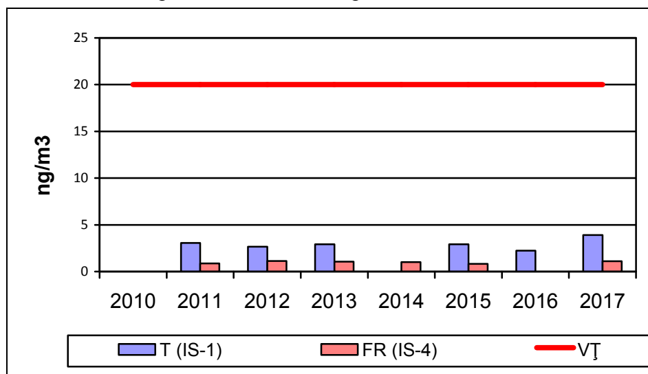
Figura I.I.8. Ni gravimetric determinat din fracția PM10 – Evoluția concentrațiilor medii anuale înregistrate la stațiile de monitorizare în raport cu VL anuală, în perioada 2010 – 2017
