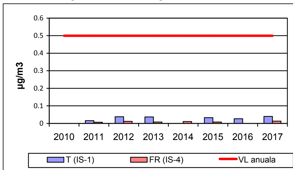
Figura I.I.6. Pb gravimetric determinat din fracția PM10 – Evoluția concentrațiilor medii anuale înregistrate la stațiile de monitorizare în raport cu VL anuală, în perioada 2010 – 2017
