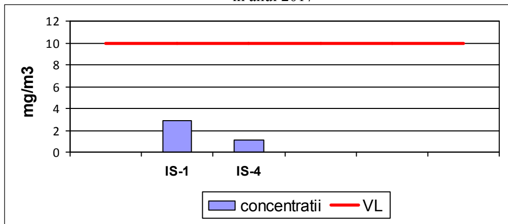
Figura I.3.5.2. CO - Maxima zilnică mediei pe 8 ore, înregistrate la stațiile de monitorizare, în anul 2017
