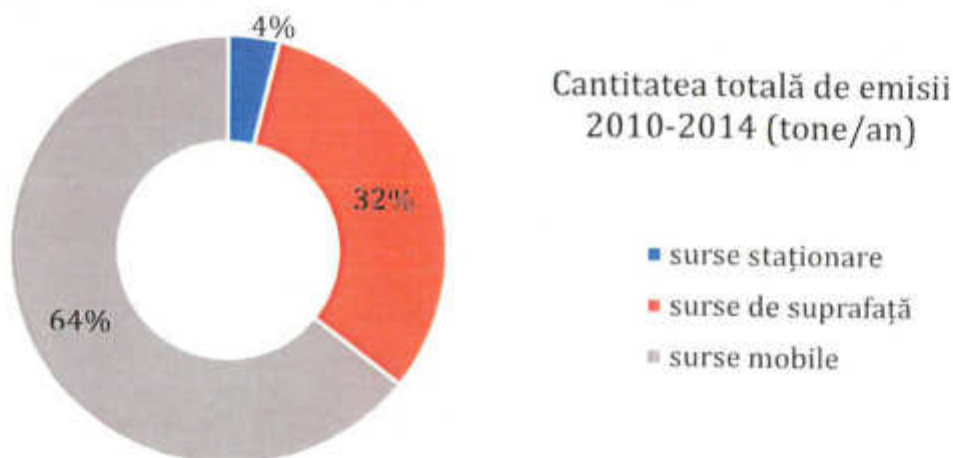
Figura nr. 5-1 – Contribuția surselor de emisii de particule în suspensie (PM 10 ), în perioada 2010-2014 pentru Aglomerarea Iași
