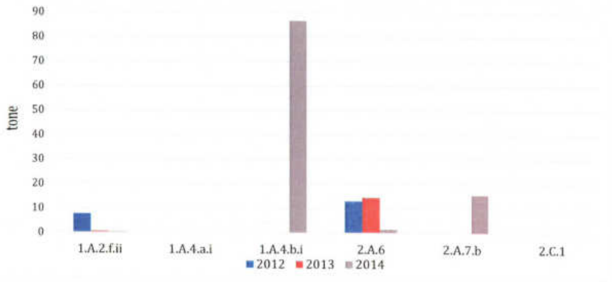
Figura nr. 5-21 - Repartizarea surselor de suprafață a PM 10 (ILE 2014) la nivelul Aglomerării Iași
