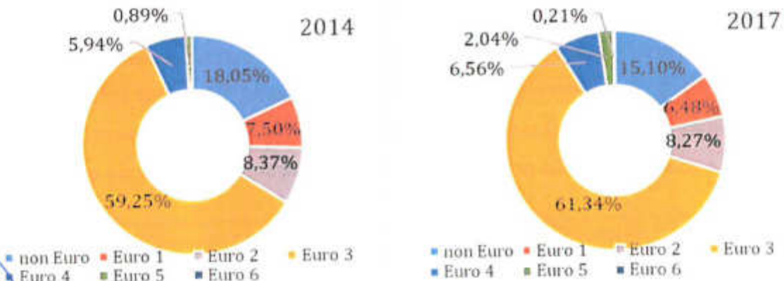
Figura nr. 5-12 - Distribuția emisiilor de PM 10 în funcție de tehnologia autoturismelor ce utilizează motorină în anul 2017 comparativ cu anul 2014
