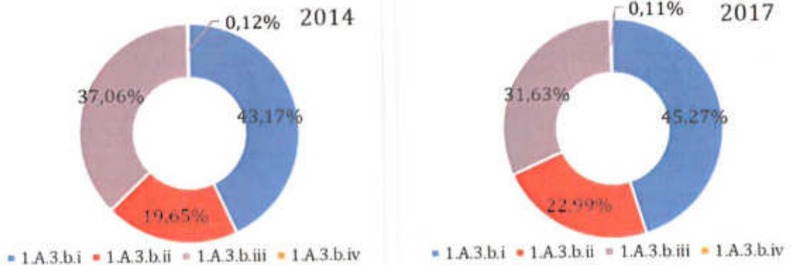
Figura nr. 5-10 - Distribuția emisiilor de PM 10 pe tipuri principale de vehicule în anul 2017 comparativ cu anul 2014
