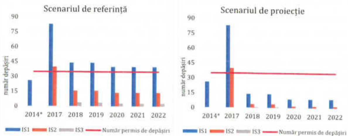
Figura nr. 10-3 – Numărul de depășiri anuale ale valorii limită zilnice pentru PM 10 în urma aplicării scenariilor
