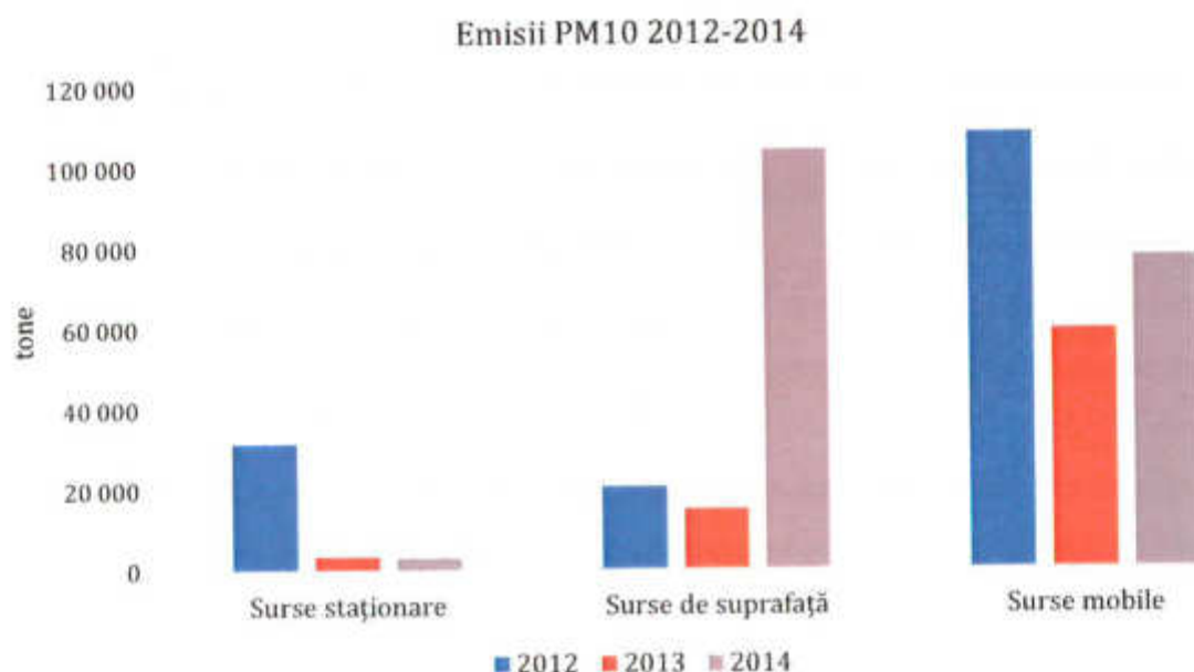
Figura nr. 5-4 - Tendința emisiilor de particule în suspensie (PM 10 ), în perioada 2012-2014 pentru aglomerarea Iași
