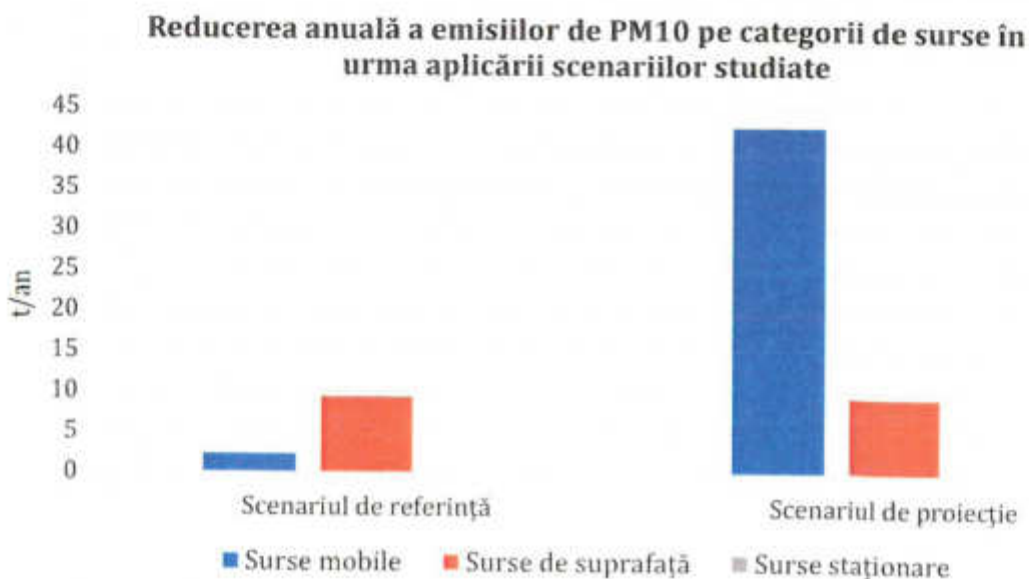
Figura nr. 10-1 - Reducerea emisiilor de PM 10 pe categorii de surse în urma aplicării scenariilor studiate în vederea încadrării sub valoarea limită
