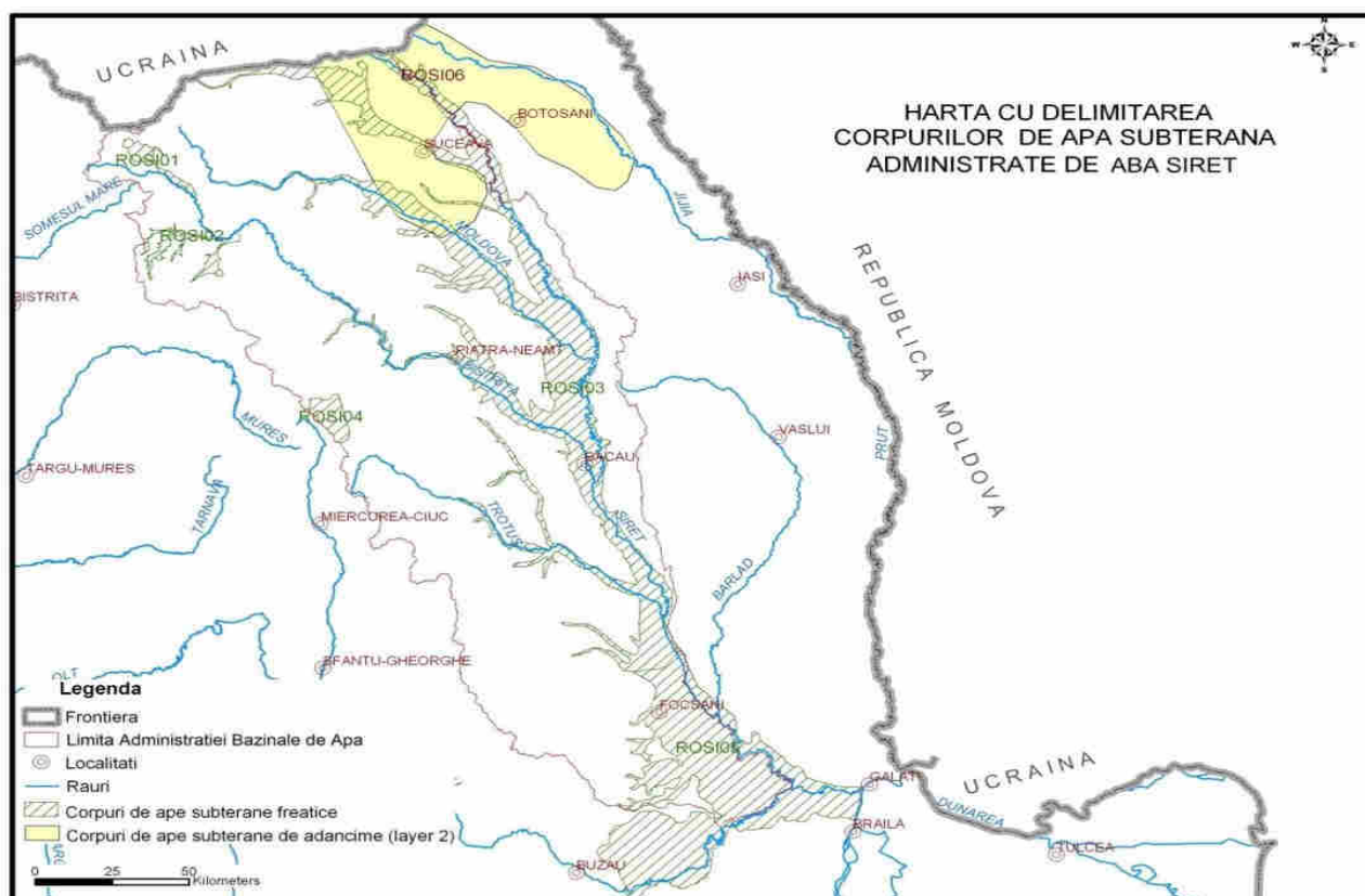
Figura nr. 17. Delimitarea corpurilor de apă subterană atribuite Administrației Bazinale de Apă Siret (Sursa: Planul de management al Spațiului Hidrografic Siret)
